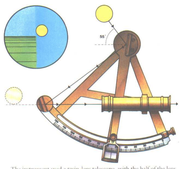
Figura 28.2: O sextante de Hadley. O observador vê a imagem do horizonte e da estrela simultaneamente, como no desenho do círculo superior esquerdo, e a escala graduada mede o ângulo de altura.
