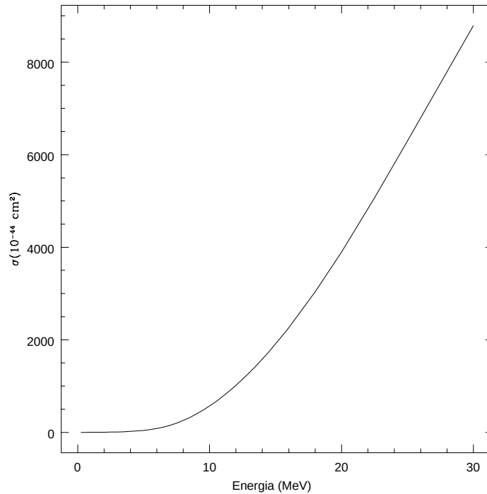
Figura 23.4: Secção de choque dos neutrinos sobre um alvo de gálio, de acordo com John N. Bahcall (1934-2005), publicado em 1997 no Physical Review C , 56, 3391. Existem ressonâncias, como a do neutrino de 15,11 MeV sobre um alvo de ^{12}\text{C} , que leva a uma secção de choque medida de (9,3 \pm 0,6) \times 10^{-42} \text{ cm}^2 .
