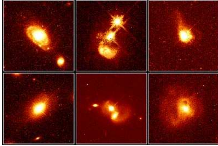
Figura 26.11: Imagens obtidas por John N. Bahcall (1934-2005) e Mike Disney com o Telescópio Espacial Hubble, da NASA, mostrando que os quasares ocorrem tanto em galáxias normais quanto em galáxias perturbadas. Por exemplo, PG 0052+251 (canto esquerdo superior), a 1,4 bilhões de anos-luz da Terra, reside em uma galáxia espiral normal; PHL 909, a 1,5 bilhões de anos-luz (canto inferior esquerdo), em uma galáxia elíptica; IRAS04505-2958, PG 1212+008, Q0316-346 e IRAS13218+0552, em vários tipos de galáxias em interação.
