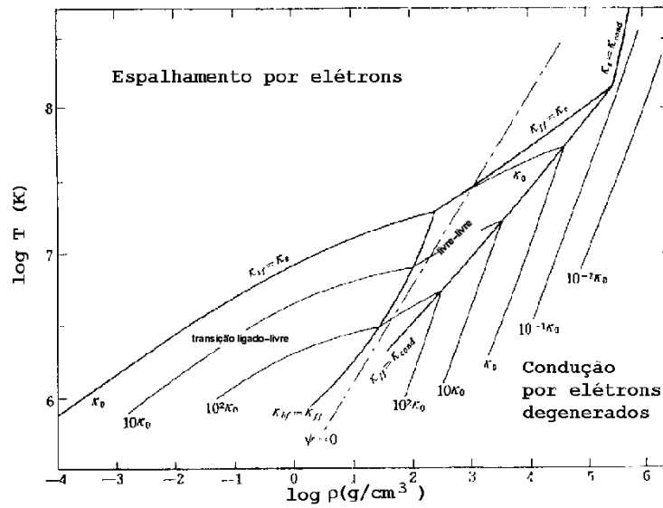
Figura 23.12: Figura publicada por Chushiro Hayashi, Minoru Nishida and Daiichiro Sugimoto (1962, Progress of Theoretical Physics Vol. 27 No. 6 p. 1233) ilustrando as regiões onde cada tipo de opacidade é mais importante, em função da temperatura e densidade.
