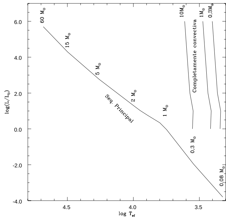
Figura 23.28: Seqüência principal e zona completamente convectiva
