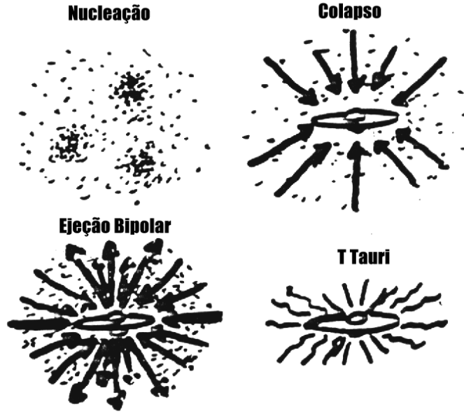
Figura 23.64: Esquema de formação estelar
