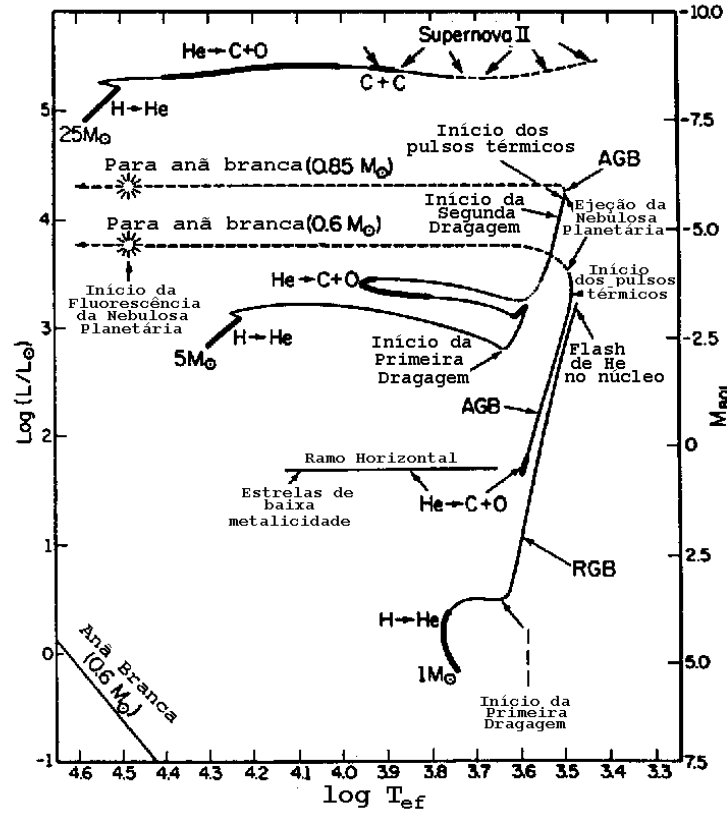
Figura 23.32: Evolução a partir da sequência principal para modelos de 1, 5 e 25 M_{\odot} . A queima de combustível no núcleo ocorre nas regiões mais escuras das curvas. Durante a fase interpulso, o He produzido pela camada termonuclear dominante, de queima de H, é acumulado na camada de He, até que um flash de He ocorra, que induz a uma zona de convecção entre as camadas. A terceira dragagem ocorre durante a fase de pulsos térmicos, e é onde se formam as estrelas carbonadas e estrelas ricas em ZrO. A opacidade das moléculas na atmosfera, que está mudando com a dragagem, bem como o aumento da perda de massa com a metalicidade, precisa ser incluída nos modelos. Nos modelos de Leo Girardi e Paola Marigo, a fase das estrelas carbonadas dura entre 2 e 3 milhões de anos.
