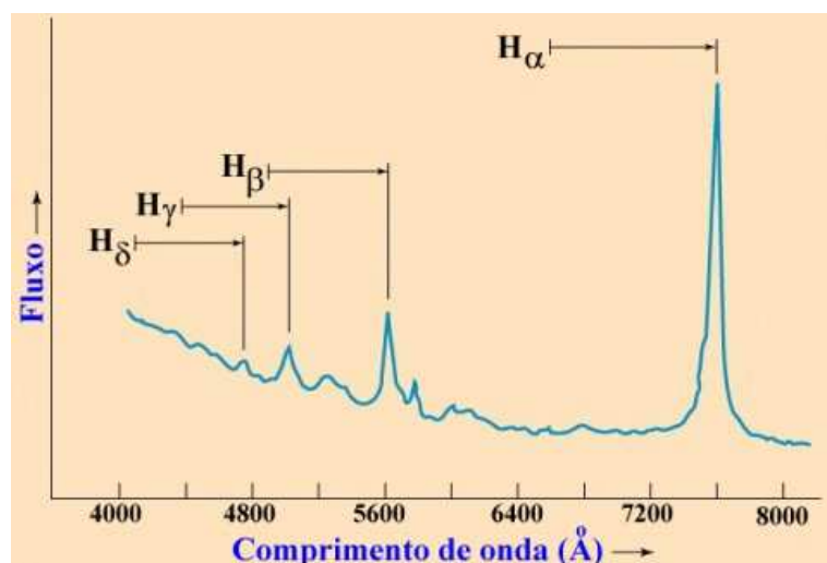
Figura 26.12: O espectro do quasar 3C 273 no ótico e infravermelho próximo é dominado pelas linhas do hidrogênio em emissão e deslocadas para o vermelho ( redshifted ) por efeito Doppler. Por exemplo, a linha H \beta está deslocada de 4861 Å para 5630 Å.
