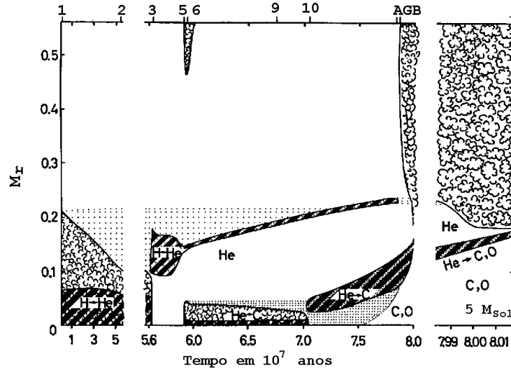
Figura 23.39: Evolução da estrutura interna de uma estrela de 5 M_{\odot} após a seqüência principal. Os números na parte superior da figura correspondem às fases equivalentes da figura na página 430. As regiões escuras indicam queima nuclear, e as com bolhas indicam convecção.
