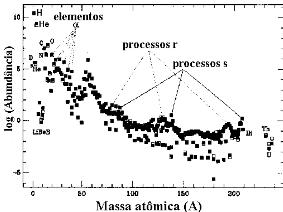
Figura 23.20: Abundâncias solares: os símbolos fechados são de acordo com a compilação de E. Anders & M. Grevesse, 1989, Geochimica et Cosmochimica Acta , 53, 197, e os abertos de Alastair G.W. Cameron (1925-), 1982, Essays in Nuclear Astrophysics , ed. Charles A. Barnes, Donald D. Clayton & David N. Schramm (1945-1997), Cambridge, p. 23. Nota-se claramente que os elementos com números pares de prótons e nêutrons têm maior abundância.
