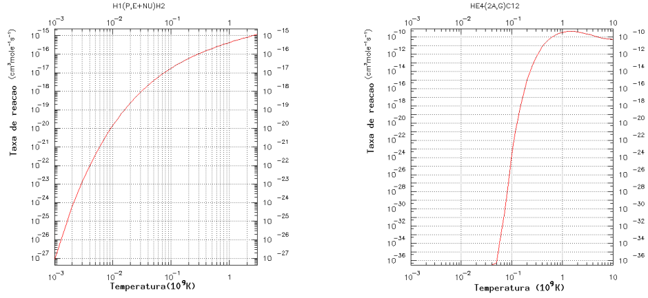
Figura 23.18: Taxa de reação nuclear para p + p \rightarrow D + e + \bar{\nu}_e e 3\text{He}^4 \rightarrow \text{C}^{12} + \gamma .
