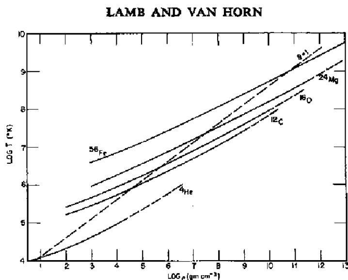
Figura 23.51: Curvas de cristalização para ^4\text{He} , ^{12}\text{C} , ^{16}\text{O} , ^{24}\text{Mg} e ^{56}\text{Fe} calculados por Donald Quincy Lamb & Hugh van Horn (1975) Astrophysical Journal , 200, 306. A curva pontilhada corresponde a divisória entre pressão de um líquido quântico (abaixo da curva) e de um gás ideal (acima da curva), isto é, os efeitos quânticos iônicos são importantes à direita da linha pontilhada. Quando a temperatura efetiva atinge esta curva, por esfriamento, ocorre uma pequena descontinuidade na capacidade térmica dos íons, devido à transição de fase.
