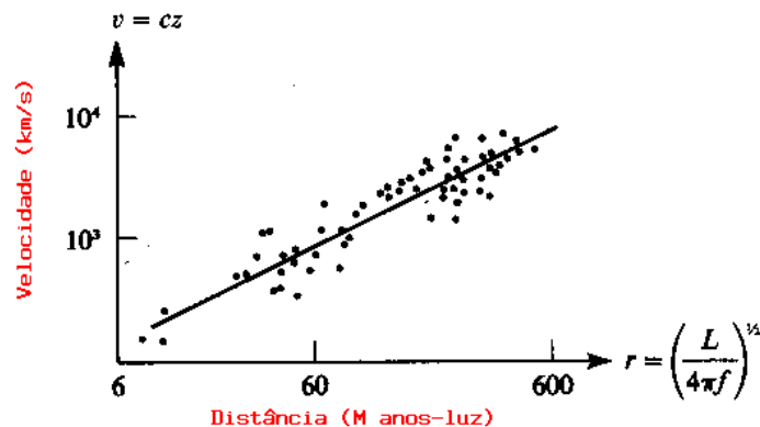
Figura 26.16: Lei de Hubble: a velocidade é proporcional à distância.
