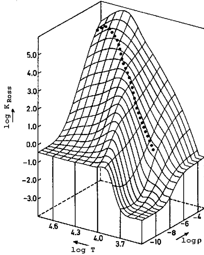
Figura 23.16: Opacidade de Rosseland K_{Ross}(\text{cm}^2/\text{g}) , para valores de \rho ( \text{g}/\text{cm}^3 ) e T(\text{K}) , para uma mistura de hidrogênio e hélio com X=0,739 e Y=0,240 , de acordo com os cálculos de Los Alamos.
