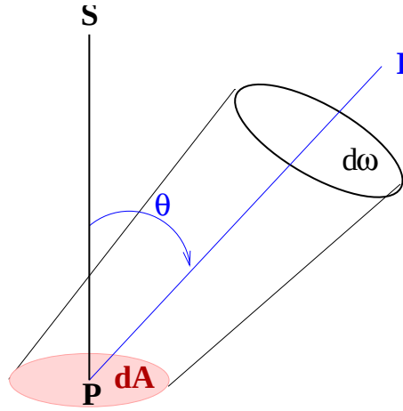
Figura 23.8: Intensidade e ângulo sólido
