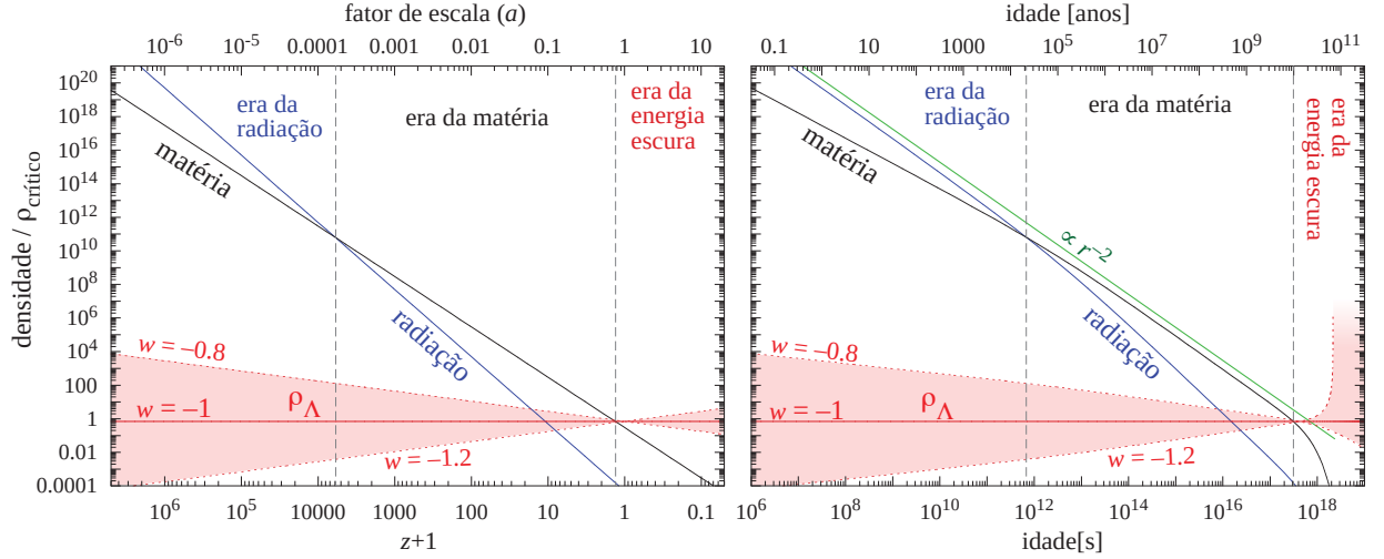
Figura 39: Evolução da densidade da matéria não-relativística (“poeira”), radiação e energia escura (constante cosmológica) em função do fator de escala (esquerda) e da idade do universo normalizada (direita). As intersecções representam os momentos de equipartição de energia. A esquerda também está representada a evolução da energia escura no caso de w = -1 \pm 0,2 , w constante. Para w = -1.2 podemos notar a ocorrência do “Big Rip” por volta de 7 \times 10^{10} anos.
