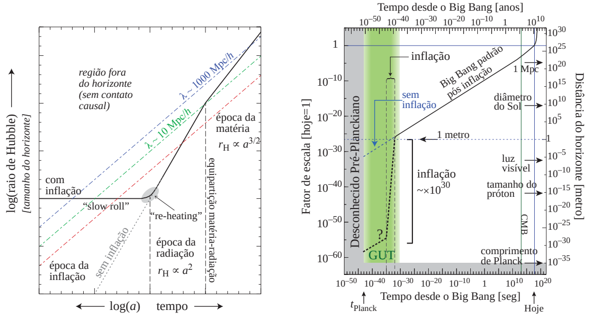
Figura 50: Esquerda: Evolução do tamanho do Universo visível (raio de Hubble) durante e após a inflação (baseado em Martin, 2004 ). A aproximação “slow-roll” significa que o potencial V da inflação é quase-plano ( H(t) é praticamente constante durante a inflação). As linhas diagonais mostram como as regiões do Universo podem entrar ou deixar de estar em contato causal. Com inflação, mesmo as maiores estruturas estiveram em algum momento em contato causal. Direita: Evolução do fator de escala mostrando o efeito da inflação comparado a outros momentos do Universo.
