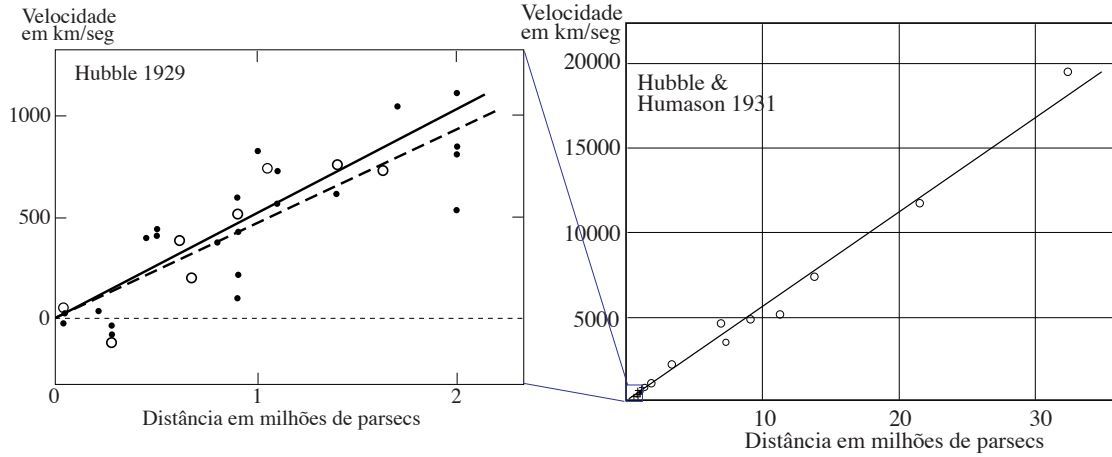
Figura 17: A relação velocidade heliocêntrica–distância. Esquerda: figura 1 de Hubble (1929); as distâncias foram medidas utilizando Cefeidas (cada círculo representa uma galáxia). Direita: figura 5 de Hubble & Humason (1931); os círculos representam valores médios de aglomerados (as distâncias são obtidas através da distribuição de magnitudes aparentes dos membros dos aglomerados).
