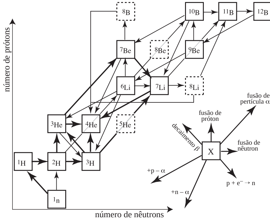
Figura 52: Cadeia de reações que ocorrem na nucleossíntese primordial. Os núcleos pontilhados são instáveis. Os núcleos ^3\text{H} e ^7\text{Be} são radiativos, mas com meia vida superior à duração da nucleossíntese primordial (12,33 anos e 53,29 dias, respectivamente).
