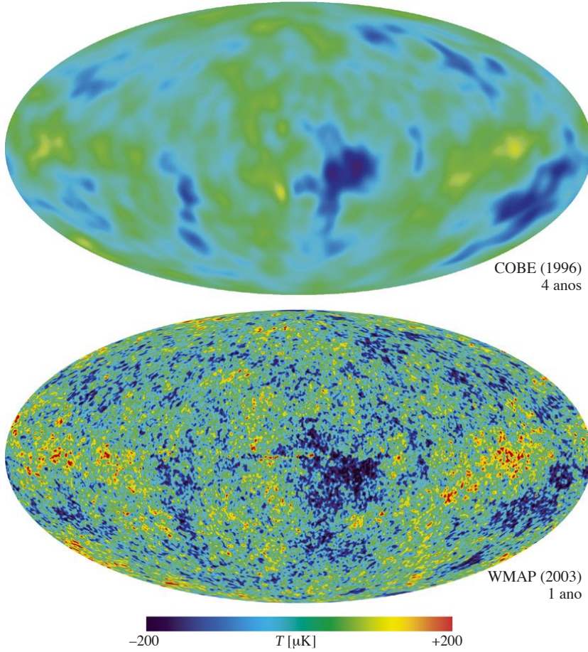
Figura 23: Imagem da CMB obtida pelo satélite WMAP (abaixo), comparada com a obtida pelo COBE (acima), onde a temperatura média, dipolo cinemático e a Via Láctea foram subtraídos. As flutuações de temperatura são da ordem de \Delta T/T \approx 10^{-5} . Compare a resolução do WMAP e COBE. Figura tirada do site do WMAP e Bennett et al. (2003).
