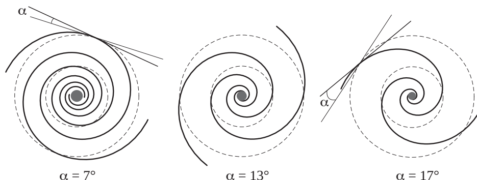
Figura 249: Ângulo de abertura de braços espirais ( pitch angle , \alpha ) medido entre as tangentes do braço e de um círculo concêntrico à galáxia.
