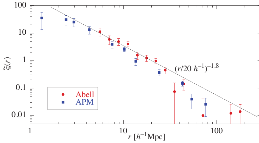
Figura 99: Função de correlação de aglomerados de galáxias selecionados no ótico (351 aglomerados do catálogo de Abell e 364 do APM Postman, 1998).
