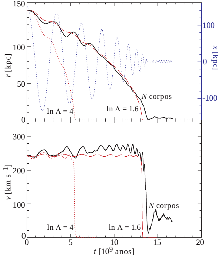
Figura 193: Fricção dinâmica agindo sobre uma galáxia satélite de 10^7 M_\odot orbitando um halo isotérmico; acima posição, abaixo velocidade da satélite. Comparação do efeito obtido em uma simulação de N -corpos (traço contínuo) com a aproximação de Chandrasekhar (traços pontilhados e tracejados). Figura tirada de Fellhauer et al. (2000) .
