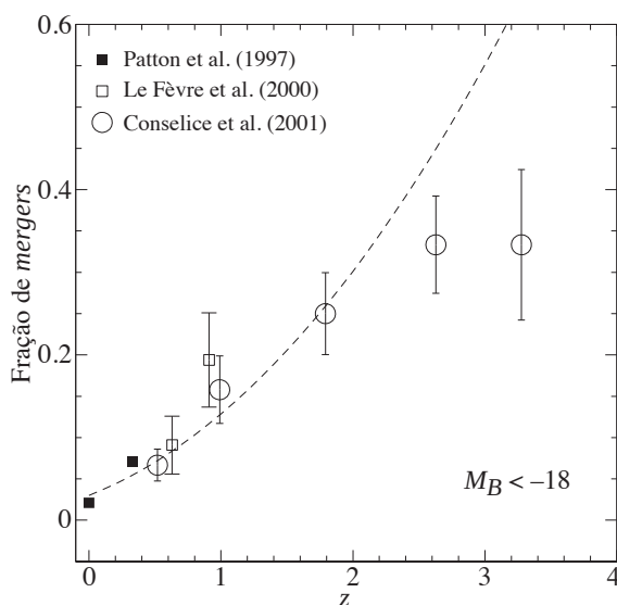
Figura 239: Taxa de merger estimado por distorções e frequência de pares de galáxias. A curva tracejada corresponde a uma taxa de merger de f = 0,03(1+z)^{2,1} . (Conselice, 2000).
