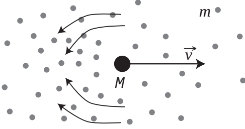
Figura 192: Ilustração do fenômeno da fricção dinâmica: um corpo de massa \mathcal{M} se desloca com velocidade \vec{v} em um meio de densidade local \rho , dispersão de velocidades \sigma , composto de partículas de massa m ( \mathcal{M} \gg m ).
