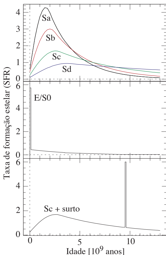
Figura 197: Exemplos de possíveis taxas de formação estelar (unidades arbitrárias) para diferentes tipos morfológicos de galáxias. Para galáxias espirais a taxa de formação estelar (sem surtos) diminui aproximadamente de forma exponencial. Figura baseada em Pogianti et al. (1999) .
