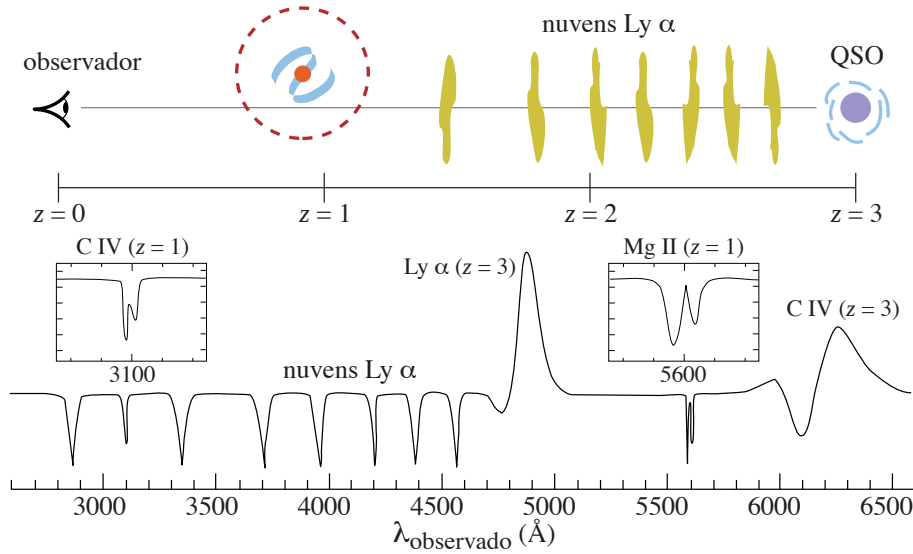
Figura 223: Representação esquemática da formação da floresta Ly \alpha . Nuvens de HI entre o observador e o QSO produzem linhas que são observadas com \lambda_{\text{obs}} = 1215,67 \text{ \AA} (1 + z_{\text{abs}}) , onde z_{\text{abs}} é o redshift da nuvem.
