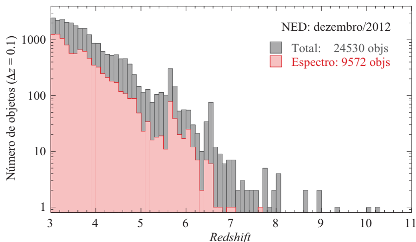
Figura 204: Distribuição em redshift dos objetos com z \geq 3 . Destacado em vermelho estão os objetos com confirmação espectroscópica; a maioria dos redshifts são estimados fotometricamente (“ redshift fotométrico”) ou com apenas uma linha (Ly \alpha 1216Å). Fonte: NED.
