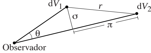
Figura 103: Definição da função de correlação de duas variáveis. As “distâncias” r e \pi entre os volumes dV_1 e dV_2 são medidas no espaço de velocidades ( redshift ).
