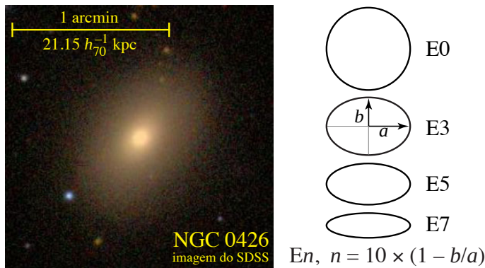
Figura 248: Classificação de galáxias Elípticas segundo o grau de achatamento aparente. a e b são os semi-eixos maior e menor, respectivamente.
