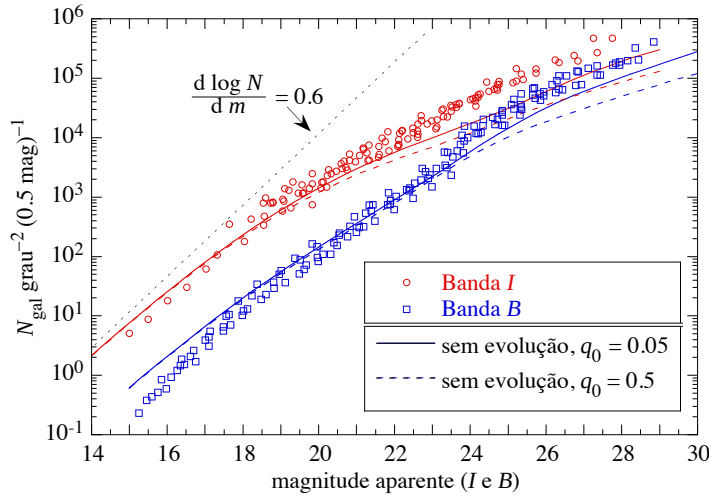
Figura 36: Contagem de galáxias nas bandas I e B . As linhas contínuas e tracejadas correspondem às previsões de contagens para dois modelos de Universo. A reta pontilhada corresponde a um Universo Euclidiano estático. Dados compilados por Metcalfe (2001).
