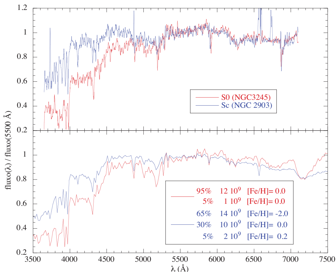
Figura 256: Espectros de galáxia S0 e Sc (acima) e espectros sintéticos (abaixo).
