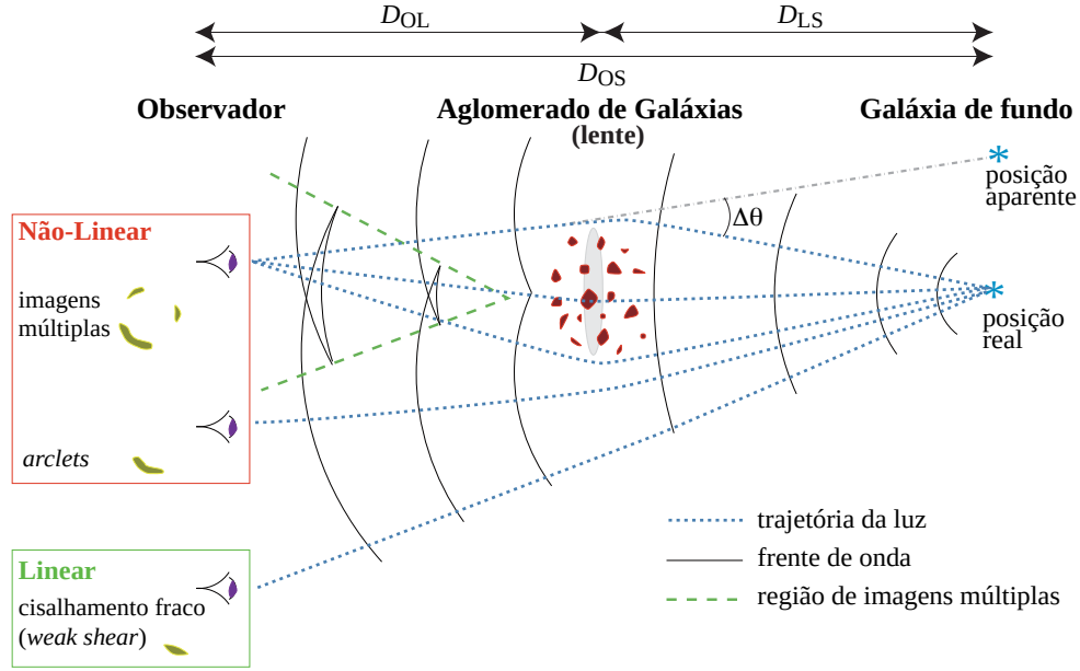
Figura 132: Diagrama mostrando a geometria de lentes gravitacionais produzidas por um aglomerado de galáxias. As distâncias aqui são angulares (cf. seção 2.7.2). No caso de lentes fortes, os arcos formados estarão aproximadamente em \theta_E e a densidade superficial da lente é maior que \Sigma_{\text{crit}} . Figura tirada de Kneib & Ellis (1996).
