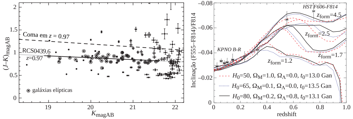
Figura 144: Esquerda: Sequência Vermelha para um aglomerado distante em z \approx 1 comparada à Sequência Vermelha do aglomerado de Coma, se este estivesse em z \approx 1 , mas ignorando a evolução passiva da Pop. estelar. Note o deslocamento para o azul em z = 1 e a pequena mudança da inclinação. Figura tirada de Barrientos et al. (2004) . Direita: Comparação da evolução da inclinação da Sequência Vermelha com o redshift para diversos modelos cosmológicos e diferentes épocas de formação das galáxias elípticas. Figura tirada de Gladders et al. (1998) .
