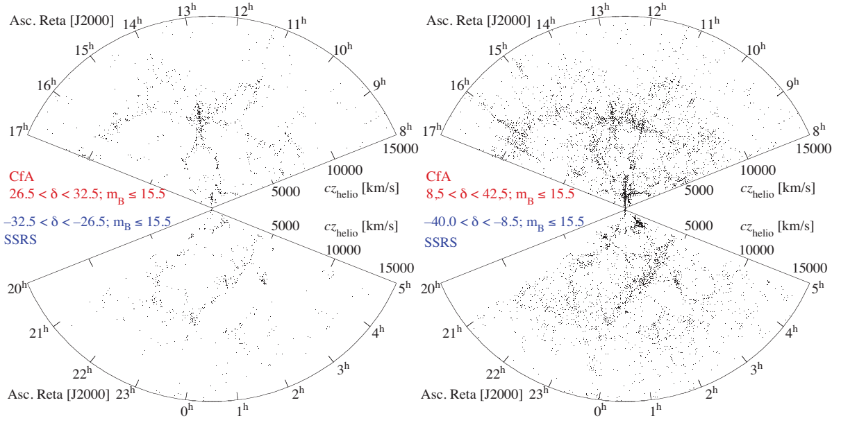
Figura 91: Distribuição de galáxias com m_B \leq 15.5 do survey do CfA (de Lapparent, Geller & Huchra, 1986) no Norte e do SSRS ( South Sky Redshift Survey , da Costa et al., 1988), no Sul. Esquerda: a fatia de declinação é de 26,5 < |\delta| < 32,5 ; Direita: a fatia é maior, de 8,5 < |\delta| < 42,5 ( -40^\circ no Sul). No Norte, a estrutura central é o aglomerado de Coma. A estrutura perpendicular a Coma é chamada ‘Grande Muro’ ( CfA Great Wall ). No Sul, vemos um vazio ( \sim 23^h e 5000 km/s) e o Grande Muro do Sul. Note como os aglomerados ricos aparecem como “dedos de deus”.
