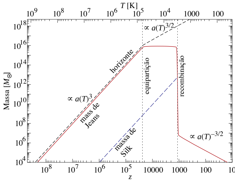
Figura 70: Massa de Jeans em função do redshift (e temperatura) para matéria bariônica. Também estão representadas a massa no interior do horizonte ( r_H \approx cH_0^{-1} ) e o limite de massa de Silk, que sobrevive ao “Silk damping”
