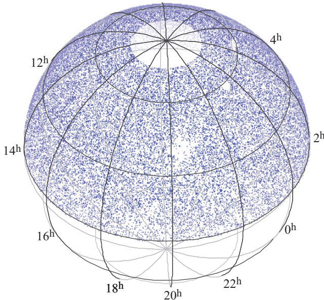
Figura 16: Distribuição em coordenadas equatoriais de fontes discretas em rádio (4,85 GHz [6 cm], fluxo entre 20 e 50 mJy) detectadas no hemisfério norte ( 0^\circ \leq \delta \leq 75^\circ ). Dados de Gregory et al. (1996)
