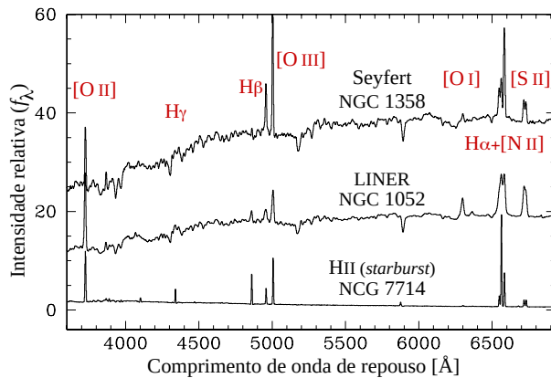
Figura 213: Comparação do espectro ótico de 3 galáxias próximas, 2 AGNs (Seyfert e LINER) e uma com alta taxa de formação estelar e sem núcleo ativo. Figura tirada de Ho (2008).
