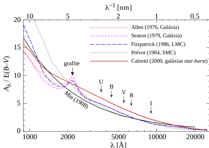
Figura 207: Curvas de extinção da Via Láctea, Nuvens de Magalhães e galáxias com alta atividade de formação estelar. Para comparação, é mostrado a curva correspondente ao modelo de espalhamento de Mie ( \propto \lambda^{-1} ). A escala no alto é usada historicamente neste tipo de diagrama. Algumas bandas espectrais no visível, UV e IV estão indicadas por flechas.
