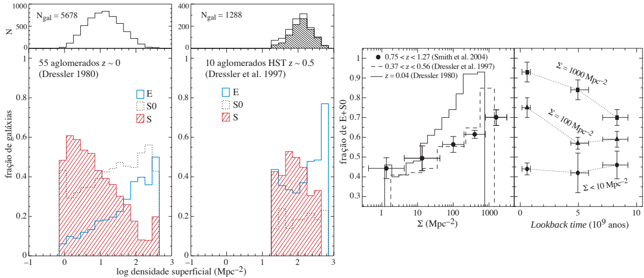
Figura 142: Relação entre o tipo morfológico e a densidade local para galáxias em aglomerados. O histograma no alto de cada painel mostra o número de galáxias para cada intervalo de densidade superficial. Para os aglomerados do HST ( 0.36 < z < 0.57 ), o histograma hachurado do alto dá a distribuição de galáxias após correção da contaminação de galáxias na linha de visada. Os dois gráficos à direita são de Smith et al. (2005) com dados adicionais até z \approx 1 .
