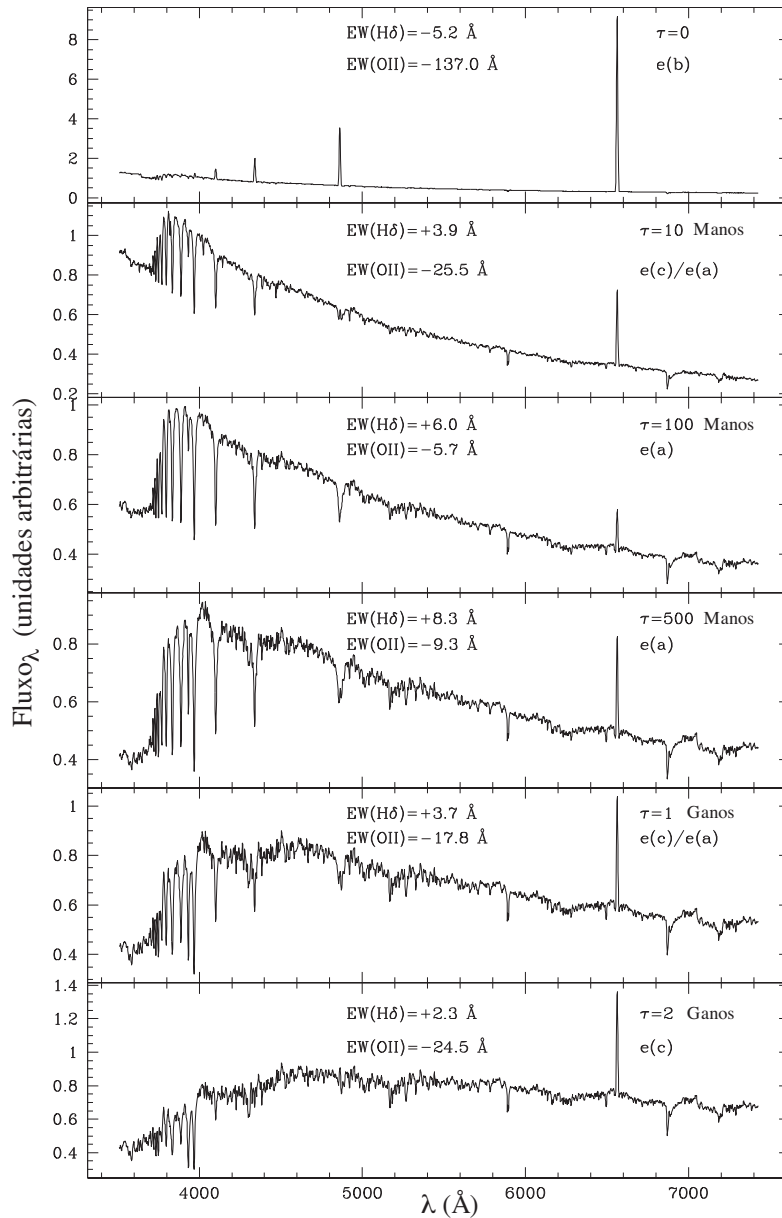
Figura 240: Evolução de um espectro de uma galáxia onde ocorre um starburst (cerca de 35% da massa) durante 100 \times 10^8 anos seguido de uma formação estelar típica de uma Sc. O tempo decorrido após o final do starburst é dado por \tau . Esta galáxia seria classificada de modo diferente segundo o momento em que é observada. Figura tirada de Poggianti et al. (1999).
