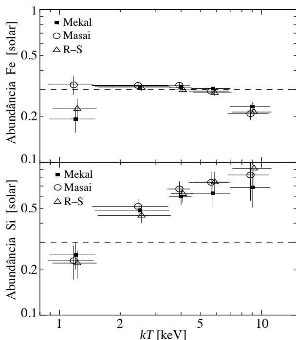
Figura 152: Abundância de ferro e silício em função da temperatura do aglomerado (excluindo a região central) obtidas com satélite ASCA. Enquanto que a abundância de Fe é praticamente independente da temperatura, o Si apresenta uma forte correlação, sendo mais abundante em aglomerados mais quentes (logo, mais maciços). Cada símbolo representa um modelo de plasma diferente. Figura adaptada de Fukazawa et al. (1998) .
