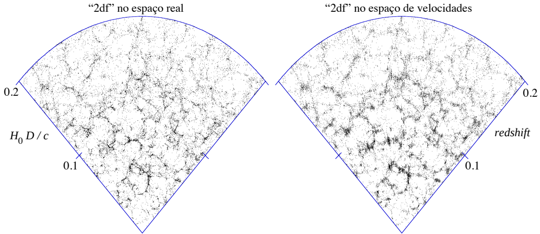
Figura 95: Comparação entre a distribuição de “galáxias” no espaço real e de velocidades em um cenário \Lambda CDM. Os pontos desta figura foram tirados de uma simulação cosmológica de N -corpos de forma a reproduzir o survey 2dF. As figuras são tiradas de Cole et al. (1998) .
