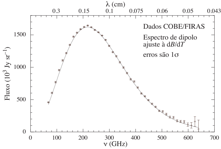
Figura 22: Espectro de dipolo cinemático da radiação cósmica de fundo ajustado aos dados COBE/FIRAS (Fixsen et al., 1996).
