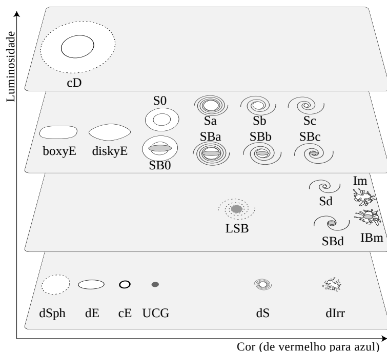
Figura 250: Classificação morfológica incluindo galáxias supergigantes (cD), anãs e de baixo brilho superficial. Para as elípticas normais é adotada a sugestão de Kormendy e Bender de usar a característica boxy/disky das isofotas ao invés do achatamento aparente. Uma classificação em volume semelhante a esta foi proposto por van den Bergh (1997) .
