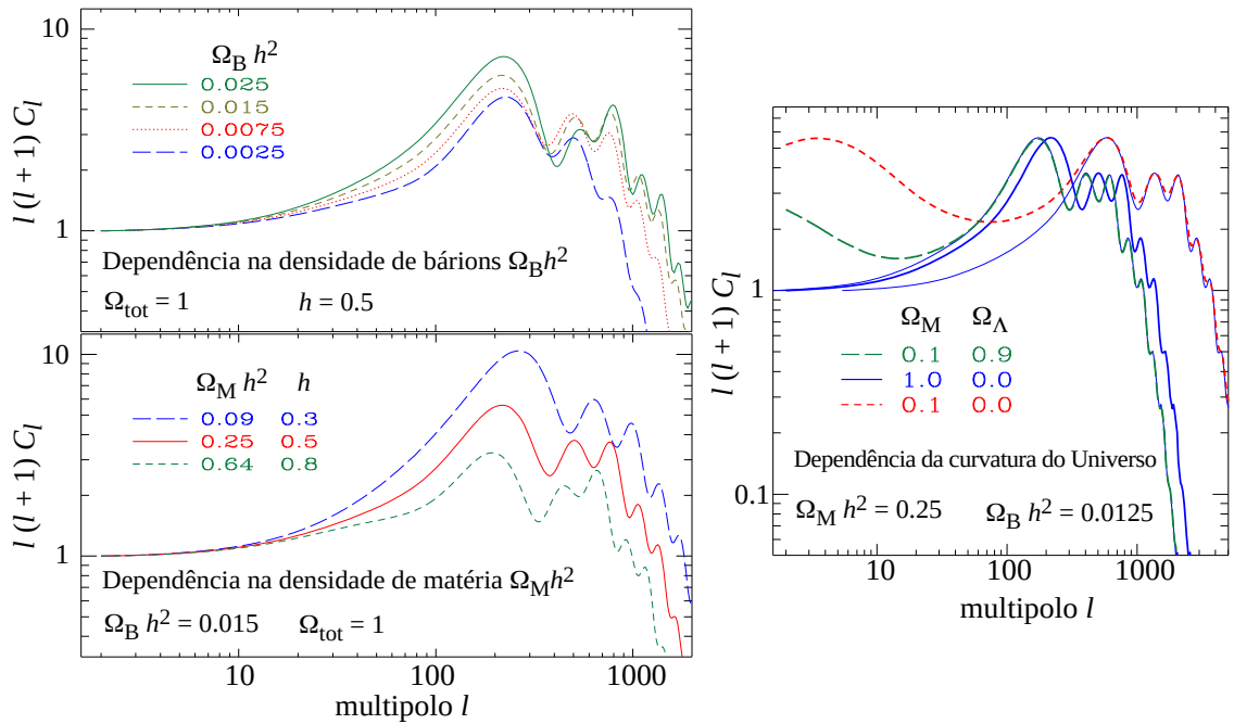
Figura 61: Dependência do espectro de potência com alguns parâmetros cosmológicos. Figura baseada nas animações de Wayne Hu, http://background.uchicago.edu/~whu/ .
