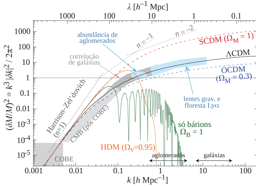
Figura 76: Espectros de flutuações de densidade para 5 cenários cosmológicos diferentes (SCDM = Standard Cold Dark Matter , Universo plano dominado por matéria escura fria; OCDM = Open Cold Dark Matter ; HDM = Hot Dark Matter , neutrino maciço; \Lambda CDM = universo plano dominado pela “energia escura”), e universo apenas com bárions. No eixo superior, \lambda = 2\pi/k é o tamanho linear característico da flutuação de densidade hoje. As linhas pontilhadas indicam a inclinação do espectro de potência, em particular o espectro inicial de Harrison–Zel’dovich com n = -1 . Foram utilizados \Omega_B = 0,046 (exceto no universo bariônico onde \Omega_B = 1 e h = 0,5 (exceto no modelo \Lambda CDM, onde h = 0,7 ). As áreas cinzas correspondem às diversas técnicas observacionais e suas respectivas escalas. As curvas foram calculadas usando o programa camb de A. Lewis, http://camb.info .
