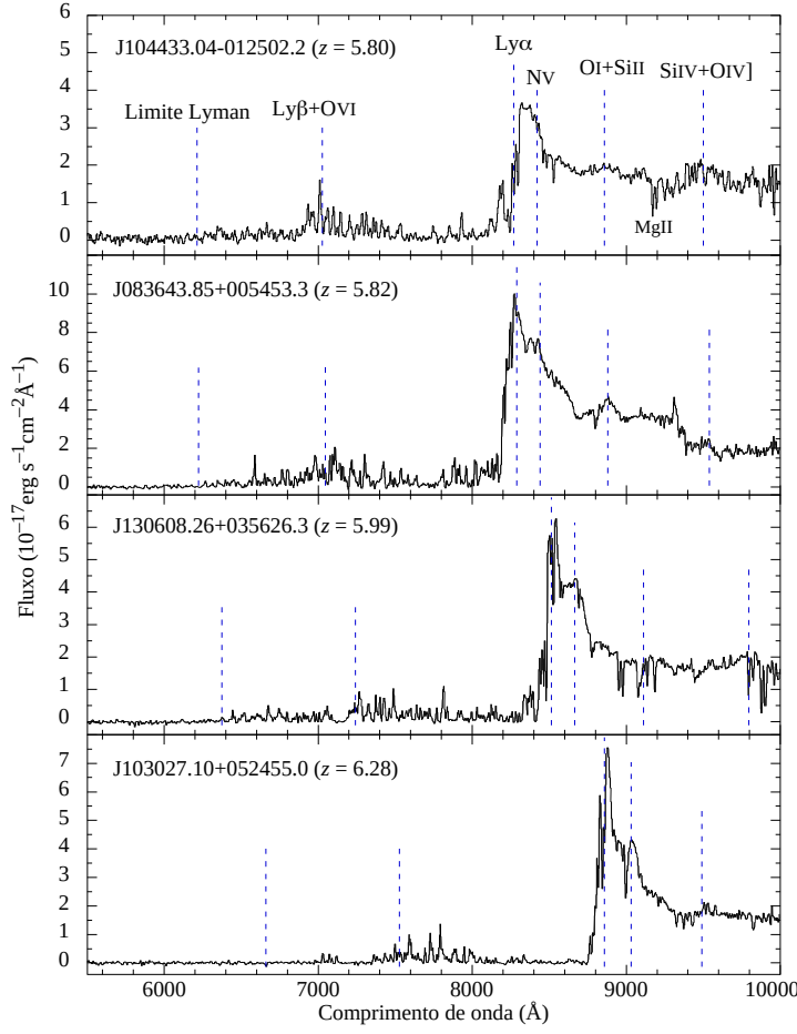
Figura 218: Exemplos de QSOs de alto redshift detectados através do SDSS (Becker et al., 2001). O pico mais importante em emissão corresponde à linha Ly \alpha (1216 Å). Note a diminuição do fluxo logo a esquerda (lado mais vermelho) da linha Ly \alpha ; esta diminuição é devido ao efeito Gunn-Peterson (mais sobre isto na Sec. 12)
