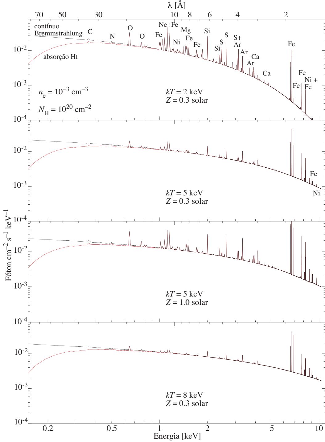
Figura 121: Emissão de um plasma isotérmico (modelo de Raymond-Smith) emitida por um aglomerado e observada após absorção pelo meio interestelar (ISM) para várias temperaturas (em keV) e metalicidades (em unidades de metalicidade solar).
