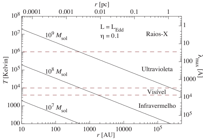
Figura 232: Temperatura do disco de acreção para diferentes massas do buraco negro central. O comprimento de onda onde a emissão de corpo negro é máxima é \lambda_{\max} = (2,9 \times 10^7 / T) \text{ \AA} .
