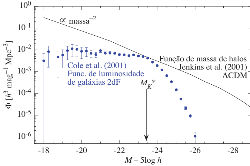
Figura 188: Comparação entre a função de luminosidade na banda K obtida pelo 2dF (Cole et al., 2001) e a função de massa de halos de simulações no cenário \Lambda CDM (Jenkins et al., 2001). A função de massa foi transformada em função de luminosidade utilizando uma razão massa/luminosidade constante. É notável o excesso predito de galáxias de baixa e alta luminosidade.
