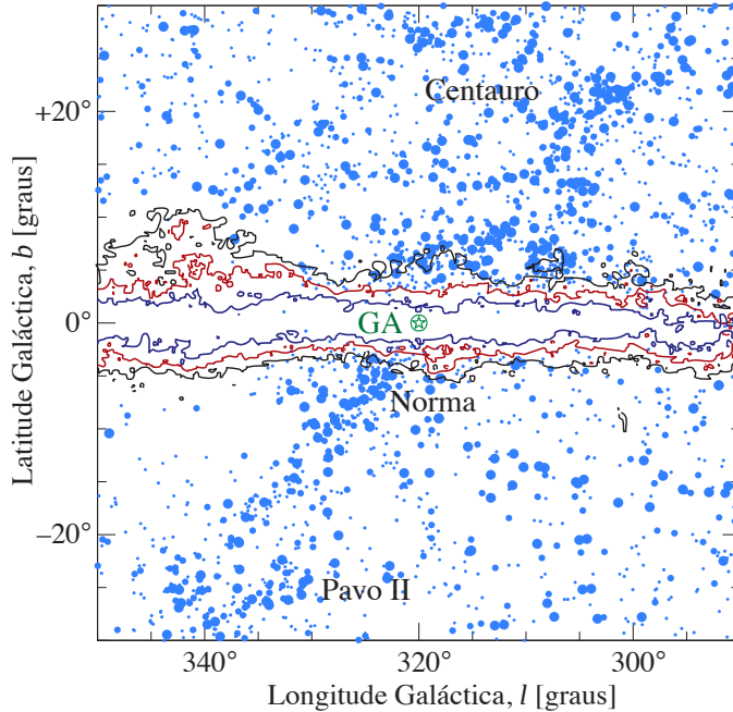
Figura 107: Distribuição de galáxias com diâmetro aparente corrigido da absorção superior a 1,3 na região do Grande Atrator (GA). Os contornos correspondem à absorção galáctica de A_B = 3.0, 5.0 e 10 magnitudes. Figura tirada de Woudt & Kraan-Korteweg (2000).
