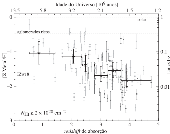
Figura 225: Evolução da metalicidade em sistemas Lyman- \alpha saturados (DLA). A escala de tempo é válida para um Universo \Lambda CDM. Os pontos escuros são as médias em diferentes intervalos de redshift . Figura tirada de Prochaska et al. (2003).
