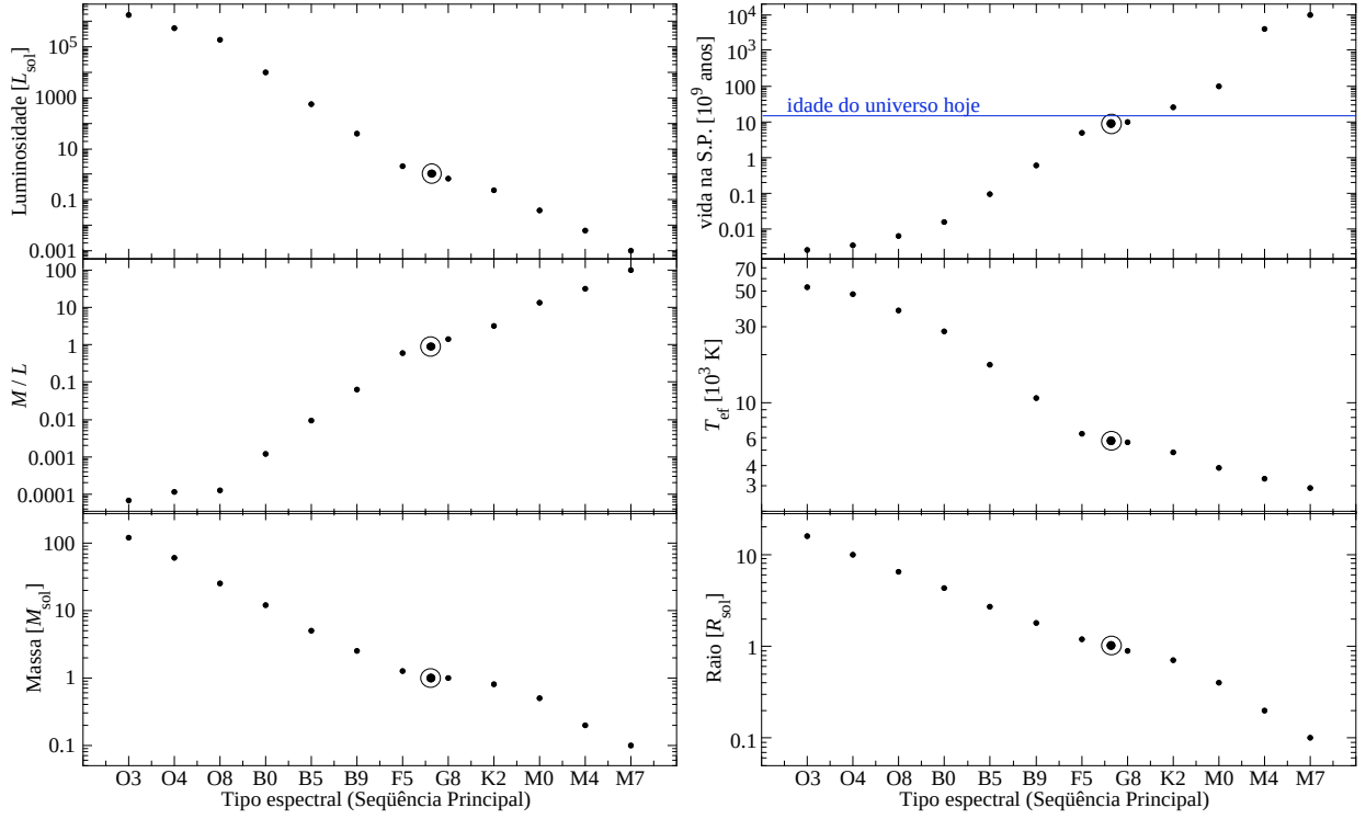
Figura 198: Propriedades físicas das estrelas da Sequência Principal. O Sol está indicado com o símbolo \odot .
