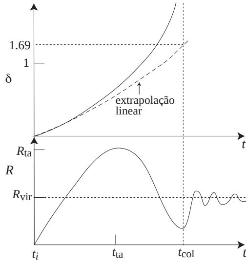
Figura 83: Evolução de uma esfera homogênea. No início o contraste de densidade evolui como previsto pela teoria linear. Eventualmente, a esfera termina sua expansão (o momento do “turn-around”, t_{ta} ) e colapsa. Seu raio final de equilíbrio será aproximadamente metade do raio de turn-around, o raio do virial, R_{vir} . Sua densidade média será \sim 200\rho(t_{col}) . Claramente a aproximação linear não é adequada para modelar o colapso esférico; a discussão detalhada da evolução não linear da formação de estruturas está no capítulo 8.
