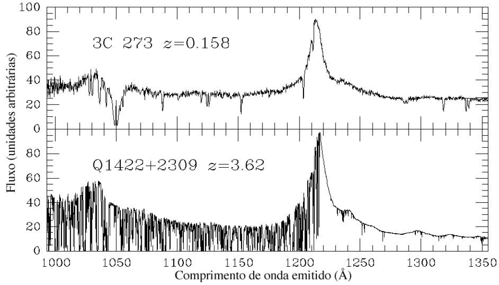
Figura 224: Comparação da floresta Ly \alpha de dois QSOs a redshifts diferentes. Figura tirada do curso de W. Keel, o espectro de 3C 273 foram obtidas pelo HST e o espectro de Q1422+2309 foi obtido com o Keck.
