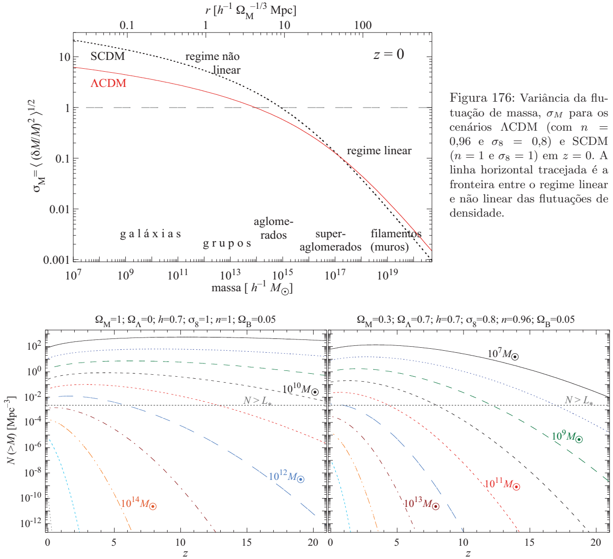
Figura 177: Distribuição de massas em função do redshift de halos colapsados (de 10^7 a 10^{16} M_\odot ). O traço horizontal indica o densidade numérica de galáxias com L > L_* na banda V no Universo próximo. Esquerda: SCDM. Direita: \Lambda CDM.
