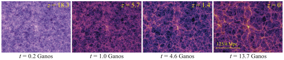
Figura 86: Sequência ilustrando a evolução da densidade (apenas matéria escura fria) da Simulação do Millennium (Springel et al., 2005), onde observamos a formação dos filamentos (“teia-cósmica”) e de halos de aglomerados de galáxias. Figura tirada do sítio: www.mpa-garching.mpg.de/galform/virgo/millennium
