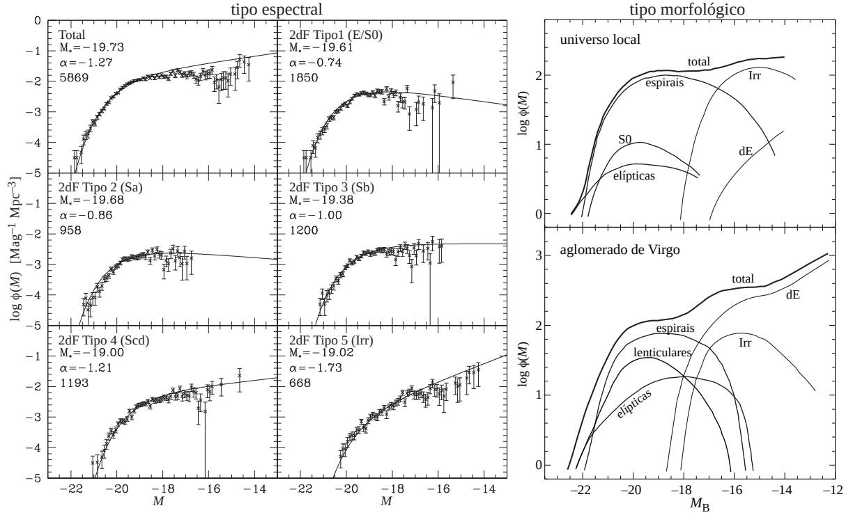
Figura 182: Esquerda: Função de luminosidade (incluindo correção K e incompleteza) segundo tipo espectroscópico. As linhas são ajustes da função de Schechter. Dados do survey 2dF (Folkes et al., 1999). Direita: Função de luminosidade segundo tipo morfológico para o campo (universo local) e para o aglomerado de Virgo (tirado de Binggeli et al., 1988).
