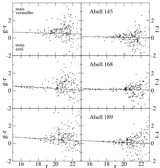
Figura 143: Relação cor–magnitude em três aglomerados. Os filtros g , r e i estão centrados em 5118 Å, 6798 Å e 8100 Å, respectivamente. As retas representam ajustes que correspondem à posição das galáxias elípticas (a chamada sequência vermelha das elípticas ). Figura tirada de ( Margoniner & de Carvalho, 2000 ).
