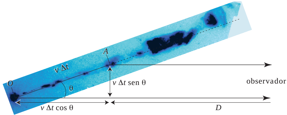
Figura 216: Geometria de um jato relativístico sendo ejetado de um núcleo ativo. “O” representa o núcleo e “A” um nó do jato que percorreu uma distância v\Delta t .
