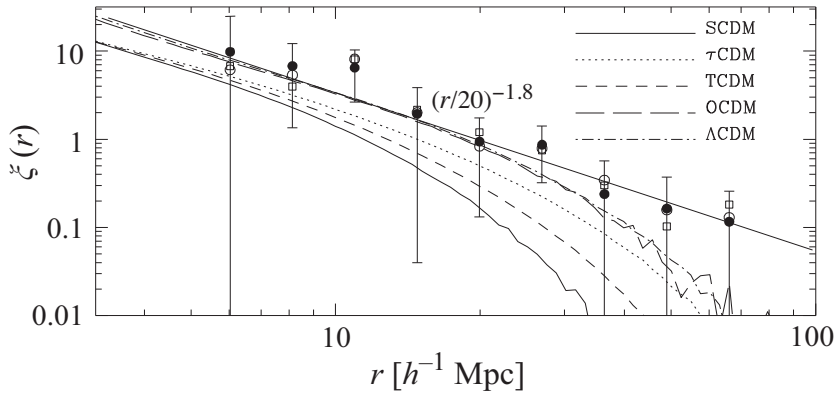
Figura 100: Função de correlação de aglomerados de galáxias selecionados em raios-X (dados do ROSAT All-Sky Survey (RASS) Moscardini et al., 2000) e comparação com modelos cosmológicos.
