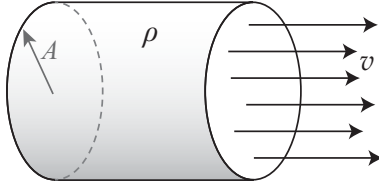
Figura 148: O gás intra-aglomerado passando por uma seção circular de raio A produz uma pressão equivalente à pressão sentida por uma galáxia que se move pelo meio intra-aglomerado.
