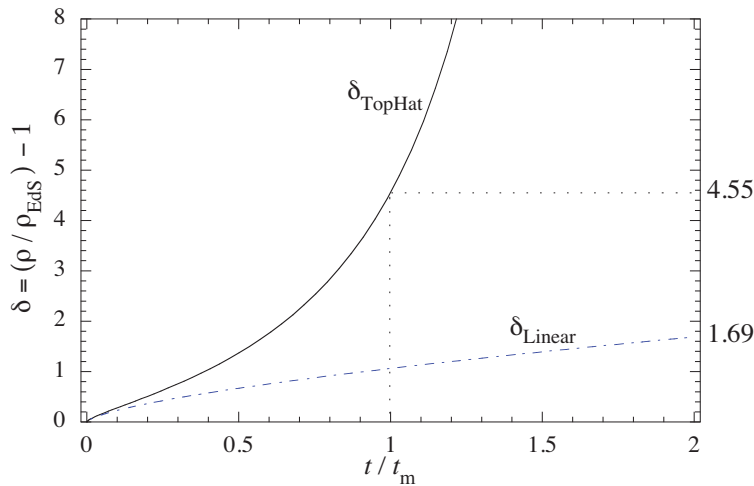
Figura 169: Evolução do contraste de densidade do modelo Top-Hat (linha contínua) comparado com a aproximação linear (ponto-traço). O valor do contraste de densidade no momento do ‘turn-around’ e da extração linear no momento do colapso são mostrados à direita. \rho_{\text{EdS}} é a densidade média do Universo (aproximação de Einstein–de Sitter).
