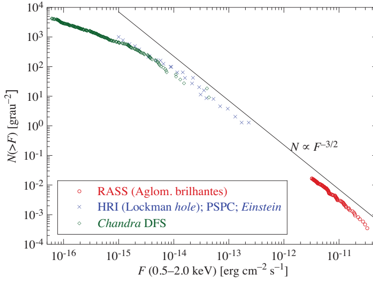
Figura 35: Número de fontes de raios-X por grau quadrado com densidade de fluxo superior a F . A reta N \propto F^{-3/2} serve como comparação. Para fluxo baixo, os dados vêm do Chandra Deep Field South (Tozzi et al., 2001); para fluxo intermediário, do ROSAT PSPC, HRI (Lockman Hole) e Einstein IPC (Gunn, 1999); para fluxo elevado, do ROSAT All Sky Survey (De Grandi et al., 1999).
