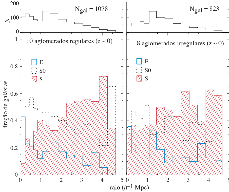
Figura 141: Relação entre o tipo morfológico e a distância do centro do aglomerado ( T-R ). O histograma no alto de cada painel mostra o número de galáxias para cada intervalo de raio (dados de Dressler 1980, cf. Dressler et al., 1997).
