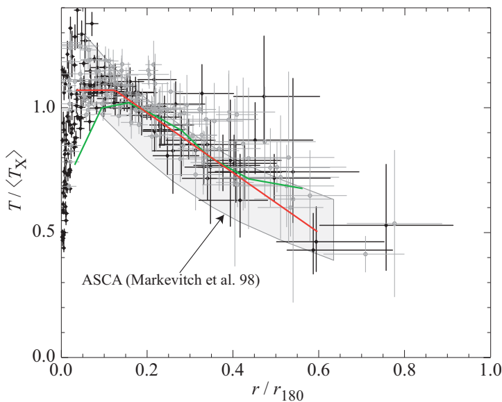
Figura 128: Perfil de temperatura de aglomerados. Os eixos estão escalonados, em unidades de r_{180} (aproximadamente o raio do virial, veja Sec. 8.1) e pela temperatura média (excluindo a região do cool-core (Sec. 5.9). Figura baseada em Vikhlinin et al. (2005) (pontos pretos, Chandra ) e Pratt et al. (2007) (pontos cinzas, XMM).
