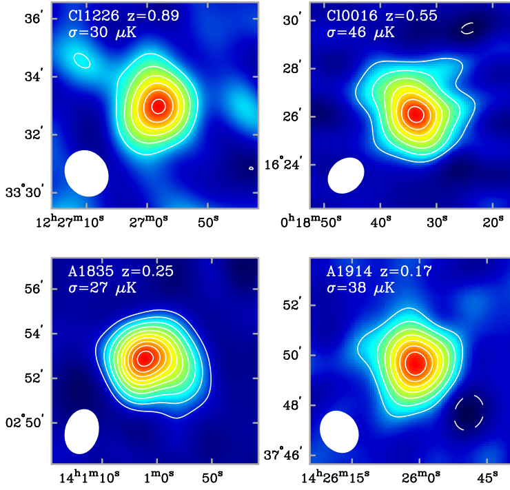
Figura 126: Efeito SZ observados em aglomerados a diferentes redshifts ; para aglomerados com luminosidades em raios-X semelhantes, o sinal do efeito SZ é aproximadamente o mesmo. O efeito SZ não depende da distância do aglomerado. Os níveis traçados em linhas contínuas correspondem a \Delta T_{\text{CMB}}/T_{\text{CMB}} < 0 . A elipses nos cantos representam a largura da PSF ( point spread function ) a meia-altura (FWHM). Figura tirada de Reese (2003).
