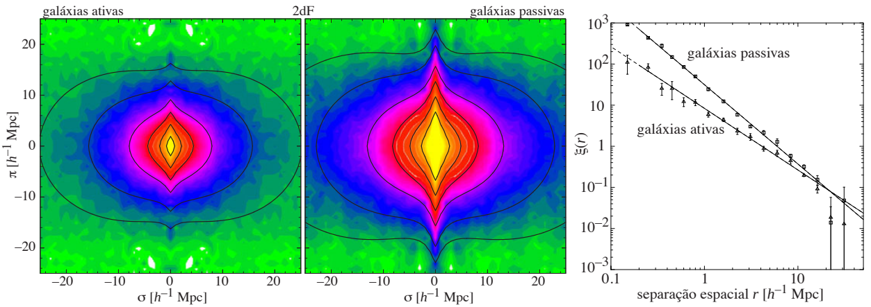
Figura 243: Esquerda e centro: Função de correlação bidimensional, \xi(\sigma, \pi) (seção 4.3.1 para definições) para galáxias com baixa taxa de formação estelar (SFR atual \leq 10\% que a média durante a vida pregressa, i.e., galáxias “passivas”) e com alta taxa de formação estelar (galáxias “ativas”). Direita: Função de correlação \xi(r) dos dois tipos de galáxias. Galáxias passivas se aglomeram mais do que as ativas em escalas menores que \sim 10 h^{-1} \text{ Mpc} . Dados do 2dFGRS, figura tirada de Madgwick et al. (2003).
