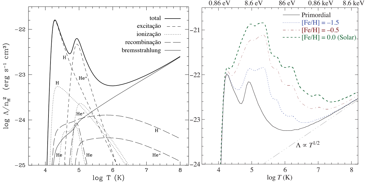
Figura 172: Esquerda: Taxas de resfriamento de um gás primordial ( X = 0.76 ); Direita: com diferentes metalicidades. A taxa total é dada pela linha mais espessa. Para baixa temperatura, o resfriamento é dominado por excitação colisional; para temperatura alta, pela emissão bremsstrahlung. Figura da esquerda tirada de Weinberg, Hernquist & Katz (1997) ; a direita de Sutherland & Dopita (1993) .
