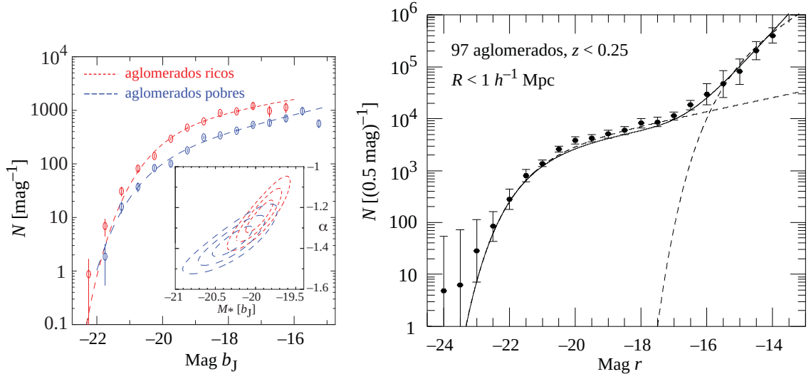
Figura 184: Esquerda: Funções de luminosidade de aglomerados de galáxias ricos e pobres. Direita: Função de luminosidade combinada de quase uma centena de aglomerados de galáxias ricos, chegando até as galáxias anãs ( Mr \sim -14 ). Figura adaptada de de Propriis et al. (2003) e Popesso et al. (2005) .
