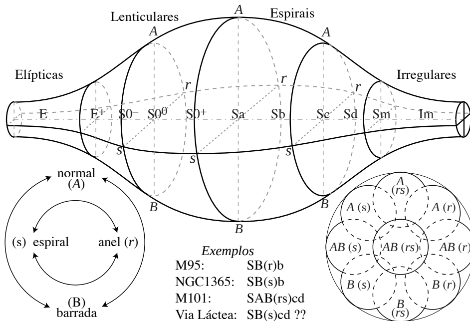
Figura 247: Classificação morfológica de de Vaucouleurs (1959) em três dimensões, dando igual importância às barras e aos anéis.
