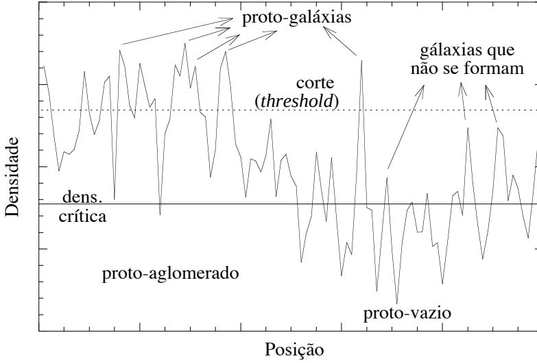
Figura 102: Formação de galáxias com bias . Picos de densidade em uma região de densidade globalmente abaixo da média, mesmo acima da densidade crítica, não formam galáxias. Neste caso, galáxias formadas não traçam a distribuição de massa do Universo (o comprimento de correlação das galáxias é menor do que se esperaria).
