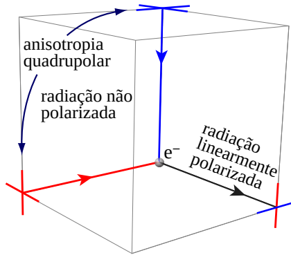
Figura 64: A radiação não polarizada, mas com anisotropia de quadrupolo (representada pelos eixos vermelho e azul, perpendiculares) ao ser espalhada por um elétron livre produz uma radiação linearmente polarizada. Figura tirada de Hu & White (1997).
