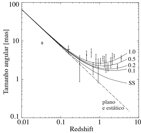
Figura 31: Tamanho angular mediano (em milissegundos de arco) de uma fonte com dimensão 9,6h^{-1} pc em função do redshift . As linhas representam modelos cosmológicos com \Omega_\Lambda = 0 e q_0 = 0,1, 0,2, 0,5 e 1,0 . A curva “SS” representa o modelo “Steady-State”. Figura tirada de Gurvits et al. (1999)
