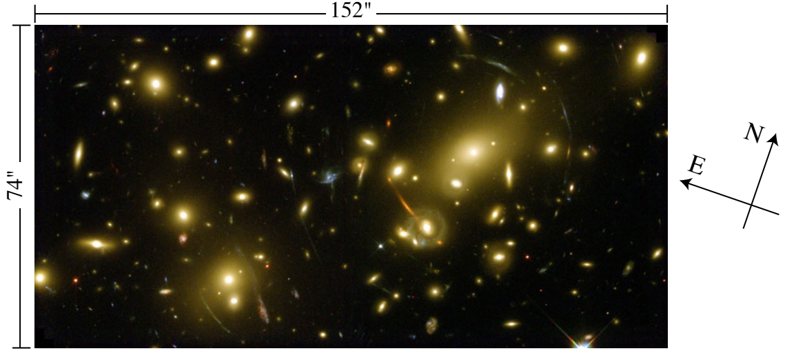
Figura 134: Abell 2218 ( z = 0,1756 , 1'' = 3h_{70}^{-1}\text{kpc} ) observado pela WFPC2 do telescópio Hubble em janeiro/2000. Figura tirada do site do HST .
