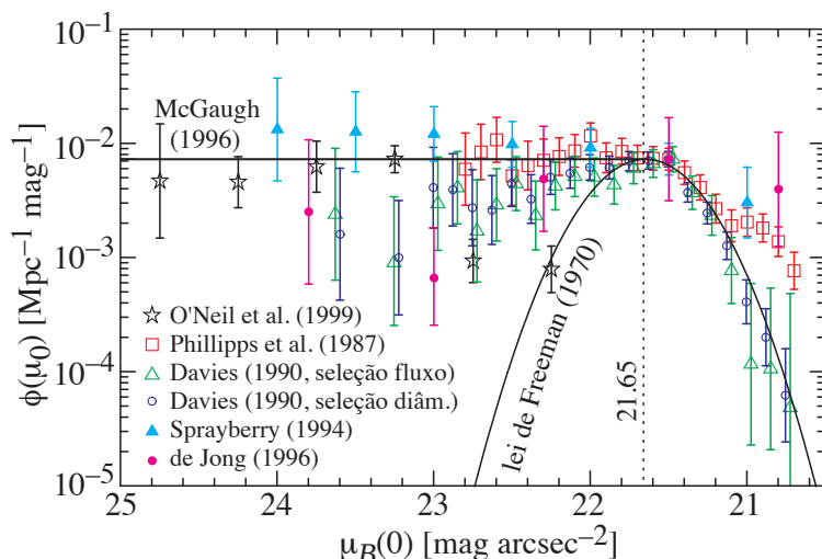
Figura 251: Função de distribuição de brilho superficial central. Para comparação, está traçada a “Lei de Freeman”. Figura tirada de O’Neil & Bothun (2000).
