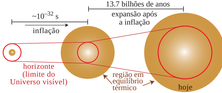
Figura 51: Durante a inflação, o fator de escala aumenta exponencialmente, enquanto o horizonte (representado pelo círculo) se expande na velocidade da luz. Em um instante inicial, toda a região em equilíbrio termodinâmico está no interior do horizonte. Figura baseada em Watson (2000) .
