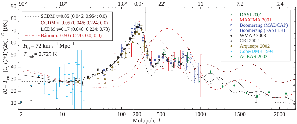
Figura 59: Espectro de potência multipolar (angular) da CMB. Os parâmetros dos modelos teóricos (alguns exemplos, calculados com cmbfast ) estão na legenda à esquerda. Os números entre parênteses são, respectivamente: \Omega_B , \Omega_{\text{cdm}} (apenas matéria escura) e \Omega_\Lambda . A densidade total de matéria é \Omega_M = \Omega_B + \Omega_{\text{cdm}} .
