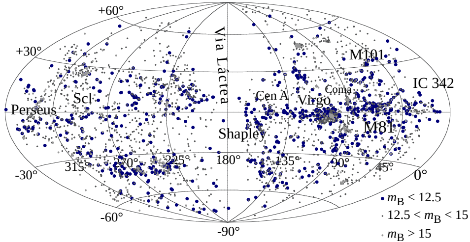
Figura 87: Distribuição de galáxias próximas em coordenadas supergalácticas, com destaque à distribuição quase plana do super-aglomerado local com centro em Virgo. As galáxias estão separadas por intervalo de magnitude aparente, dando grosseiramente uma informação sobre a distância das estruturas observadas. Figura feita com um subconjunto de galáxias do catálogo RC3.
