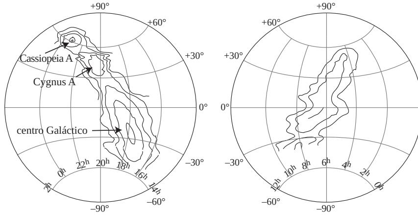
Figura 13: Isocontornos em rádio (160 MHz) da Via Láctea obtida por Reber (1944) onde podemos ver o centro da Galáxia, Cas A (um resto de supernova) e a primeira rádio-galáxia observada, Cygnus A. A projeção é de Airy em coordenadas equatoriais.
