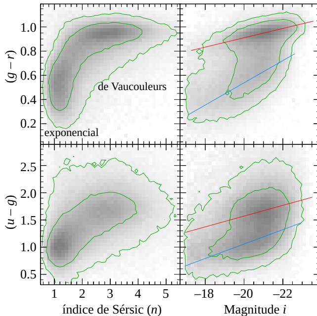
Figura 257: Relações cor–magnitude–índice de Sérsic onde o nível de cinza representa a densidade de luminosidade, \sum_i L_i/V_{i,\max} , de \sim 183.000 galáxias, mostrando o caráter bimodal da distribuição das propriedades das galáxias. Nos diagramas cor–magnitude são mostradas a Sequência Vermelha das elípticas e a Sequência Azul das espirais. Nas relações com o índice de Sérsic, n = 4 corresponde ao perfil de de Vaucouleurs e n = 1 corresponde a perfis exponenciais. Figura adaptada de Blanton et al. (2003)
