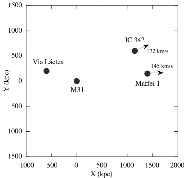
Figura 164: Posições da Via Láctea, M31, Maffei 1 e IC 342 em coordenadas supergalácticas. Como Maffei 1 e IC 342 estão praticamente no plano supergaláctico, a representação bidimensional é uma boa aproximação da situação em 3 dimensões. (Figura tirada de Valtonen et al., 1993)
