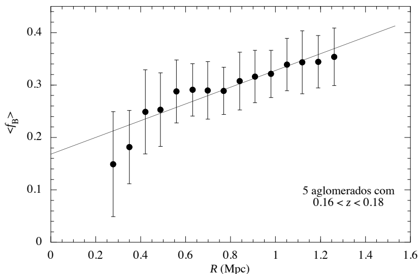
Figura 146: Dependência da fração de galáxias azuis com a distância ao centro do aglomerado (Margoniner & de Carvalho, 2000)
