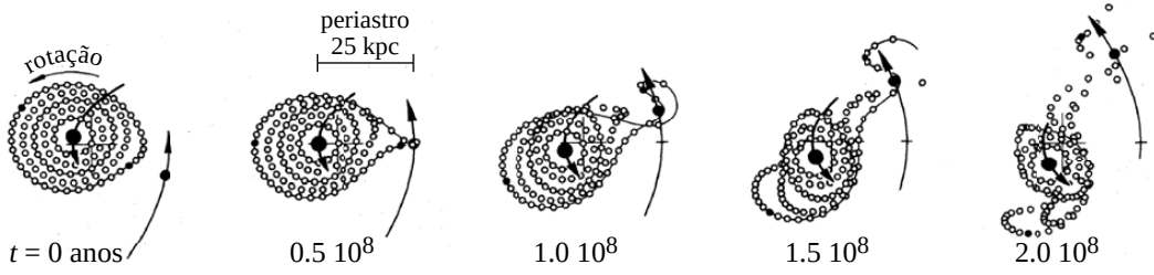
Figura 195: Simulação mostrando a formação de braços espirais devido à passagem de uma galáxia com 1/4 da massa da primária em órbita no plano do disco. Figura baseada em Toomre & Toomre (1972) .
