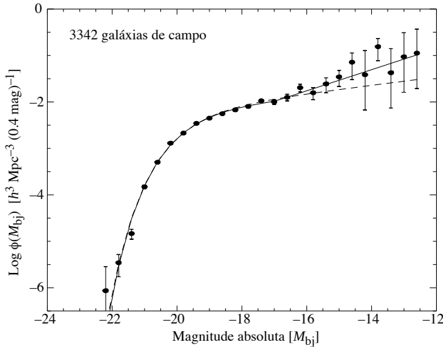
Figura 183: Função de luminosidade de galáxias de campo (em número de galáxias h^3 \text{ Mpc}^{-3} em bins de 0,4 mag) para 3342 galáxias mais brilhantes que M_{bj} = -12,4 + 5 \log h . As linhas pontilhada e contínua correspondem a um ajuste de uma função de Schechter única e um ajuste de Schechter mais uma lei de potência [Eq. (381)], respectivamente (Zucca et al., 1997).
