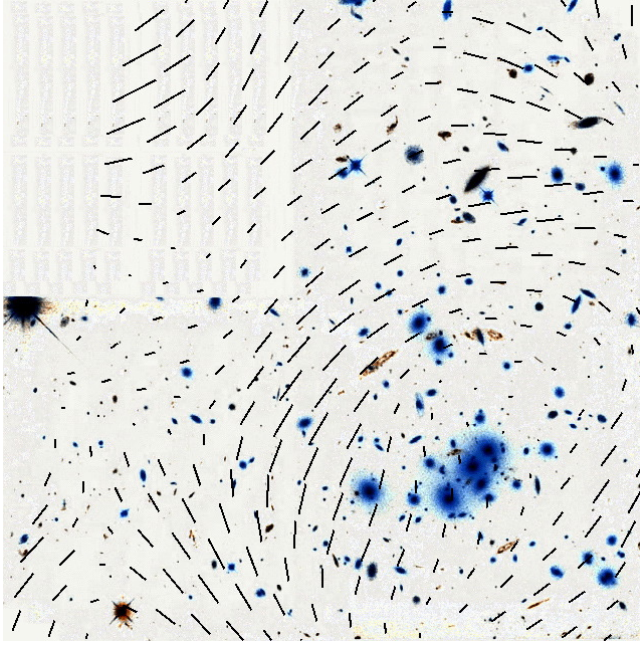
Figura 136: Campo de cisalhamento superposto na imagem do HST do aglomerado Cl0024. Cada traço representa a elipticidade e orientação médias das galáxias de fundo na região próxima ao traço. Figura tirada de Narayan & Bartelmann (1996) .
