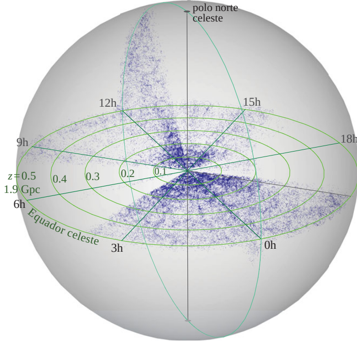
Figura 94: Distribuição das galáxias com velocidade medida do SDSS-DR12 compreendendo uma faixa entre -2,5^\circ \leq \delta \leq +2,5^\circ em todo o equador celeste e uma faixa perpendicular entre a ascensão reta 0^h e 12^h . Note que os lados opostos não têm a mesma completude. Neste gráfico temos um pouco menos de 180 mil galáxias. Compare a dimensão radial deste survei com o das Las Campanas, Fig. 93.
