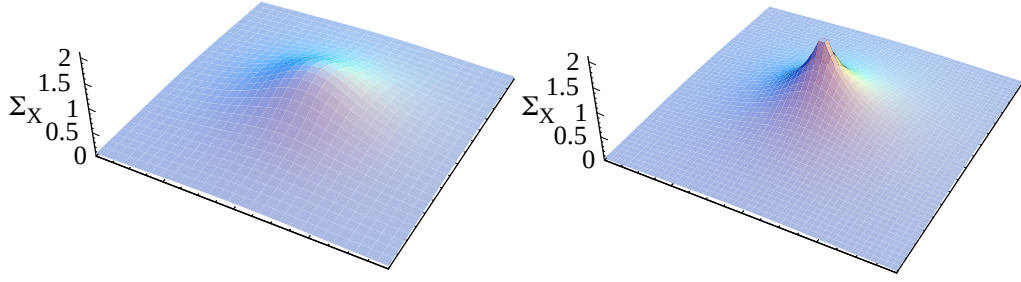
Figura 138: Mapa de emissão em raios-X 3D comparando de um aglomerado sem “cool-core” (esquerda) com um aglomerado com “cool-core” (direita). A primeira evidência observacional é o excesso de emissão central em comparação com o modelo \beta , Eq. (271).
