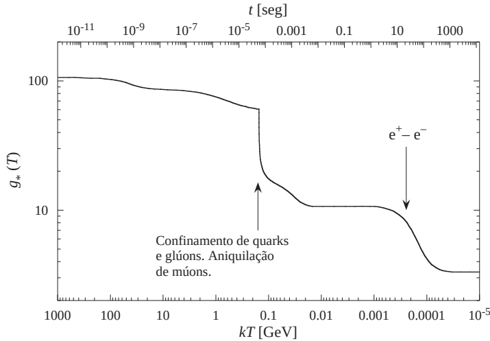
Figura 18: Evolução do número de graus de liberdade efetivos, g_* em função da temperatura do Universo. Acima, a escala de tempo após o Big Bang assumindo um universo \Lambda CDM.
