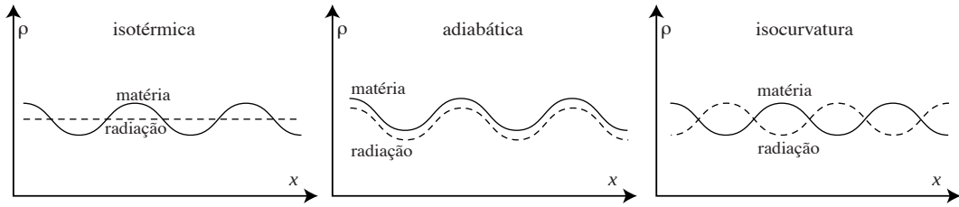
Figura 75: Perturbações de densidade isotérmica, adiabática e isocurvatura.
