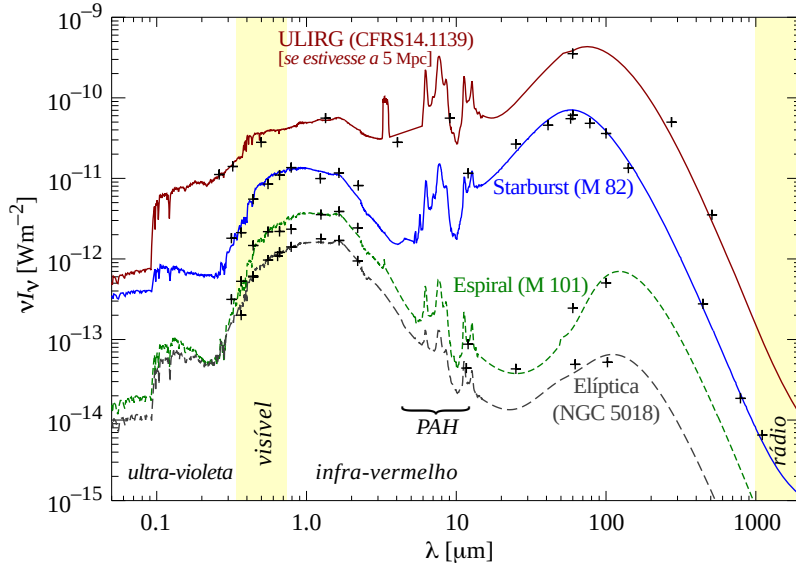
Figura 157: Distribuição espectral de energia de uma ULIRG comparada com galáxias normais e uma starburst próximas da Via Láctea. A SED da ULIRG foi normalizada, colocando-a a 5 Mpc de distância (CFRS14.1139 tem z = 0,66 ). Note a semelhança das SEDs, no infravermelho, entre a ULIRG e a starburst, M82. Figura adaptada de Galliano (2004) .
