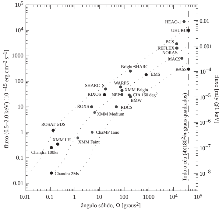
Figura 115: Área coberta (ângulo sólido) e fluxo limite de diversos surveys realizados em raios-X. As linhas tracejadas correspondem, de cima para baixo, a 100, 1000 e 10000 fontes detectáveis na banda 0,5–2,0 keV. Figura baseada em Brandt et al. (2001) ; Rosati et al. (2002)
