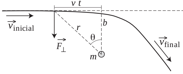
Figura 191: Geometria de um encontro gravitacional de uma partícula teste com um corpo de massa m .
