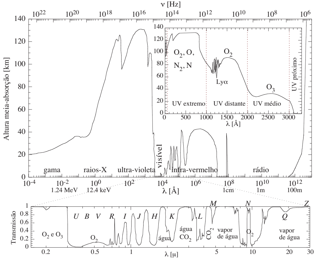
Figura 262: Transparência da atmosfera em função do comprimento de onda ou frequência dado em termos da altitude onde metade do fluxo incidente na Terra é absorvido pela atmosfera. Nos detalhes temos a região do ultravioleta (UV) e infravermelho, com suas diversas bandas fotométricas (que em geral coincidem com as janelas).
