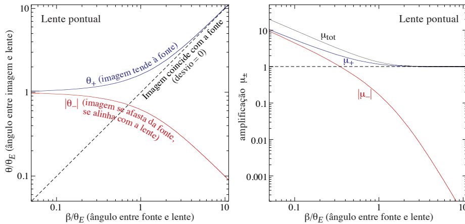
Figura 131: Esquerda: Posição das imagens criadas por uma lente gravitacional pontual, \theta_+ e |\theta_-| , cf. Eq. (255). Direita: amplificação da luminosidade para as imagens produzidas por uma lente pontual, cf. Eq. (257).
