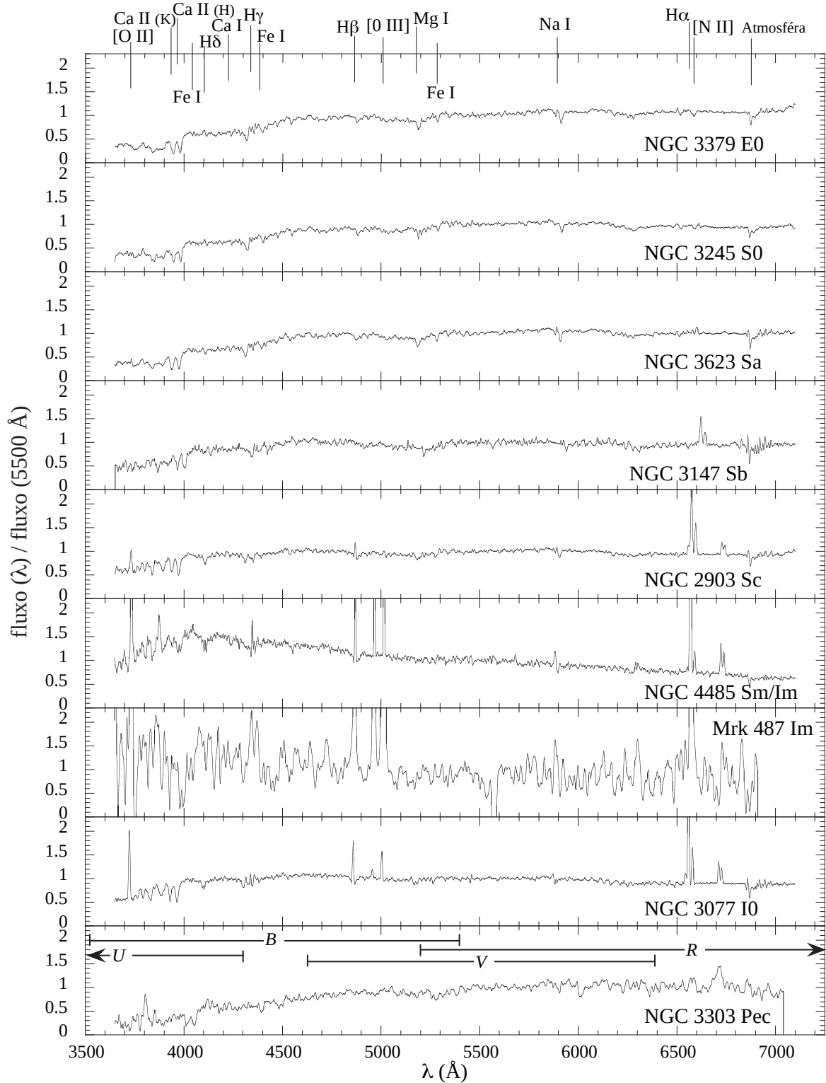
Figura 254: Espectro de galáxias normais do catálogo de Kennicutt (1992). Algumas linhas espectrais mais importantes e os filtros do sistema UBVR são mostrados. A galáxia NGC3303 é na realidade um par de galáxias em processo de fusão.
