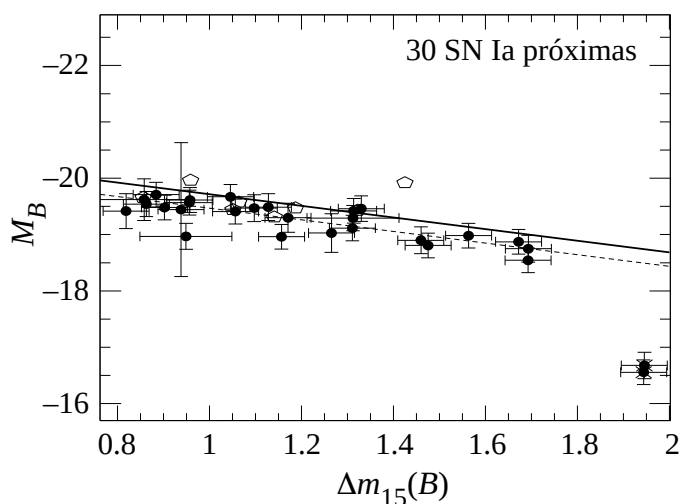
Figura 260: Relação entre a luminosidade máxima na banda B e a diminuição do brilho em 15 dias para supernovas de Tipo Ia. Figura tirada de Turatto (2003).
