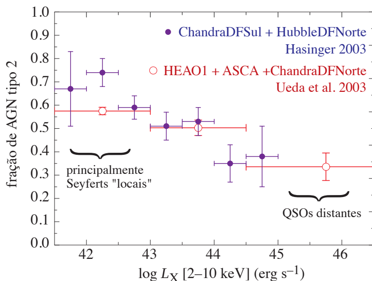
Figura 211: Fração de AGNs tipo 2 em função da luminosidade em raios-X. No Universo local cerca de 60% das AGNs são de tipo 2. Esta proporção diminui em AGNs mais potentes em raios-X. Figura tirada de Hasinger (2003) .
