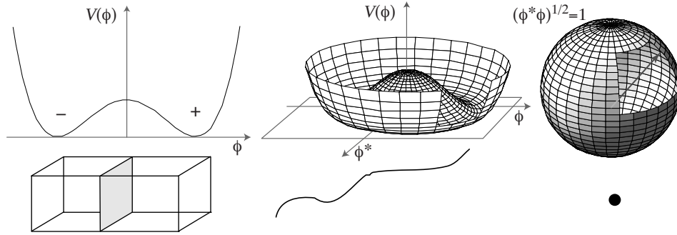
Figura 74: Defeitos topológicos devido à quebra de simetria do campo escalar \phi . Esquerda: “domain wall”; Meio: “string”; Direita: monopolo.
