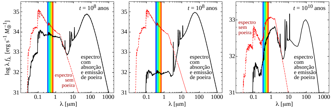
Figura 208: Alteração da distribuição de energia espectral devido à presença de poeira em uma galáxia tipo espiral vista de face. Esquerda: espectro estelar (linha vermelha, fina) de uma galáxia jovem (ainda com alta taxa de formação estelar) comparado ao espectro na presença de poeira (traço espesso). Note a absorção em baixo comprimento de onda e a emissão no infra-vermelho distante. Centro: a mesma galáxia jovem, mas com uma quantidade maior de poeira. Direita: galáxia espiral típica, com 10^{10} anos, baixa taxa de formação estelar e a mesma quantidade relativa de poeira que no painel da esquerda. Figura baseada em Devriendt et al. (1999) . Veja também a Fig. 157, pag. 147, para o efeito da poeira em ULIRGs, galáxias com formação estelar ultraluminosas no infravermelho.
