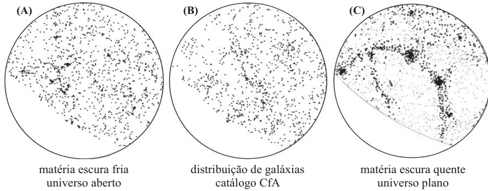
Figura 84: Simulações numéricas com 32768 ( 32^3 ) partículas em uma grade cúbica de (A) um universo aberto dominado por CDM e \Omega_M = 0,2 e (C) universo plano dominado por HDM. No centro, (B) uma distribuição comparável às simulações das galáxias do catálogo do CfA (veja Sec. 4.2). Figura tirada de Frenk (1986) [veja também Davis et al. (1985) ].
