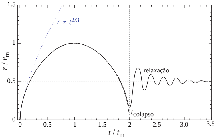
Figura 170: Evolução do raio de uma esfera no modelo “Top-Hat”. A linha tracejada é o modelo como escrito na seção anterior (Fig 169), a linha pontilhada é a aproximação linear e o traço contínuo representa a evolução, baseado em simulações numéricas. Após o colapso, a esfera relaxa (virializa) rapidamente.
