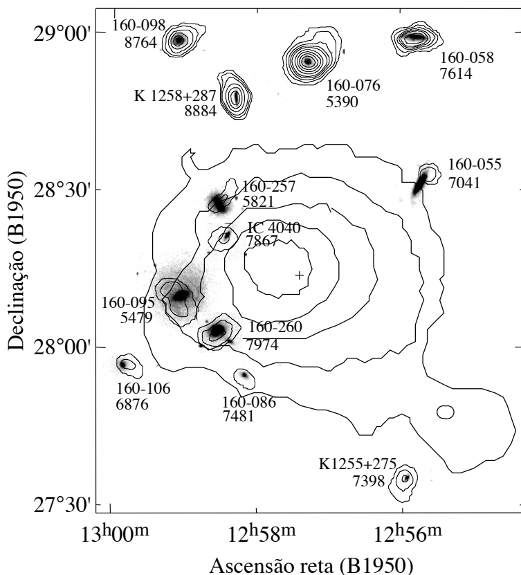
Figura 147: Efeito da pressão de arraste em Coma. Os contornos espessos representam a emissão em raios-X, os contornos finos representam a emissão de HI, superpostas às imagens ópticas (níveis de cinza) das galáxias (ampliadas por um fator 7). Cada objeto tem sua identificação e velocidade de recessão (em km/s). A cruz central corresponde à elíptica gigante NGC 4874. Figura tirada de Bravo-Alfaro et al. (2000).
