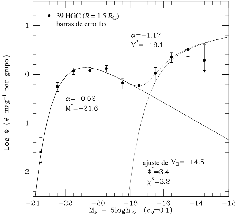
Figura 186: Função de luminosidade dos Grupos compactos de Hickson. As populações brilhantes e fracas são ajustadas separadamente com 2 funções de Schechter (uma única função não ajusta bem os dados). Linha contínua: parte brilhante; linha pontilhada: parte fraca; linha tracejada: ajuste composto. Dados obtidos na banda R (Hunsberger et al., 1998).
