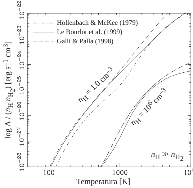
Figura 174: Função de resfriamento para o hidrogênio molecular, calculado para duas densidades médias diferentes, representando o regime de alta e baixa densidade do meio. Figura tirada de Glover (2005).
