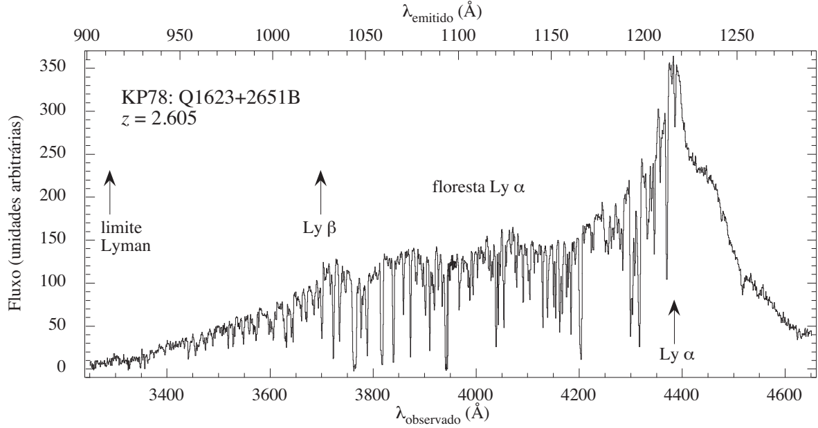
Figura 222: Espectro do QSO 1623+2651B (Crotts & Fang, 1998). Estão indicados os comprimentos de onda das linhas Ly \alpha e Ly \beta ( \lambda_\alpha = 1216 \text{ \AA} e \lambda_\beta = 1026 \text{ \AA} , respectivamente).
