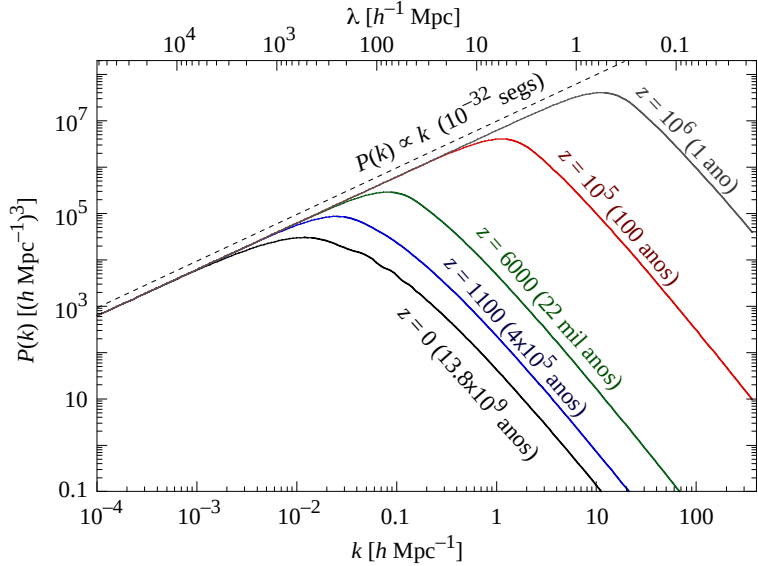
Figura 79: Evolução do espectro de potência. Após a inflação, P(k) \propto k^n com n \approx 1 . As perturbações de densidade que entram no horizonte são amortecidas e surge o “turnover”. O espectro de potência evolui até o momento da equipartição matéria-radiação. O figura é baseada em um cenário \Lambda CDM.
