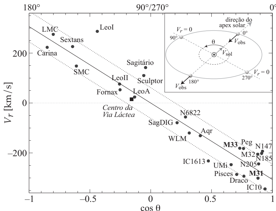
Figura 165: Velocidades heliocêntricas, V_r dos membros do Grupo Local em função de \cos \theta , onde \theta é a distância angular do apex solar (direção do movimento do Sol no Grupo Local Courteau & van den Bergh, 1999 ). Nesta figura, o movimento do Sol é de 306 \pm 18 \text{ km s}^{-1} na direção de \ell = 99^\circ \pm 5^\circ e b = -3^\circ \pm 4^\circ (linha sólida). As linhas pontilhadas correspondem a uma dispersão radial de \pm 61 \text{ km s}^{-1}
