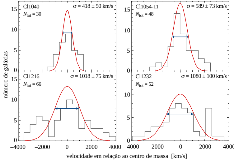
Figura 127: Distribuição de velocidades em quatro aglomerados de galáxias, ajustadas por uma gaussiana. As dispersões, \sigma , de cada gaussiana estão indicadas para cada aglomerado. Figura tirada de Halliday et al. (2004) .
