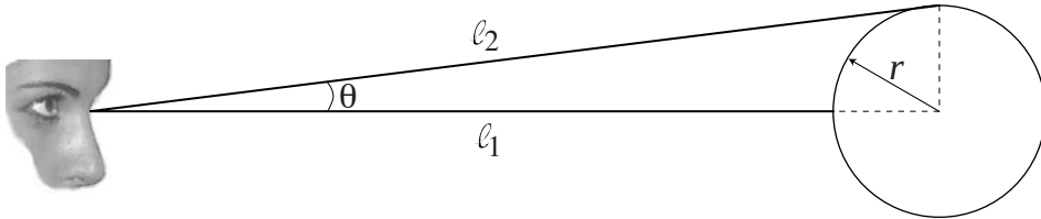
Figura 231: Diferença entre os percursos de fóton emitido na borda e no centro de uma fonte esférica.
