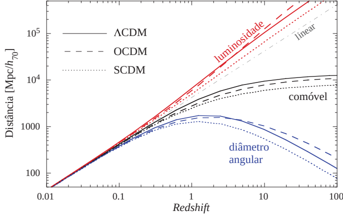
Figura 30: Comparação das distâncias comóvel, diâmetro angular e luminosidade para diferentes modelos cosmológicos; \Lambda CDM e SCDM são planos, OCDM é aberto, sem energia escura. Para um dado redshift , as distâncias em um Universo \Lambda CDM são sempre maiores do que em um universo plano sem energia escura. Note que o modelo OCDM tem um comportamento mais próximo de um \Lambda CDM. A linha ponto-traço fina mostra a relação linear entre redshift e distância, válida apenas para baixo z .
