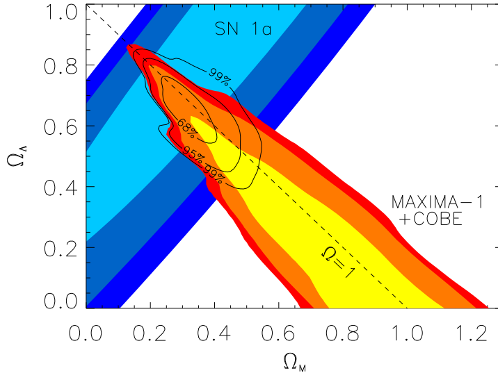
Figura 63: Limites de confiança dos parâmetros cosmológicos obtidos com a análise de dados do COBE e MAXIMA-1 combinados com as SN Ia (veja Fig. 46). Estes dados implicam em \Omega_\Lambda = 0,65^{+0,15}_{-0,16} e \Omega_M = 0,32^{+0,14}_{-0,11} . Figura tirada de Stompor et al. (2001).
