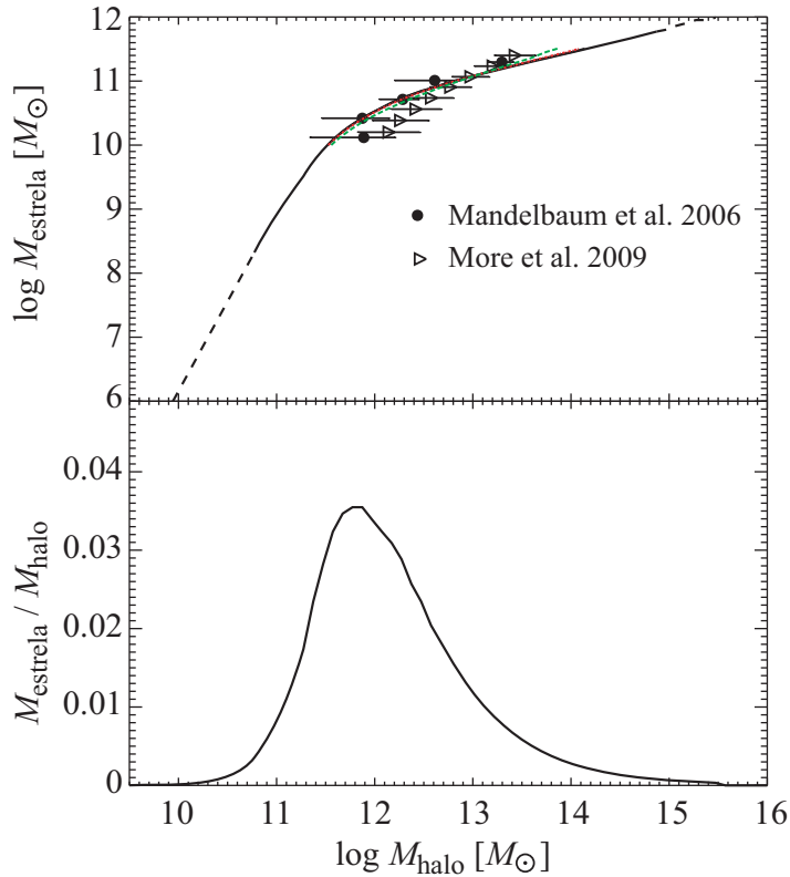
Figura 190: Acima: Relação entre a massa estelar e a massa total do halo. A linha contínua é obtida usando uma correspondência entre a função de luminosidade das galáxias do SDSS-DR7 com a função de massa das simulações do Millennium (a linha tracejada é uma extrapolação desta relação). Abaixo Razão entre massa estelar e massa total em função da massa total do halo. Figura tirada de Guo et al. (2010).
