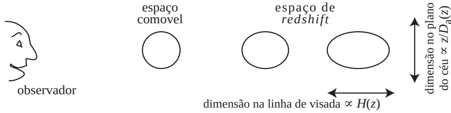
Figura 105: Ilustração do efeito Alcock–Paczynski, da deformação aparente de uma distribuição esférica quando observado no espaço de redshift .
