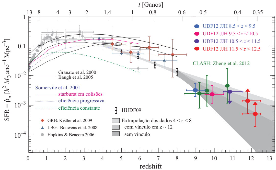
Figura 206: Taxa de formação estelar, SFR, em função do redshift ( diagrama de Madau-Lilly ). Os pontos observacionais foram corrigidos levando-se em conta a completude da contagem de objetos e a extinção devido à poeira. A SFR em alto redshift foi estimada usando Gamma Ray Bursts (GRB) e Lyman Break Galaxies (LGB). As curvas representam vários modelos semi-analíticos de diferentes taxas de formação estelar, para um modelo hierárquico \Lambda CDM. Figura tirada de Ellis et al. (2013) ; Kistler et al. (2009) ; Baugh et al. (2005) e Somerville et al. (2001) [veja também Ellis (2001) ].
