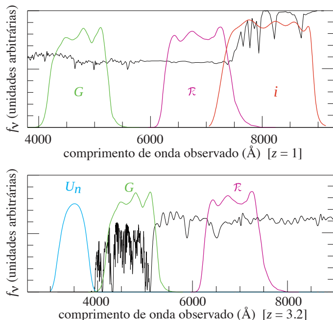
Figura 203: Exemplo da técnica de identificação de galáxias pela cor. Superpostos aos espectros (sintéticos) estão os perfis de transmissão de cada filtro (definidos em Steidel et al. (1996) ). As quebras de Balmer e Lyman (no alto e abaixo, respectivamente) fazem com que as galáxias a estes redshifts tenham cores bem características. As galáxias identificadas pela quebra de Lyman são frequentemente chamadas “ Lyman Break Galaxies ”
