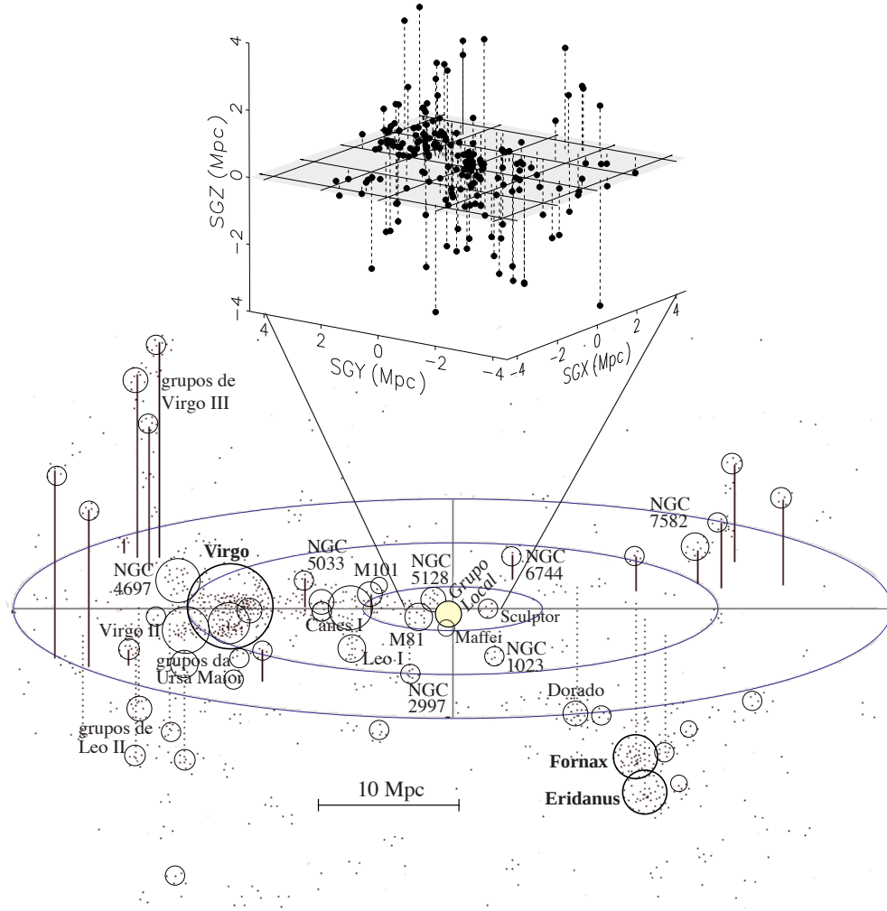
Figura 159: Acima: Plano Super-Galáctico com as galáxias mais próximas da Via Láctea. Figura tirada de (Carroll & Ostie, 1996, cap. 25). Abaixo: Super-aglomerado local.
