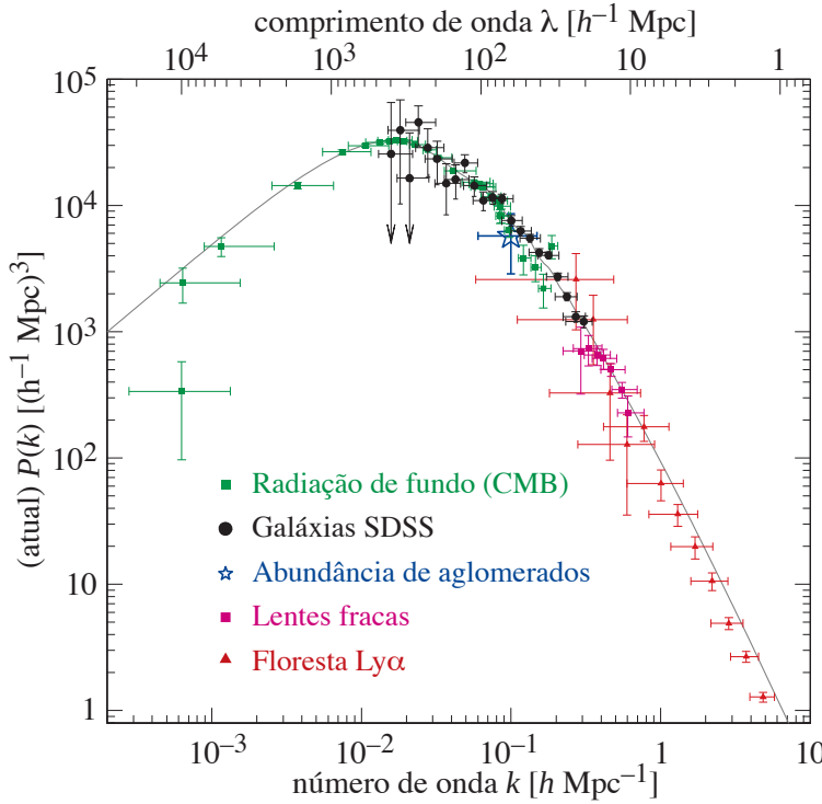
Figura 77: Espectro de potência das flutuações de densidade determinados a partir de diversas técnicas (note que cada uma é mais sensível para um certo intervalo de número de onda k ). O traço contínuo representa um modelo com \Omega_{\Lambda} = 0,72 , \Omega_M = 0,28 e h = 0,72 , com perturbações iniciais independente de escala ( n = 1 ) e profundidade óptica até a superfície de último espalhamento \tau = 0,17 (cf. seção 12). Figura tirada de Tegmark et al. (2004).
