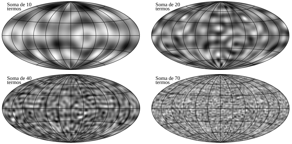
Figura 60: Soma dos primeiros termos dos harmônicos esféricos, ilustrando como podemos reproduzir a observação das flutuações de temperatura da radiação cósmica de fundo. Aqui usamos fases aleatórias, como é normalmente assumido, e um espectro de potência de ruído branco (diferente da CMB). Para reproduzirmos a imagem da CMB obtida pelo satélite WMAP, precisaríamos somar mais de 1500 termos.
