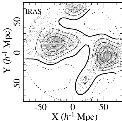
Figura 108: Distribuição de massa no Universo local obtida a partir da distribuição de galáxias IRAS. Note a semelhança com a Fig. 106. Figura tirada de Sigad et al. (1998).
