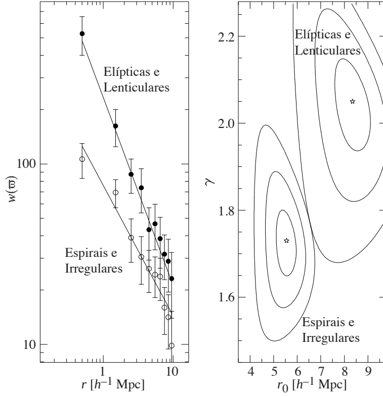
Figura 98: Dependência da função de correlação segundo o tipo morfológico. Figura tirada de Guzzo et al. (1997).
