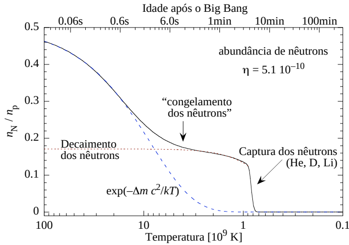
Figura 53: Evolução da abundância de nêutrons livres em função da temperatura (e idade) do Universo. A curva tracejada corresponde à Eq. (103), a curva pontilhada ao decaimento do nêutron. A queda abrupta da abundância corresponde à captura dos nêutrons restantes nos núcleos de He, D e Li.
