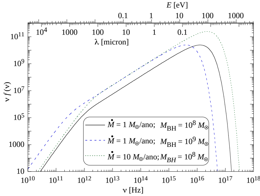
Figura 233: Espectro contínuo do disco de acreção calculado usando a Eq. (452), ilustrando o efeito de diferentes massas do buraco negro central supermaciço e da taxa de acréscimo de matéria.
