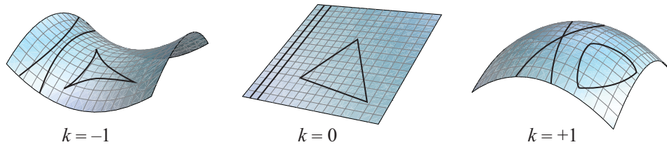
Figura 28: Representação da curvatura de uma superfície bidimensional em um espaço de três dimensões. Por exemplo, a soma dos ângulos internos de um triângulo depende da curvatura do espaço. Para o nosso Universo, basta imaginar esta figura em 4 dimensões...
