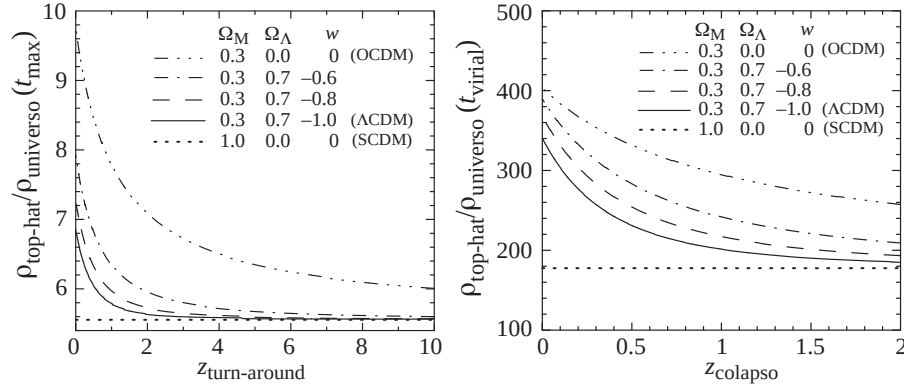
Figura 171: Esquerda: Contraste de densidade no momento de máxima expansão do Top-Hat (isto é, momento do turn-around ). Compare com a Fig. 169 e \delta_{\text{turn-around}} = (3\pi/4)^2 - 1 \approx 4,552 . Direita: Contraste de densidade do Top-Hat virializado; para o modelo SCDM, \rho_{\text{TH}} = 177,7\rho_{\text{EdS}} . Modelos com -1 < w < -1/3 são de quintessência. Figura tirada de Horellou & Berge (2005).
