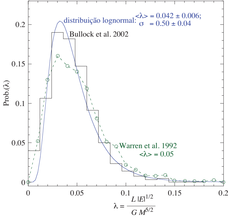
Figura 179: Distribuição do parâmetro de rotação de halos formados em simulações de Universos dominado por CDM (cenário hierárquico). A linha contínua representa a distribuição lognormal, Eq. (360).
