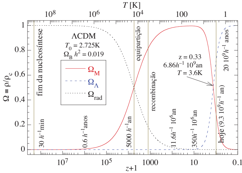
Figura 38: Variação dos parâmetros de densidade, \Omega em função do redshift e temperatura da radiação para o caso \Lambda CDM. As linhas verticais marcam algumas etapas importantes: fim da nucleossíntese primordial, equipartição matéria-radiação, recombinação (último espalhamento da CMB), equipartição matéria-energia escura.
