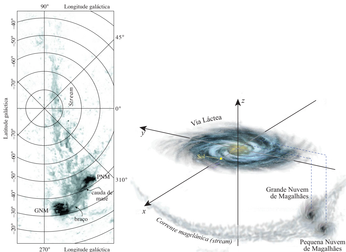
Figura 166: Esquerda: Mapa mostrando as Nuvens de Magalhães (LMC e SMC, grande e pequena, respectivamente), e a Magellanic Stream . Os níveis de cinza correspondem à densidade de coluna do hidrogênio neutro, variando logaritmicamente de 2 \times 10^{18} a 6 \times 10^{20} \text{ cm}^{-2} (Putman, 1999). Na figura também estão indicados o braço ‘ leading ’ da LMC e a cauda de maré da SMC. Note a ausência de uma contrapartida da Magellanic Stream na direção oposta. Direita: Ilustração tri-dimensional das posições das Nuvens de Magalhães, Via Láctea e da Magellanic Stream (D. Parr, CSIRO media release 98/194).
