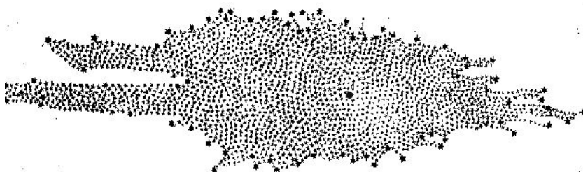
Figura 2: Modelo de Universo de Herschel 1785 baseado em contagens de estrelas. O Sol está aproximadamente no centro (círculo cinza) e a distribuição mostra um achatamento.
