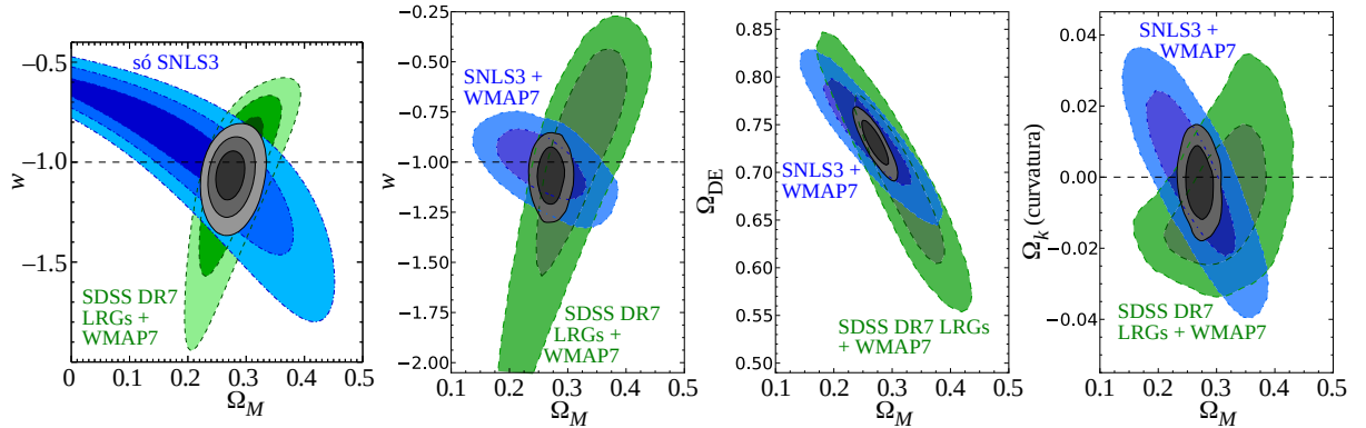
Figura 47: Determinação dos parâmetros cosmológicos com uma amostra de 472 supernovas de tipo Ia, junto com observações da CMB e o espectro de potência de galáxias (discutido na Sec. 3.4). O painel mais a esquerda utiliza um método de ajuste dos parâmetros de \chi^2 ; os contornos correspondem a 68,3%, 95,4% e 99,7% de confiança. Nos outros casos, é usado um método de Markov-Chain Monte Carlo (MCMC) e os contornos são de 68.3% e 95.4% de confiança. Os contornos cisas correspondem à combinação de todos os vínculos cosmológicos. O valor para a energia escura que corresponde à constante cosmológica é w = -1 e uma geometria plana é \Omega_k = 0 . Figura adaptada de Sullivan et al. (2011).
