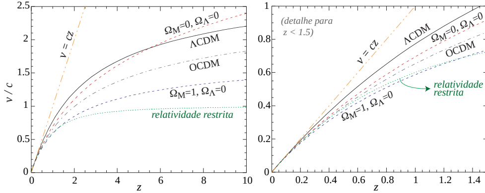
Figura 44: Relação entre a velocidade de recessão de um objeto de redshift z no momento em que é observado para diferentes modelos cosmológicos. Para comparação, também é mostrado a relação v(z) do efeito Doppler da relatividade restrita.
