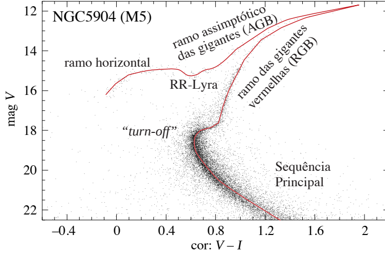
Figura 42: Diagrama cor-magnitude do aglomerado M5. A curva contínua representa a isócrona que melhor se ajusta, correspondendo a uma idade de 12 bilhões de anos. Dados do grupo de Padova, veja Rosenberg et al. (2000) .
