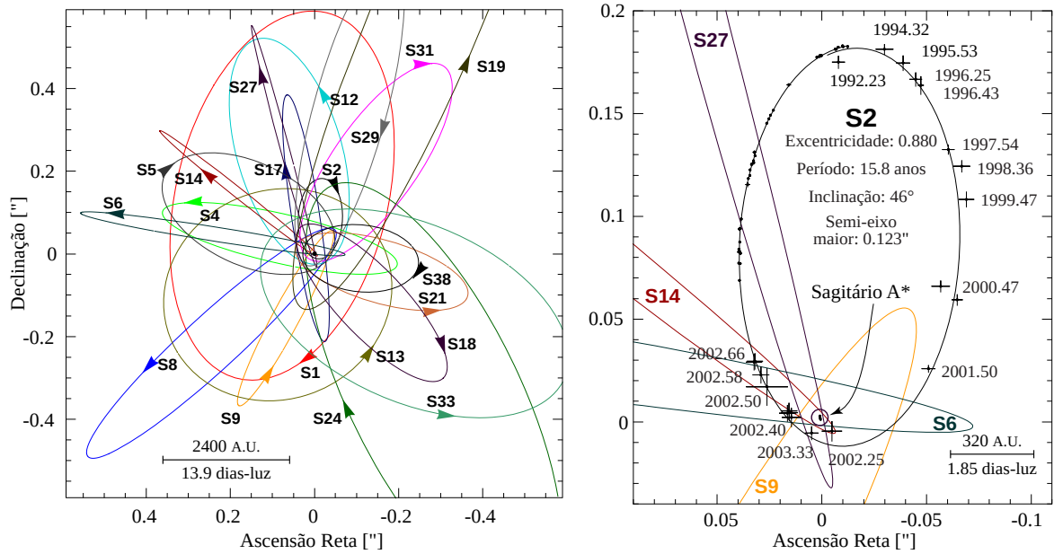
Figura 234: Distribuição das estrelas próximas do centro galáctico com destaque à órbita kepleriana da estrela S2 em torno de Sgr A* ( 17^{\text{h}}45^{\text{m}}39^{\text{s}}.95 , -29^{\circ}00'28''.2 , J2000). O pericentro está a cerca de 118 A.U. (tomando a distância de Sgr A* seja 8.0 kpc); os parâmetros orbitais implicam uma massa central de \approx 4 \times 10^6 M_{\odot} . O modelo mais aceito é de um buraco negro supermaciço central. Figuras tiradas de Schödel et al. (2002) ; Gillessen et al. (2009) .
