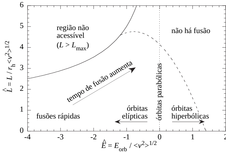
Figura 196: Critério de fusão de duas galáxias de massa comparável em função da energia orbital e momento angular iniciais normalizados. Órbitas no canto superior esquerdo não existem. Acima da linha tracejada a fusão pode ocorrer mas em um tempo muito elevado (maior que H_0^{-1} ). Figura tirada de Binney & Tremaine (1987) .
