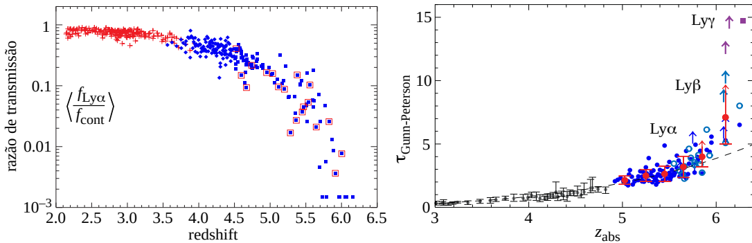
Figura 238: Esquerda: razão entre a transmissão do fluxo da linha Ly- \alpha e o contínuo adjacente em função do redshift medido em QSOs. Direita: profundidade óptica devido ao efeito Gunn-Peterson em função do redshift de absorção da linha Ly- \alpha . A linha tracejada corresponde a uma evolução passiva de \tau_{Ly} e os pontos por volta de z = 6 mostram a rápida evolução nesta época. Figuras tiradas de Songaila (2004) e Fan et al. (2006).
