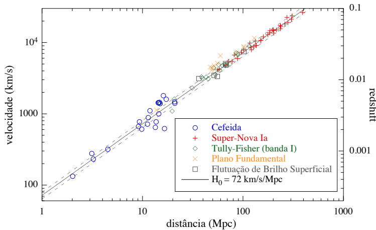
Figura 45: Resultado final do projeto chave do HST para medida da constante de Hubble. Compare este gráfico com o trabalho original de Hubble, Fig. 17. Figura baseada nos dados publicados em (Freedman et al., 2001). A incerteza em H_0 é de \pm 4 \text{ km s}^{-1} \text{ Mpc}^{-1} .
