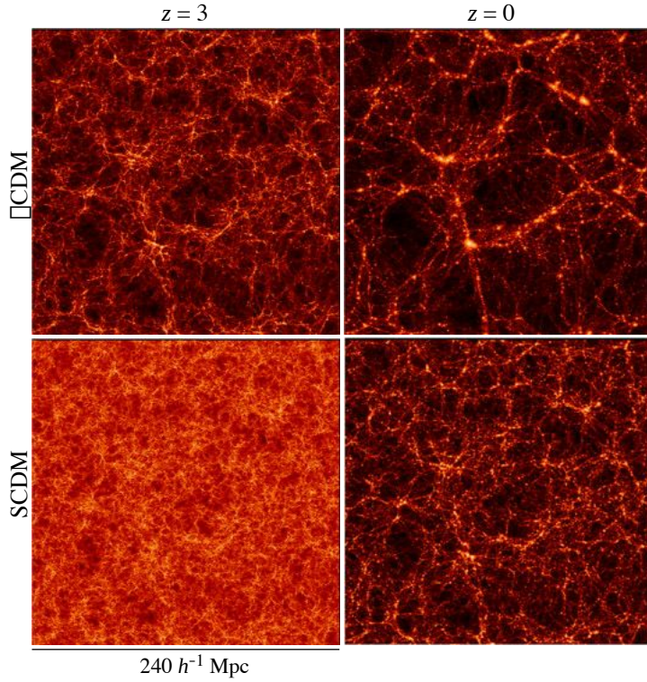
Figura 85: Simulação de dois cenários cosmológicos, \Lambda CDM ( \Omega_\Lambda = 0,7 , \Omega_M = 0,3 , h = 0,7 ) e SCDM ( \Omega_M = 1 , h = 0,5 ), mostrados na época atual ( z = 0 ) e em z = 3 . A profundidade da fatia do Universo nos painéis tem um décimo da largura. Cada simulação tem 256^3 partículas. Figura tirada de (Jenkins et al., 1998, Virgo Consortium ).
