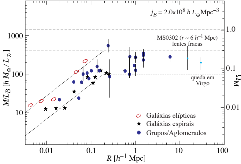
Figura 181: Razão massa–luminosidade na banda B em função da escala. O parâmetro de densidade, \Omega_M é obtido supondo a densidade de luminosidade média dada no canto superior direito. As medidas de aglomerados são no interior de 1,5 h^{-1} \text{Mpc} . Figura baseada em Bahcall et al. (2000).
