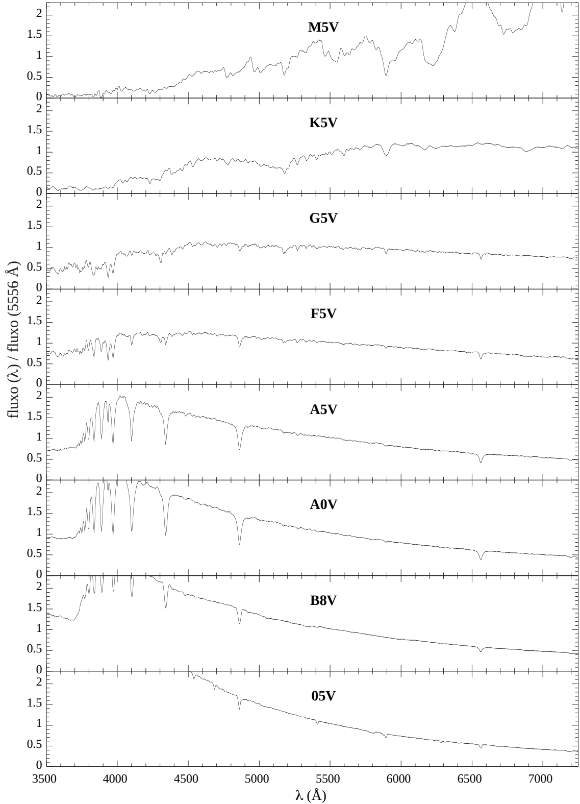
Figura 255: Espectro de estrelas da sequência principal do catálogo de Pickles (1998) .
