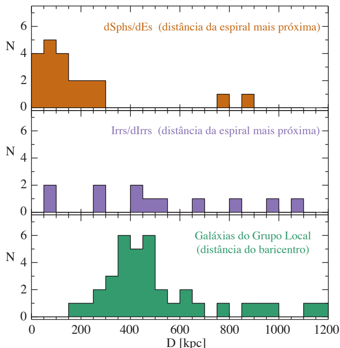
Figura 162: Distribuição das distâncias no Grupo Local (baseado em Grebel, 2000). As galáxias se agrupam em torno das galáxias dominantes e não em torno do baricentro.
