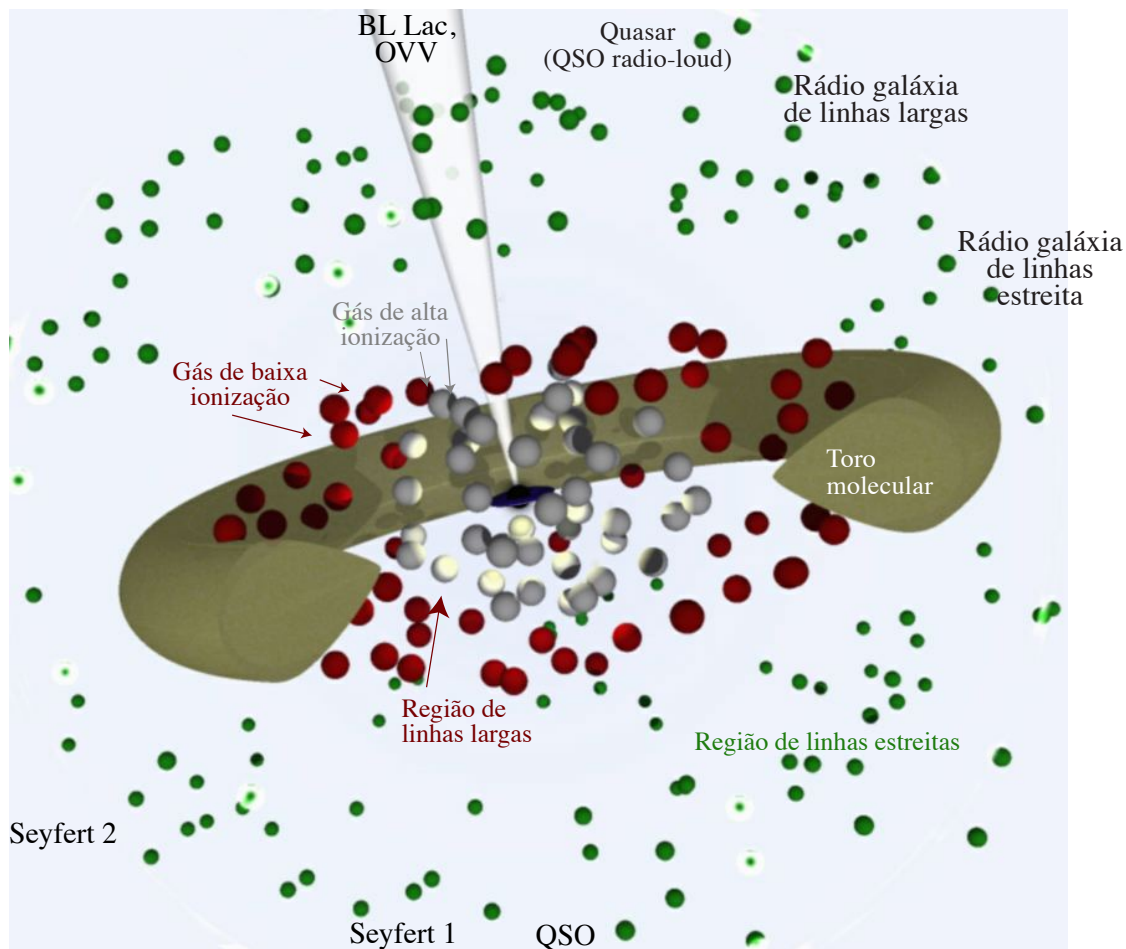
Figura 228: Modelo unificado de AGNs (fora de escala). No centro está o disco de acreção e o buraco negro. Dependendo da posição do observador, a AGN é classificada de maneira diferente. Em geral, se a região central pode ser observada temos uma AGN tipo 1; se a região central está escondida, temos uma AGN tipo 2. Para efeito de ilustração apenas um jato é mostrado (quando existem, os jatos são aproximadamente simétricos em relação ao núcleo).
