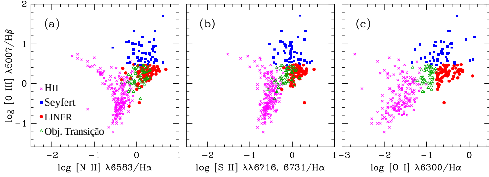
Figura 242: Diagnósticos de razões de linhas de emissão onde podemos distinguir galáxias star-burst (regiões HII), LINERs, “objetos de transição” e Seyferts (veja também Secs. 11.1 e 11.2). Figura tirada de Ho (2008).
