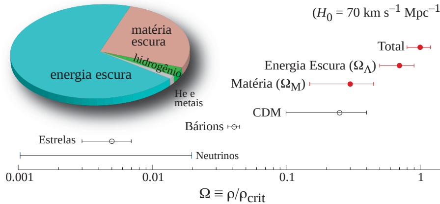
Figura 73: Composição do Universo, data em termos do parâmetro de densidade \Omega . Quando necessário, a constante de Hubble foi fixada no valor acima. A contribuição da CMB hoje é \Omega_{\text{CMB}} = 2,47 h^{-2} \times 10^{-5} . A contribuição do H I é \Omega_{\text{H I}} = (2,85 \pm 0,45) h^{-1} 10^{-4} .
