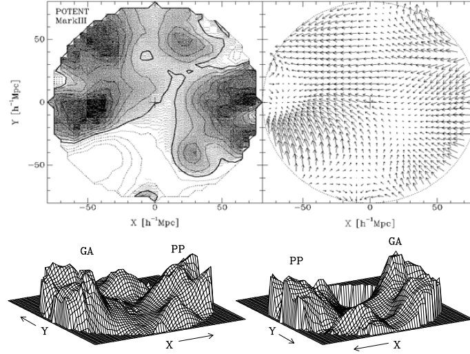
Figura 106: Distribuição de massa no Universo local pelo método POTENT. Abaixo, uma representação tridimensional. Os eixos correspondem às coordenadas supergalácticas. As siglas “GA” e “PP” correspondem ao Grande Atrator e ao super-aglomerado de Peixes-Perseus (compare com a figura 88). A Galáxia e o Grupo Local se encontram no centro destes gráficos. Figuras tiradas de (Dekel et al., 1999).
