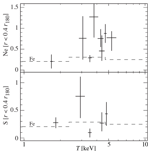
Figura 153: Abundância de neônio e enxofre em função da temperatura do aglomerado obtidas com satélite ASCA. Apesar das barras de erro, estes elementos são significativamente mais abundantes que o Fe (linha tracejada). Figura adaptada de Finoguenov et al. (2001) .
