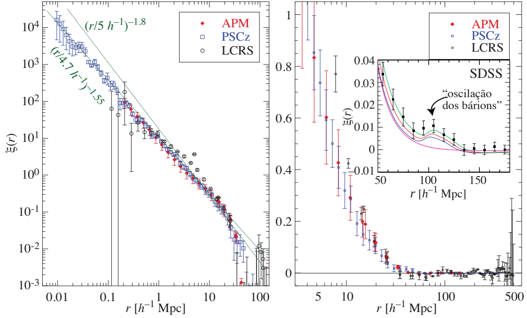
Figura 97: Função de correlação de galáxias. Esquerda: para pequenas escalas; Direita: grandes escalas. Três catálogos são utilizados: APM [a partir da deprojeção da distribuição 2D, (Baugh, 1996)]; PSCz [ Point Source Catalog , galáxias selecionadas no infravermelho com o satélite IRAS, (Hamilton & Tegmark, 2002)]; LCRS [ Las Campanas Redshift Survey , galáxias selecionadas no ótico, (Tucker et al., 1997)]. No destaque, a direita, dados do SDSS [galáxias vermelhas, luminosas (Eisenstein et al., 2005)]. A flecha mostra a escala onde é detectado a oscilação de bárions devido às flutuações de densidade primordial (veja Sec. 3.5).
