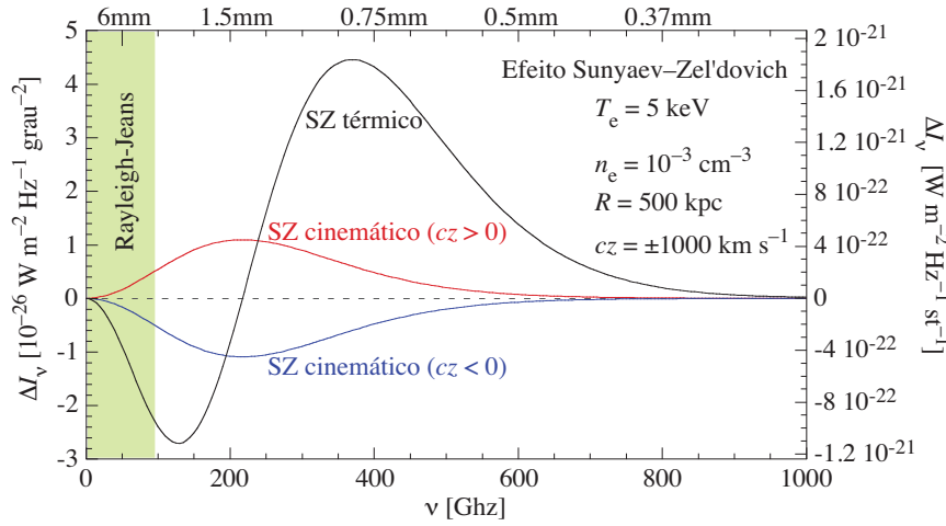
Figura 125: Variação da radiação cosmológica de fundo devido aos efeitos SZ térmico e cinemático. Note que para \nu = 215 GHz o efeito SZ térmico é nulo enquanto que o efeito SZ cinemático (em módulo) é máximo). Na parte Rayleigh-Jeans o efeito SZ térmico é sempre negativo.
