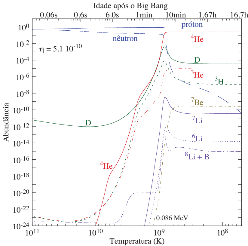
Figura 54: Evolução da abundância (em massa para o ^4\text{He} , numérica para os demais elementos, em relação ao hidrogênio) dos núcleos formados em função da idade e temperatura do Universo, para \Omega_B h^2 = 0,019 . O ^7\text{Be} é instável e decai com meia-vida de 53,3 dias principalmente em ^7\text{Li} ; o ^8\text{Li} é instável com meia-vida de 0,84 s. O boro corresponde à soma dos isótopos ^{10}\text{B} e ^{11}\text{B} . Figura baseada em Tytler et al. (2000) .
