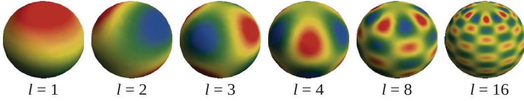
Figura 58: Harmônicos esféricos, \sum_{m=-l}^l Y_l^m(\theta, \phi) , sobre uma esfera. A escala de cores vai de vermelho (quente) a azul escuro (frio). Neste exemplo, usamos sempre a mesma fase.
