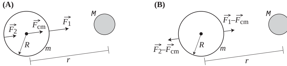
Figura 194: A força de maré, F_M ocorre em corpos extensos devido à diferença da força gravitacional entre os pontos próximos e distantes do corpo perturbador de massa \mathcal{M} a distância r .
