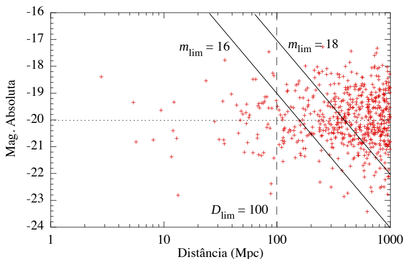
Figura 110: Ilustração do viés de Malmquist. Aqui supomos uma distribuição espacial homogênea de galáxias que seguem uma distribuição de luminosidade gaussiana, com magnitude absoluta média -20 e desvio padrão igual a 1. As galáxias selecionáveis estão abaixo das curvas de magnitude aparente constante (limite observacional), ou a esquerda do traço vertical (limite em distância).
