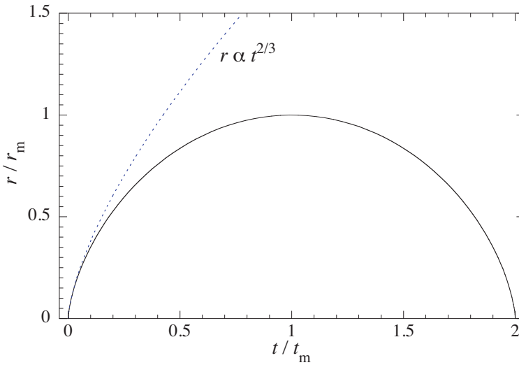
Figura 168: Evolução do modelo Top-Hat (linha contínua). Em pontilhado, a aproximação linear ( t \ll t_m ).
