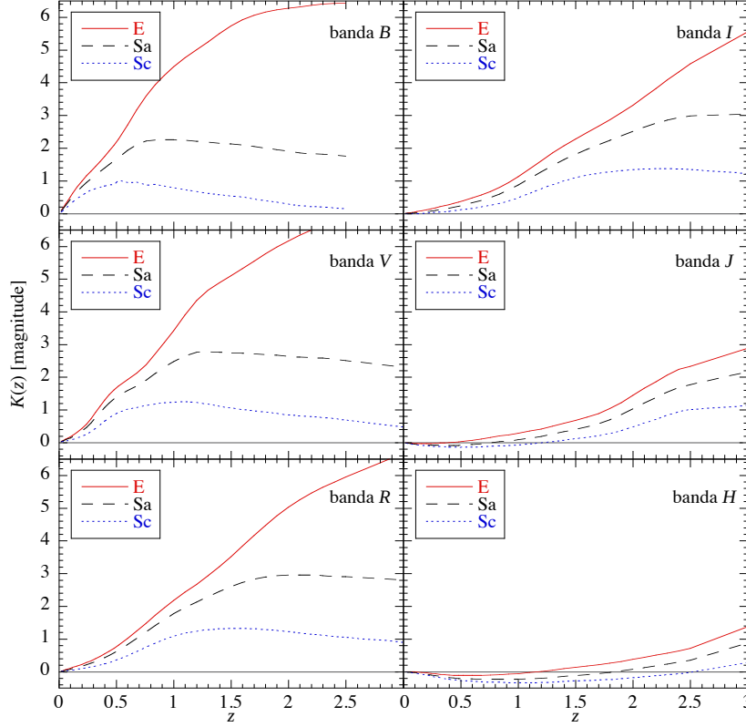
Figura 33: Correção K [Eq. (55)] para galáxias elípticas (E), e espirais (Sa e Sc) para diversos filtros do sistema Johnson estendido. Baseado em dados de Poggianti (1997).
