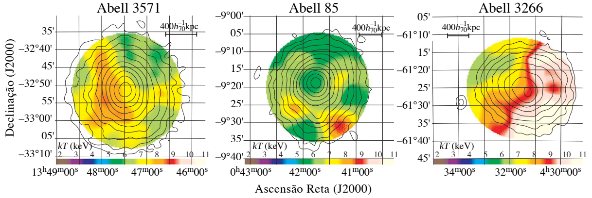
Figura 122: Mapas de temperatura (imagens coloridas, escala em keV) de três aglomerados ricos obtidas com o satélite ASCA. As curvas de nível superpostas representam a intensidade da emissão em raios-X. Podemos notar as estruturas complexas em temperatura, indicando processos dinâmicos (fusões) ou resfriamento do gás (p.ex., região central de Abell 85). Figura tirada de Donnelly et al. (2003) .
