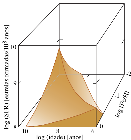
Figura 200: Evolução da taxa de formação estelar (SFR) na Via Láctea. O eixo horizontal representa a idade das estrelas, o eixo diagonal representa a metalicidade (em termos da abundância de ferro em relação à abundância solar) e o eixo vertical, a taxa de formação estelar. Atualmente, a SFR da Via Láctea é estimada em 1,65 \pm 0,20 M_\odot/\text{ano} (Licquia & Newman, 2015).
