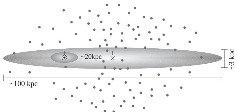
Figura 11: Modelo de Universo de Shapley (1918) . Os pequenos círculos cinza são aglomerados globulares. No modelo de Shapley, a região próxima do Sol tem um excesso de densidade. O “X” indica o centro da Galáxia e “ \odot ” a posição do Sol. Note a diferença de escala entre os modelos de Shapley e Kapteyn.
