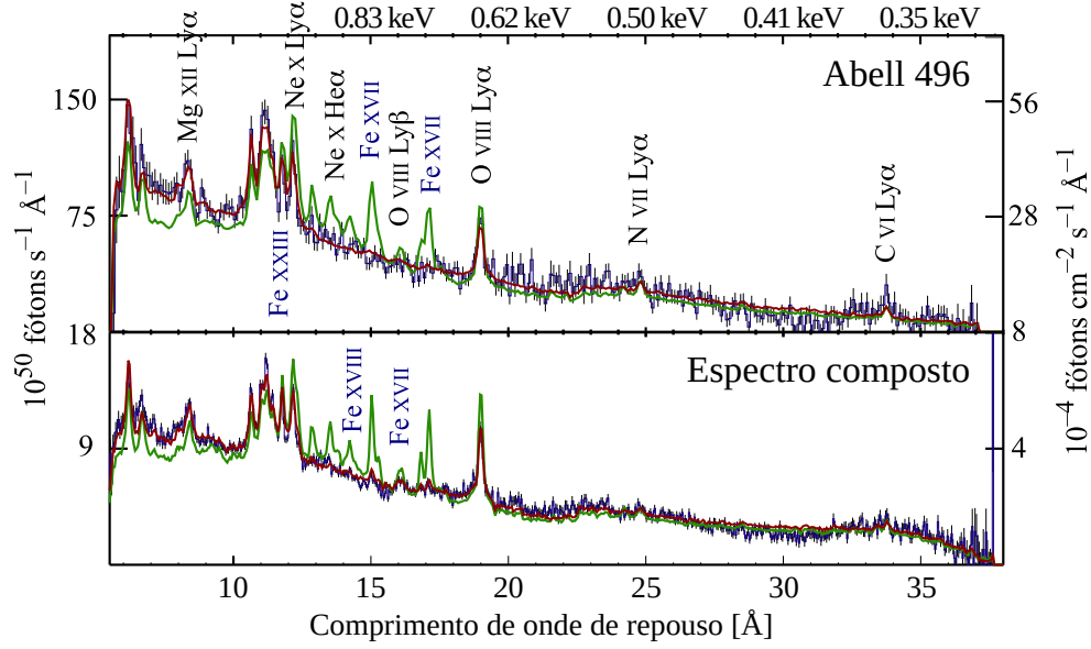
Figura 139: Espectro de alta resolução do detector RGS do XMM-Newton comparado ao espectro previsto pelo cenário clássico de “cooling-flow” (linha verde). A linha vermelha representa um modelo empírico onde o gás não é tão frio ( kT \gtrsim 1 keV). O painel de cima mostra a observação de um aglomerado e o painel de baixo a composição de várias observações. Figura baseada em Peterson et al. (2003) .
