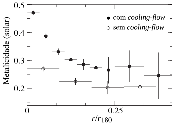
Figura 151: Gradiente de metalicidade em aglomerados ricos com e sem cooling-flow obtidos com satélite BeppoSAX. A distância radial é dada em termos de r_{180} \approx R_{\text{virial}} (cf. seção 8.1). Figura tirada de De Grandi & Molendi (2001)
