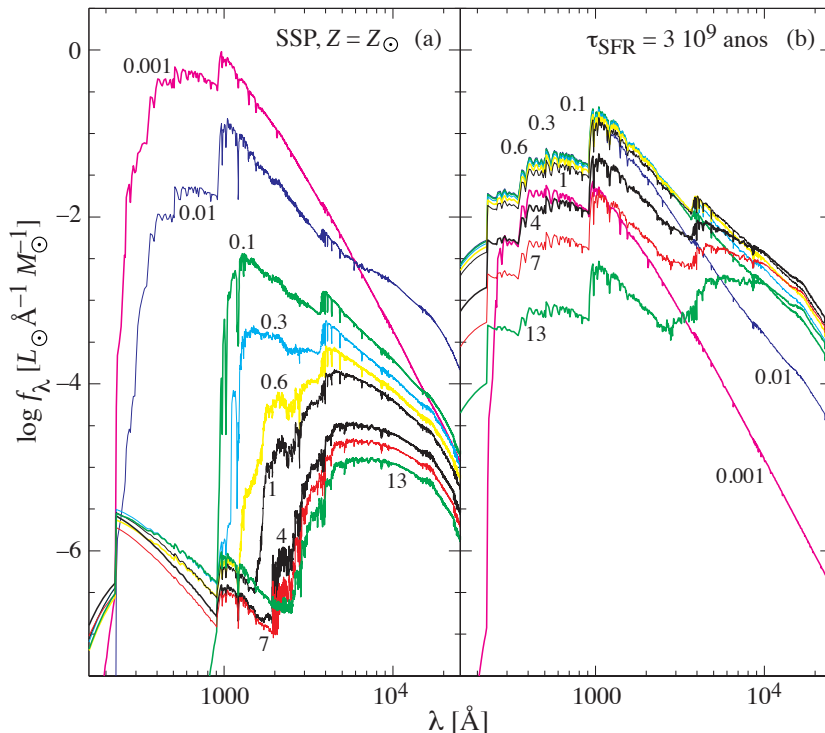
Figura 199: Evolução da distribuição espectral de energia (SED). (a) Evolução passiva de uma população estelar formada instantaneamente em t = 0 . (b) Evolução passiva de uma população estelar com taxa de formação estelar exponencial, \Psi(t) = \exp(-t/\tau_{\text{SFR}}) . No painel da direita, o fluxo F_\lambda está multiplicado por 100. (Figura tirada de Bruzual, 2001 )
