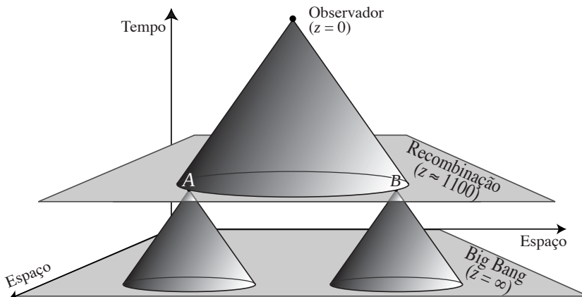
Figura 49: Problema do horizonte no modelo cosmológico pré-inflacionário: Em z = 0 observamos dois pontos A e B que estão no interior do nosso cone de luz passado. Contudo, como não há intersecção entre os cones de luz passados de A e B, estes pontos não estão casualmente conectados.
