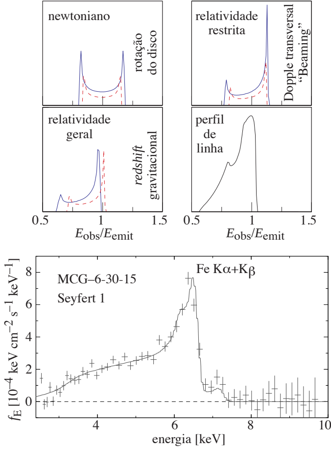
Figura 229: Perfil da linha K do ferro ( E \approx 6,4 keV) produzida em um disco de acreção de AGN. Esta linha é alargada pela rotação e efeitos relativísticos: efeito Doppler transversal, “beaming” e redshift gravitacional. A linha contínua (azul) ilustra a emissão mais próxima do buraco negro, \sim 6r_s – o raio mais interno onde há órbitas estáveis no caso de um BN de Kerr (em rotação); a linha tracejada (vermelha) corresponde à emissão mais distante ( \sim 30r_s ). Abaixo a observação pelo satélite XMM-Newton da linha do Fe K em uma Seyfert tipo 1. Figura baseada em Fabian et al. (2000, 2002).
