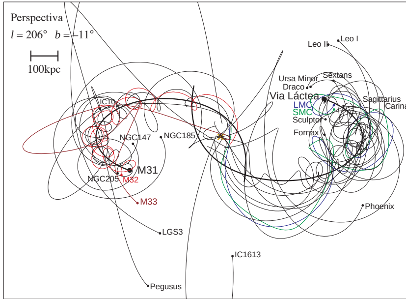
Figura 163: Uma das inúmeras possibilidades de trajetórias das galáxias do Grupo Local. As órbitas da Via Láctea e M31 são praticamente elipses com o baricentro do Grupo Local em um dos focos. Cada uma destas galáxias é seguida por seu cortejo de galáxias anãs. Figura tirada de Sawa & Fugimoto (2005).
