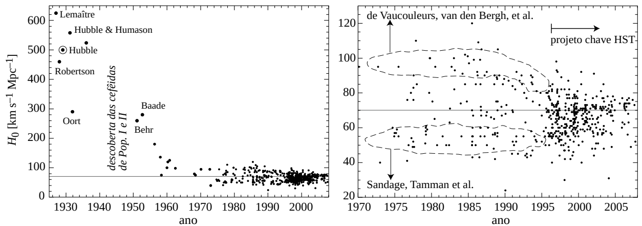
Figura 15: Evolução histórica da determinação da constante de Hubble. Baseado na compilação feita por John Huchra, cfa-www.harvard.edu/~huchra/hubble , como parte do “projeto chave” do HST. Note que a primeira medida é de Georges Lemaître.
