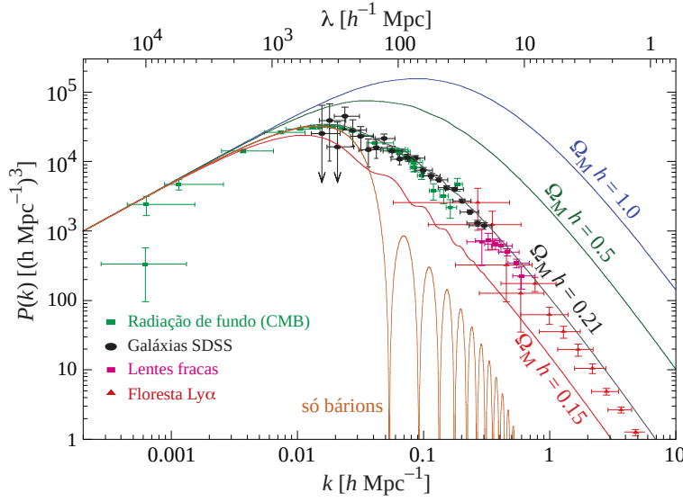
Figura 78: A forma do espectro de potência depende do parâmetro \Gamma = \Omega_M h . Os espectros estão normalizados na escala da CMB e, para comparação, temos o espectro de potência de um universo puramente bariônico com \Omega_B = 0,3 .
