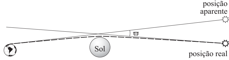
Figura 129: Desvio gravitacional da trajetória de um raio luminoso que passa próximo do Sol. O ângulo de desvio, \varpi calculado de forma Newtoniana, neste caso rasante, é de \varpi = 2GM_{\odot}/(c^2 R_{\odot}) = 0,876'' . A linha tracejada espessa representa a trajetória (geodésica) da luz.
