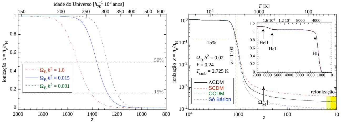
Figura 26: Esquerda: Taxa de ionização em função do redshift e da idade do Universo ( q_0 = 1/2 ) para diferentes valores de \Omega_B h^2 , utilizando a aproximação Y = 0 . Direita: Taxa de ionização utilizando modelo mais realista incluindo o He (calculado com o código recfast ) para diversos modelos cosmológicos. Note que os modelos OCDM e \Lambda CDM são praticamente indistinguíveis. Nesta figura, não levamos em conta a reionização do Universo a partir de z \approx 15 (veja seção 12).
