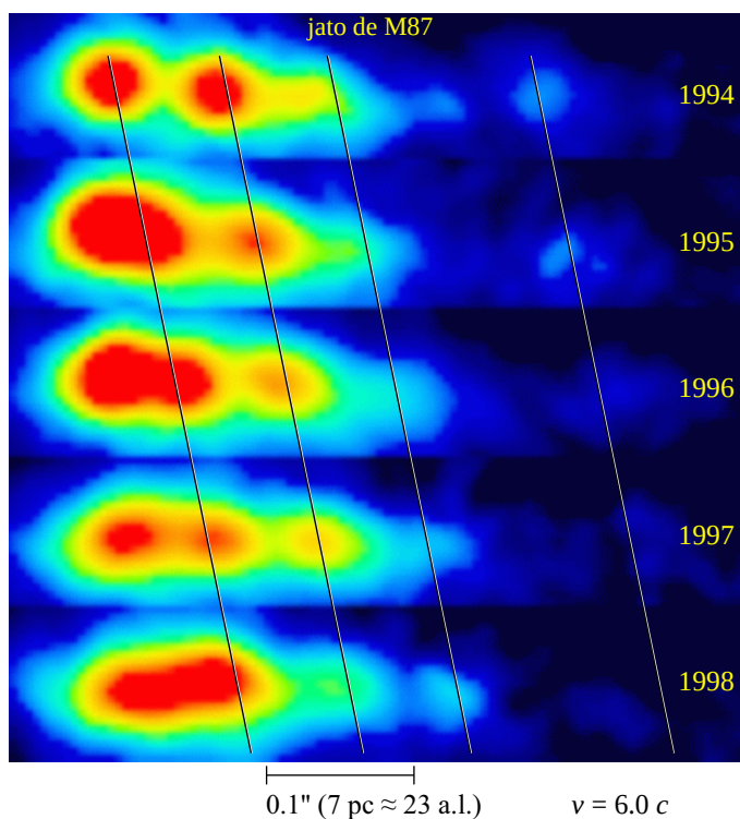
Figura 215: Movimento aparente no jato óptico de M87. As linhas diagonais correspondem a um movimento aparente uniforme no plano do céu de 6 vezes a velocidade da luz! As imagens foram produzidas por John Birretta, do Space Telescope Science Institute .
