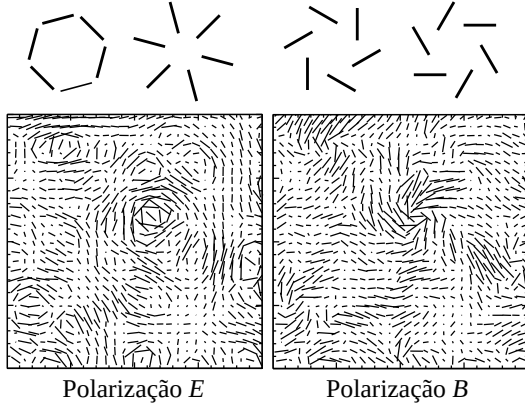
Figura 66: Aparência do padrão de polarização para os modos E (divergente) e B (rotacional) esperados na CMB. O nível de polarização das anisotropias é < 10\% . Figura tirada de (Hu & White, 1997; Kaplan et al., 2003).
