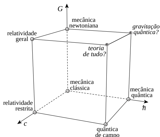
Figura 261: “Cubo da Física”. As teorias de gravitação quântica e “teoria de tudo” ainda precisam ser inventadas. Os eixos são a constante da gravitação, G , velocidade da luz, c , e constante de Planck, \hbar . Figura tirada do site de James Schombert, abyss.uoregon.edu/~js .
