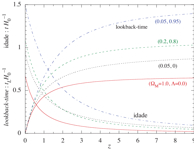
Figura 41: Idade e lookback-time do Universo para algumas combinações de \Omega_M e \Omega_\Lambda . Para cada modelo, as curvas se cruzam quando o Universo tem metade da idade atual.
