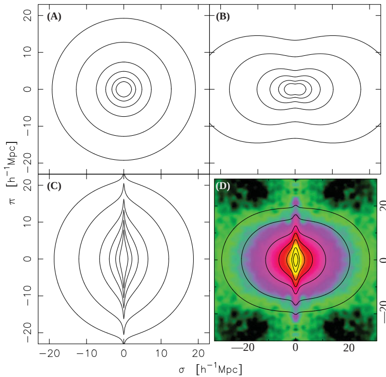
Figura 104: Função de correlação em 2 dimensões. (A) modelo sem distorção de velocidades peculiares. (B) modelo apenas com distorções devido à queda coerente em grandes estruturas (efeito Kaiser). (C) modelo com distorções devido ao movimento aleatório em poços de potencial gravitacional ( \sqrt{v^2} = 500 \text{ km s}^{-1} ). Modelos tirado de Hawkins et al. (2003). (D) Função de correlação de duas dimensões no espaço de redshift obtida com o catálogo 2dFGRS. A função é obtida no primeiro quadrante e reproduzida nos demais por reflexão. Os contornos ( \xi = 10, 5, 2, 1, 0.5, 0.2 e 0.1 ) correspondem a um modelo cosmológico com \beta = 0.4 . Figura tirada de Peacock et al. (2001).
