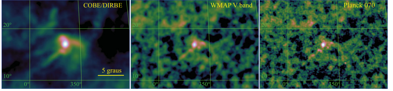
Figura 24: Comparação entre os satélites COBE de 1990, WMAP de 2001 e Planck de 2009 (ano de lançamento), mostrando o ganho em resolução angular. Os dados do COBE correspondem a 4 anos de observação, os do WMAP a 9 anos, e para o Planck é 1 ano e meio.
