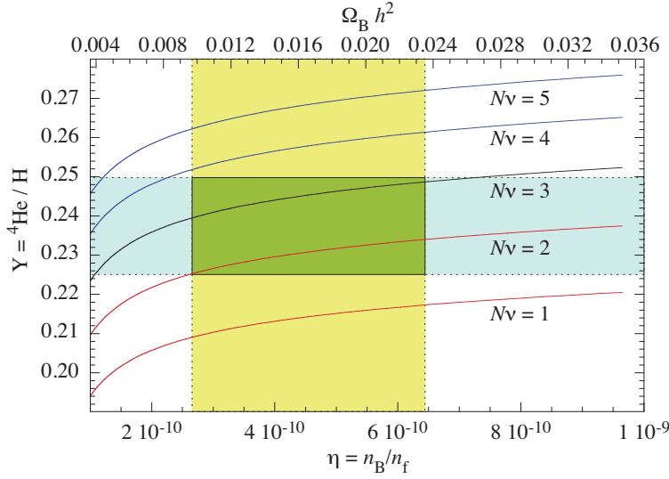
Figura 57: Dependência da abundância primordial de Hélio-4 em função do número de famílias de neutrinos (léptons), N_\nu . A banda horizontal dá os limites observacionais de abundância do ^4\text{He} ; a banda vertical dá os limites da fração de bárions.
