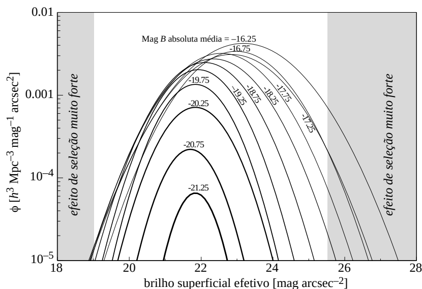
Figura 252: Distribuição do brilho superficial de galáxias para diversos intervalos de luminosidade total (em magnitude absoluta na banda B ). As galáxias menos luminosas apresentam tendência de terem maior dispersão, isto é, podem ter brilho superficial muito baixo ou alto. Figura baseada em Driver et al. (2005).
