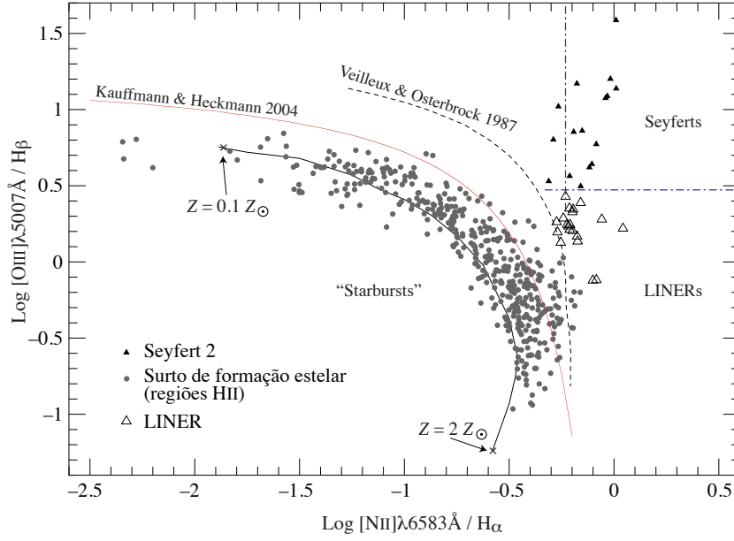
Figura 241: Diagrama BPT de linhas de emissão para distinguir AGNs de regiões HII (formação estelar intensa). A linha contínua representa regiões HII de diferentes metalidades segundo Dopita & Evans (1986). A linha tracejada separa AGNs de regiões de formação estelar segundo Veilleux & Osterbrock (1987). Figura tirada de Gronwall et al. (2002).
