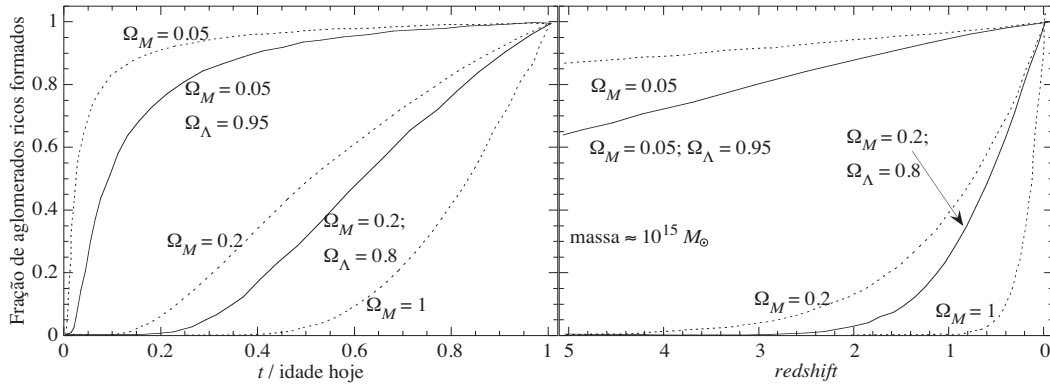
Figura 118: Estimativa da fração de aglomerados de 10^{15} M_{\odot} formados, normalizada ao número de aglomerados já relaxados. As observações sugerem \Omega_M \sim 0,2-0,5 , dando poucos vínculos à \Omega_{\Lambda} . Figura tirada de Richstone, Loeb & Turner (1992).
