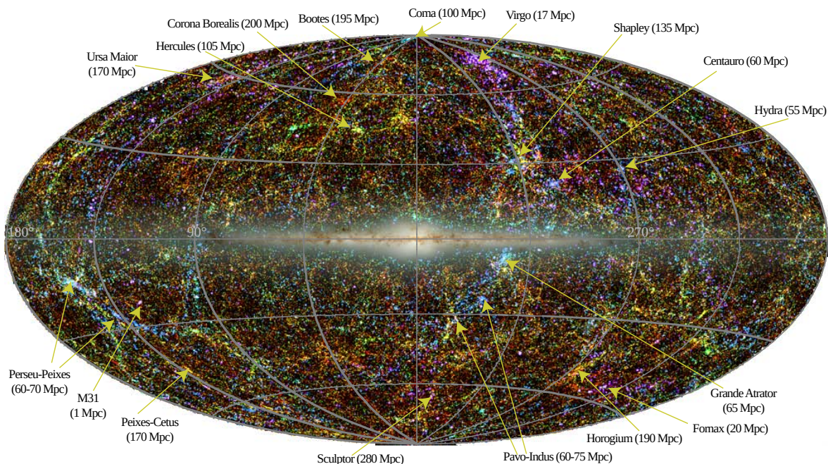
Figura 90: Estrutura em grande escala vista pelo 2MASS, em uma projeção de áreas iguais (Hammer-Aitoff) em coordenadas Galácticas. As cores representam diferentes intervalos de redshift. As distâncias de algumas estruturas estão indicadas entre parênteses. Figura original criada por T. Jarrett (IPAC/Caltech); veja também Jarrett et al. (2004).
