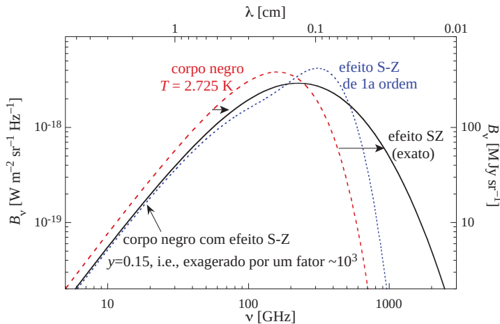
Figura 124: Distorção do espectro de corpo negro da radiação cósmica de fundo (tracejada) devido ao efeito Sunyaev–Zel’dovich (linha contínua, cálculo exato; linha pontilhada, 1ª ordem). Para frequências inferiores a \sim 210 GHz, há uma diminuição aparente da temperatura da CMB
