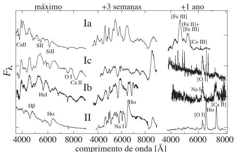
Figura 258: Tipos de supernova segundo o tipo de espectro próximo do máximo de luminosidade, após 3 semanas e 12 meses depois (Cappellaro & Turatto, 2000).
