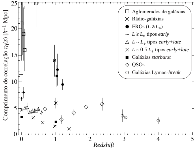
Figura 101: Comprimento de correlação para diversos objetos em função do redshift . Figura tirada de Overzier et al. (2003).
