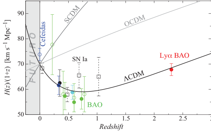
Figura 48: Determinação da evolução do parâmetro de Hubble, H(z) . Os cenários cosmológicos representados pelas linhas cheias estão normalizados em H_0 = 70 \text{ km s}^{-1} \text{ Mpc}^{-1} . Figura baseada em Busca et al. (2013).
