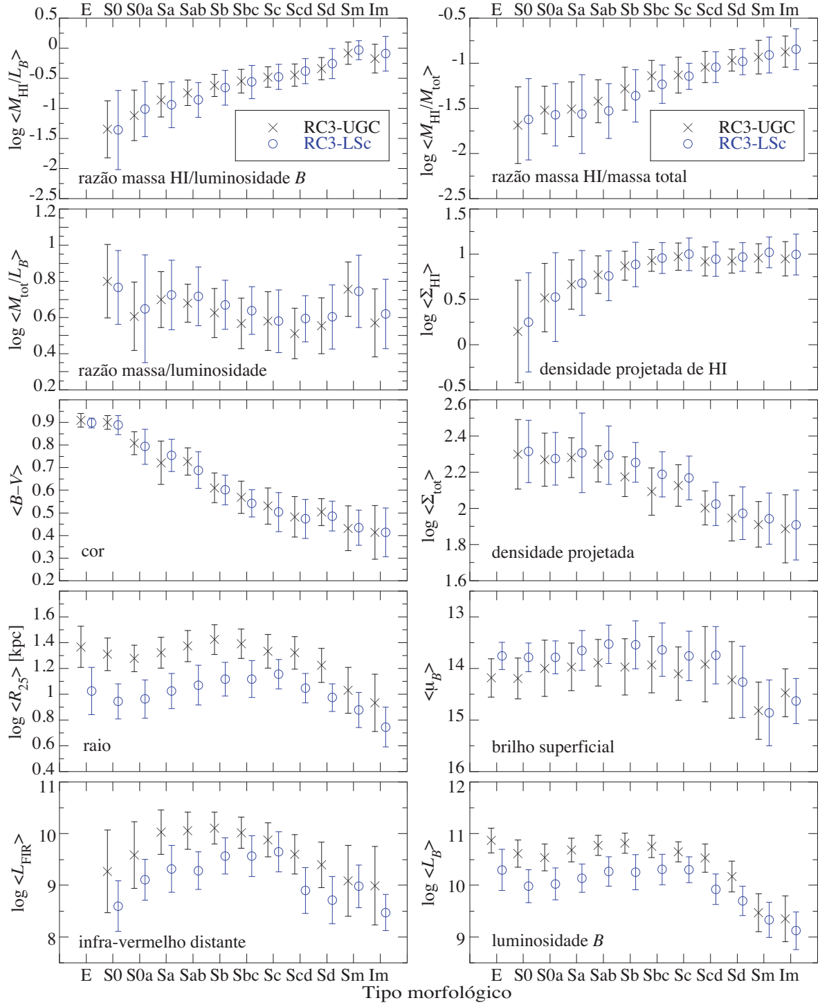
Figura 245: Propriedades físicas de galáxias ao longo da sequência de Hubble. As unidades de massa e luminosidade são solares. Dados tirados de Roberts & Haynes (1994) , utilizando \sim 8000 galáxias.
