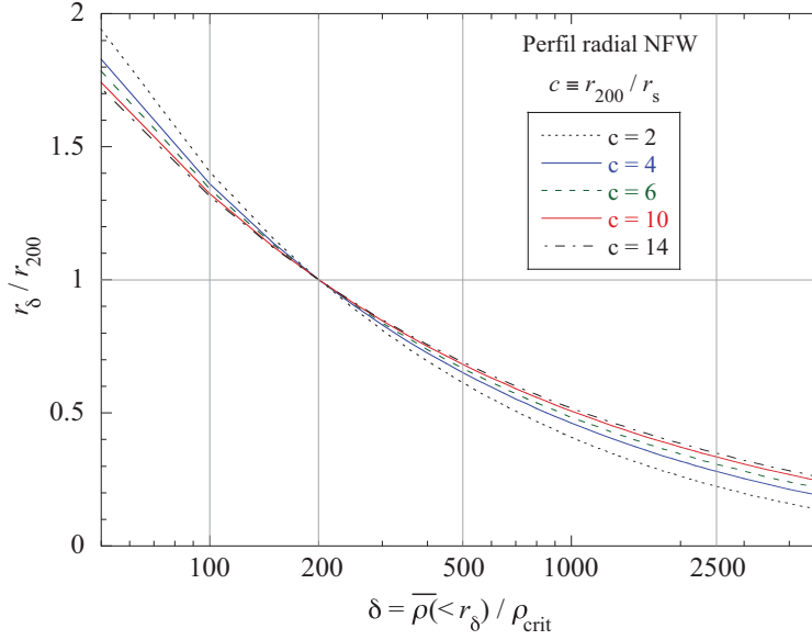
Figura 81: Relação entre r_\delta e \delta para diferentes valores de concentração c do perfil de NFW. Alguns raios encontrados frequentemente na literatura estão em destaque.
