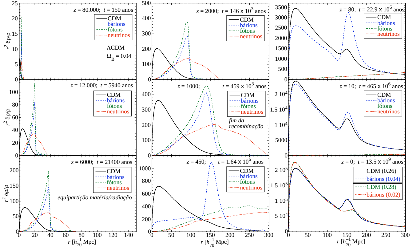
Figura 82: Evolução de uma perturbação, \delta\rho/\bar{\rho} em função do tempo da matéria escura fria (CDM), bárions, fótons e neutrinos sem massa. A área sob cada curva representa a massa contida na perturbação relativa à massa \bar{\rho}V , no mesmo volume da perturbação. A escala espacial (em unidades comóveis) na primeira coluna é metade das outras duas colunas e a escala de densidade aumenta com o tempo. Estas curvas foram calculadas usando a aproximação linear de crescimento de perturbações para o modelo \Lambda CDM, h = 0,7 e \Omega_B = 0,04 (exceto no último painel onde também está ilustrado o caso \Omega_B = 0,02 ). Figuras baseadas em (Eisenstein, Seo & White, 2007) e no texto de D. Eisenstein em cmb.as.arizona.edu/~eisenste/acousticpeak .
