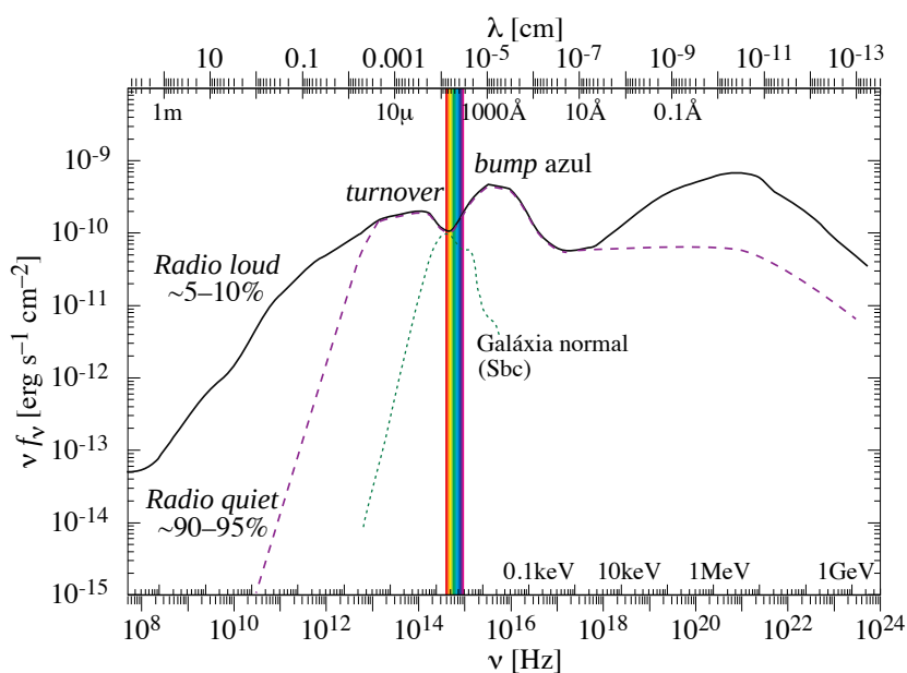
Figura 209: Contínuo típico de AGNs. Os traços contínuo e tracejado representam as “radio-louds” e as “radio-quiets”, respectivamente. Em pontilhado, o contínuo típico de uma galáxia normal (tipo Sbc). Figura baseada em Peterson (1997) .
