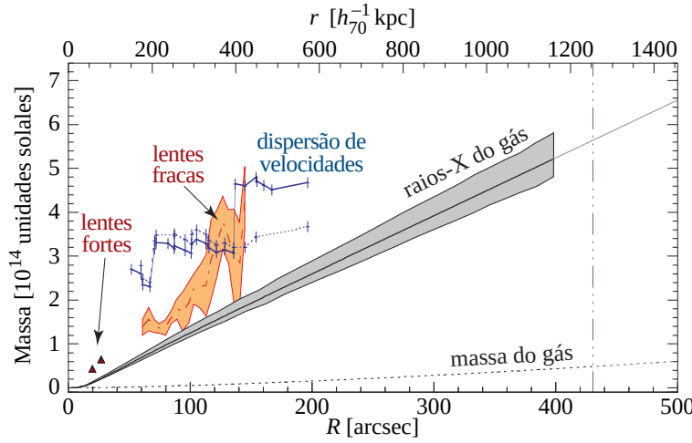
Figura 137: Perfis de massa para o aglomerado Abell 586 estimados por diversas técnicas. A reta vertical indica o raio do virial (definido na Sec 8.1). As estimativas concordam com uma diferença inferior a um fator 2. Figura baseada em Cypriano (2005) .
