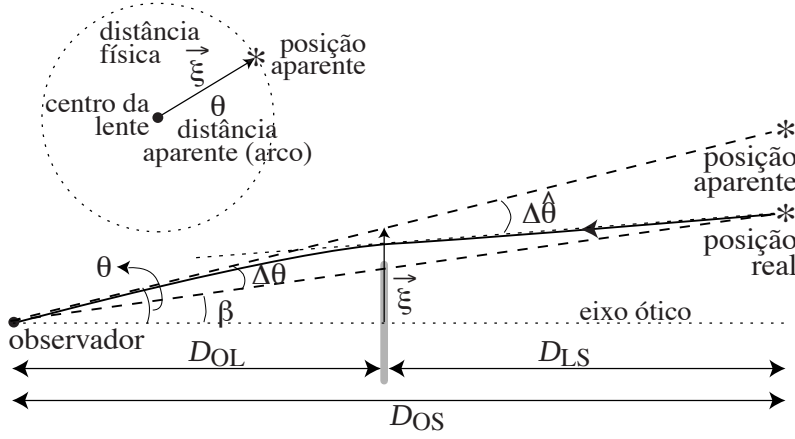
Figura 130: Desvio gravitacional da luz devido a presença de um corpo maciço (lente). O astro é observado em uma posição aparente \theta , distante \Delta\theta da posição verdadeira ( \beta ). A distância \xi medida no plano da lente entre o eixo ótico e a trajetória não perturbada do raio de luz é o parâmetro de impacto.
