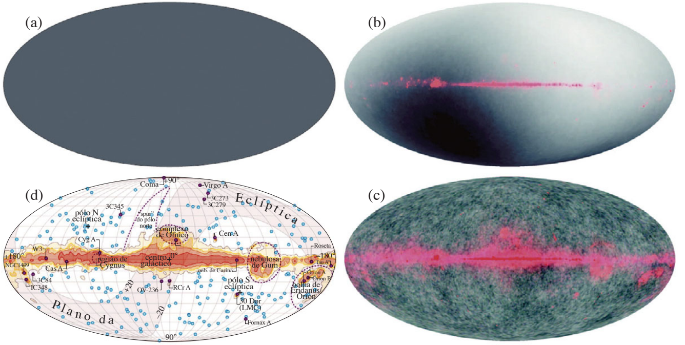
Figura 21: Imagem (em escala de temperatura) da radiação de fundo em todo o céu. (a): a temperatura medida diretamente em todo o céu: ela é realmente assim! (b): subtraindo a temperatura média, a componente de dipolo é colocada em evidência, indicando o movimento da Sistema Solar em relação à CMB. A variação máxima de temperatura do dipolo é de \Delta T/T \approx 10^{-3} . A emissão da Via Láctea está representada em outra escala de cor. (c): subtraindo a componente de dipolo, resta as flutuações devido à anisotropia da radiação de fundo e a imagem da Via Láctea em microondas se torna evidente. (d): diagrama com os principais objetos vistos em microondas e infravermelho distante. Figura baseada em Bennett et al. (2003) .
