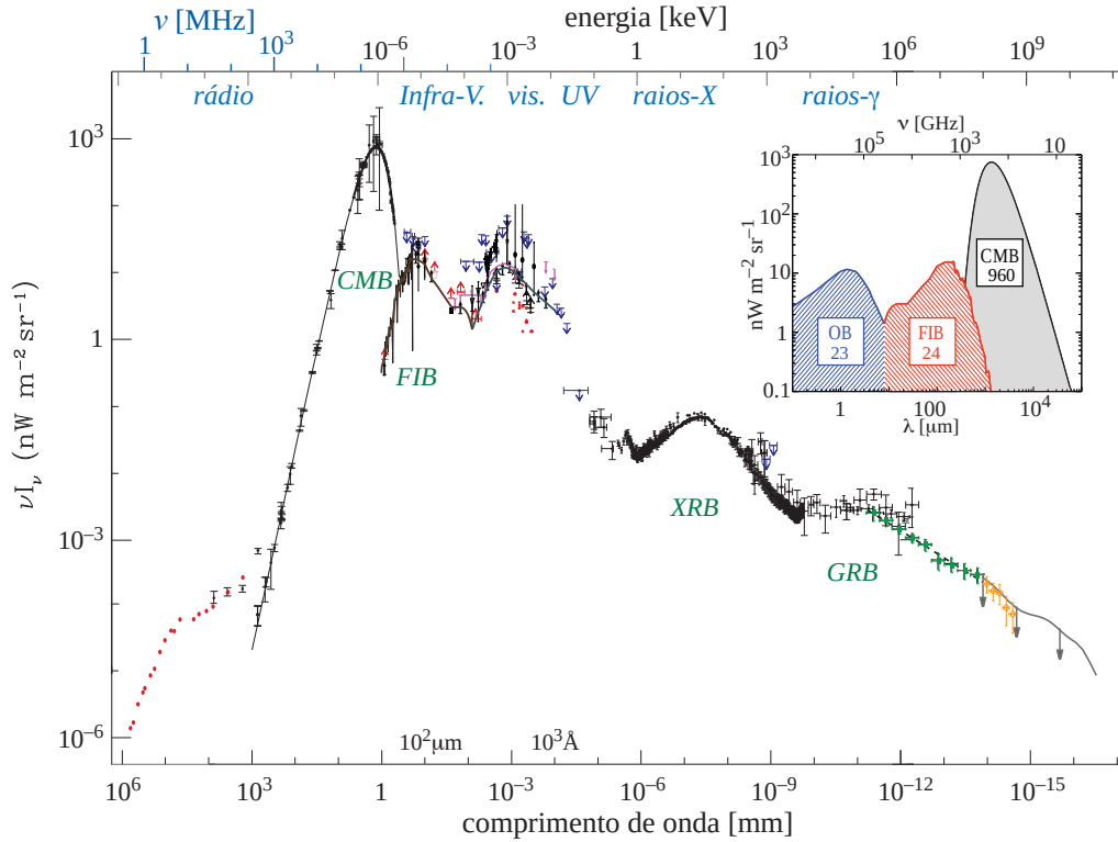
Figura 27: Distribuição espectral de energia da radiação de fundo. Note que a CMB é a maior contribuição em energia (Scott, 2000). No painel a direita, está ilustrada de forma esquemática as contribuições dos fundos óptico (OB), infravermelho (FIB) e micro-ondas (CMB) com suas respectivas contribuições em \text{nW m}^{-2} \text{sr}^{-1} .
