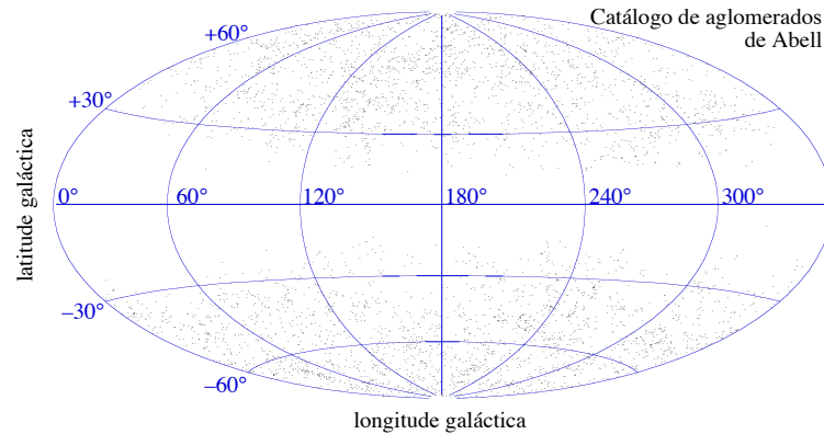
Figura 114: Distribuição dos aglomerados do catálogo de Abell (4076 objetos) em coordenadas galácticas.
