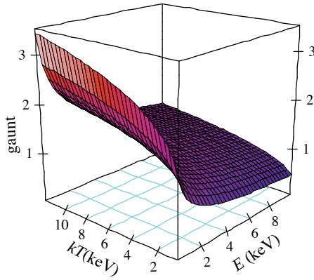
Figura 120: Fator de gaunt para energias e temperaturas características de aglomerados de galáxias calculado segundo a aproximação analítica de Itoh et al. (2002). Para cálculos de ordem de grandeza, podemos tomar em geral g(E, T) \sim 1,2 .
