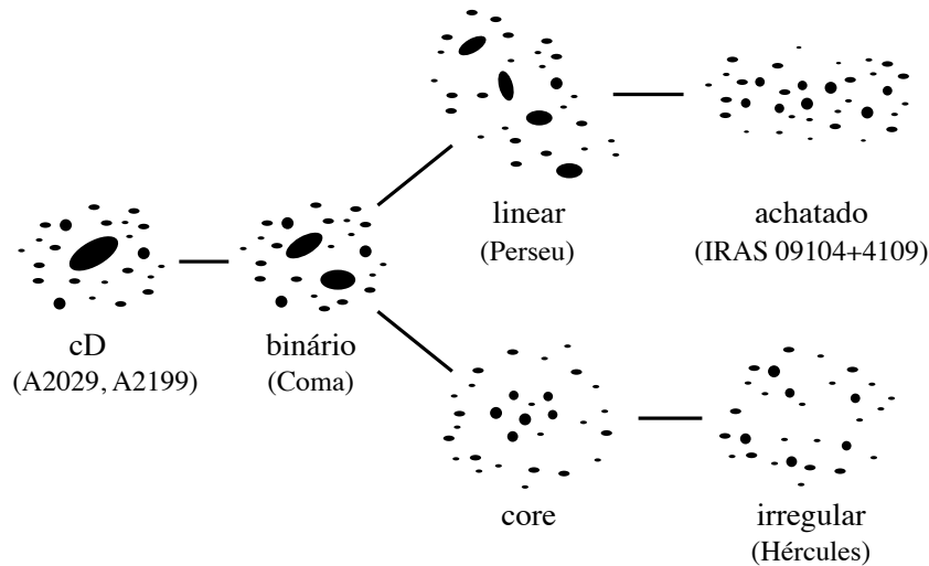
Figura 116: Sistema de classificação de Rood & Sastry.
