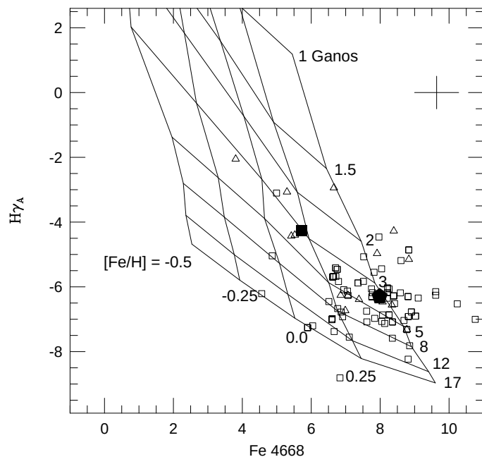
Figura 202: Diagrama idade-metalicidade de galáxias elípticas (quadrados) e S0 (triângulos). As intensidades das linhas H_\gamma e Fe 4668 são indicadores de idade e metalicidade, respectivamente. A grade representa o modelo de Worthey (1994) .
