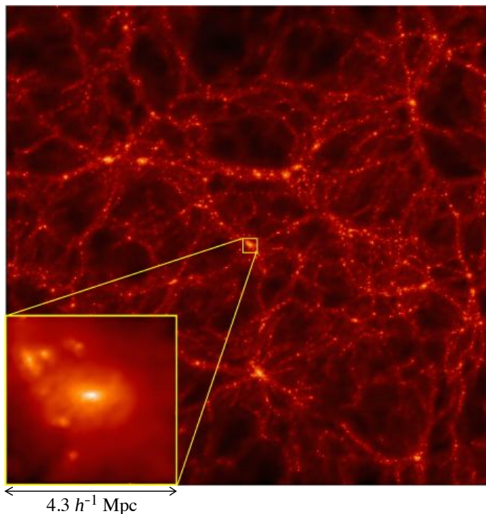
Figura 113: Fatia do Universo de uma simulação de um cenário \Lambda CDM em z = 0 . No detalhe, uma estrutura semelhante a um aglomerado rico, recém colapsado (note as sub-estruturas), na intersecção de dois filamentos. Figura tirada de (Kay, 2000, – Virgo Consortium ).
