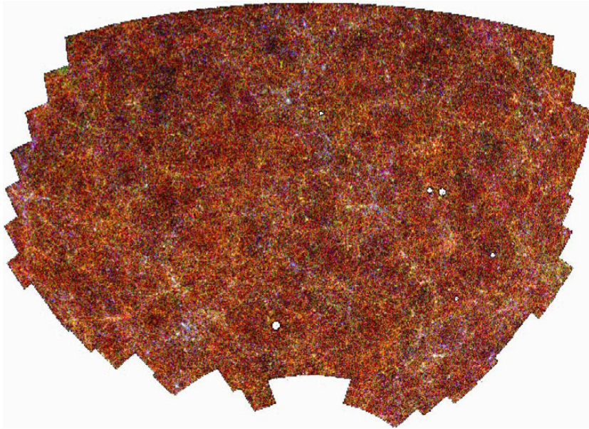
Figura 89: Projeção Hammer-Aitoff (área igual) de cerca de 3 milhões de galáxias ao redor do pólo sul galáctico ( 5^h < \alpha < 21^h , -72^\circ < \delta < -18^\circ ), obtido pelo APM galaxy survey (Maddox et al., 1990). As galáxias têm magnitude aparente entre 17 \leq b_J \leq 20.5 (as mais fracas estão representadas em vermelho, as intermediárias em verde e as mais brilhantes em azul).
