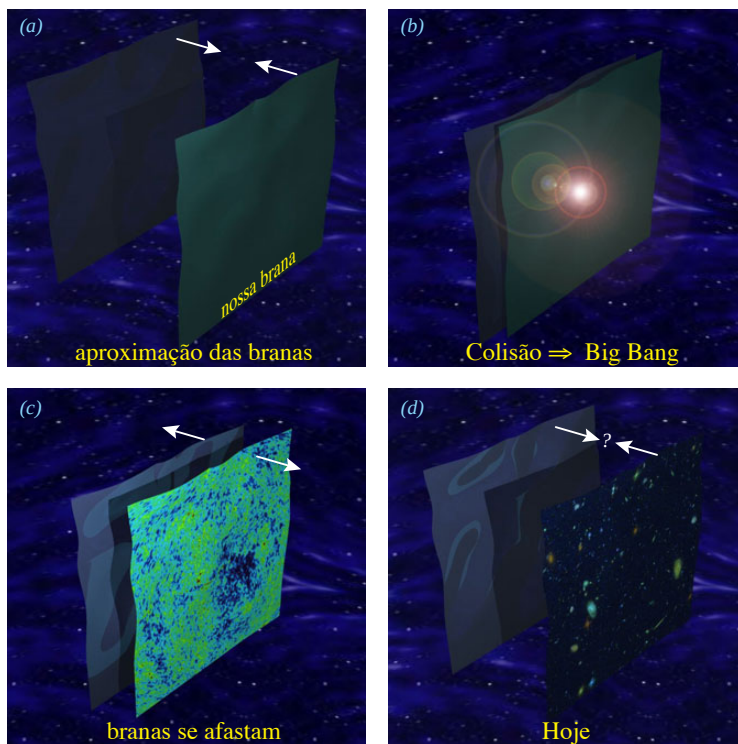
Figura 67: Cenário pré-Big Bang de Branas. Nosso Universo se encontra confinado em uma brana com três dimensões espaciais que se aproxima de outra brana (a). Quando colidem (b) ocorre o que chamamos de Big Bang. As branas se afastam (c) e, eventualmente as estrelas e galáxias se formam (d). No cenário ekpirótico as branas voltam a se aproximar quando a energia escura começa a predominar.
