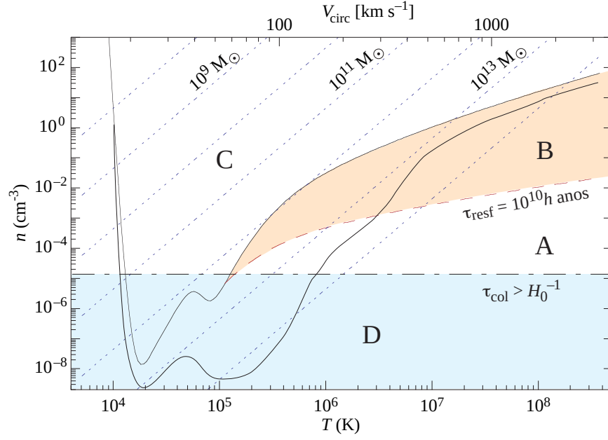
Figura 173: Diagrama densidade-temperatura do resfriamento do gás em um halo de matéria escura. O traço contínuo espesso representa os pontos onde \tau_{\text{resf}} = \tau_{\text{col}} de um gás primordial ( Y = 0,24 ); o traço fino, um gás com metalicidade solar. Nas regiões A e B, \tau_{\text{resf}} > \tau_{\text{col}} , na região C, \tau_{\text{resf}} < \tau_{\text{col}} . Na região B, \tau_{\text{resf}} < 10^{10} h anos. As linhas tracejadas diagonais correspondem à massa (total) de Jeans constante, de 10^6 a 10^{12} M_{\odot} . Halos de massa \mathcal{M} e densidade n devem se encontrar próximos às linhas de M_{\text{Jeans}} constante para estarem em equilíbrio hidrodinâmico. A linha horizontal (traço-ponto) representa 5,5 vezes a densidade crítica: nuvens abaixo desta linha (região D) não têm densidade suficientemente alta para ter colapsado até hoje. O eixo superior é a velocidade circular ( V_{\text{circ}} = 0,167\sqrt{T} \text{ km s}^{-1} ) do halo. Baseado em Rees & Ostriker (1977) ; Sutherland & Dopita (1993) .
