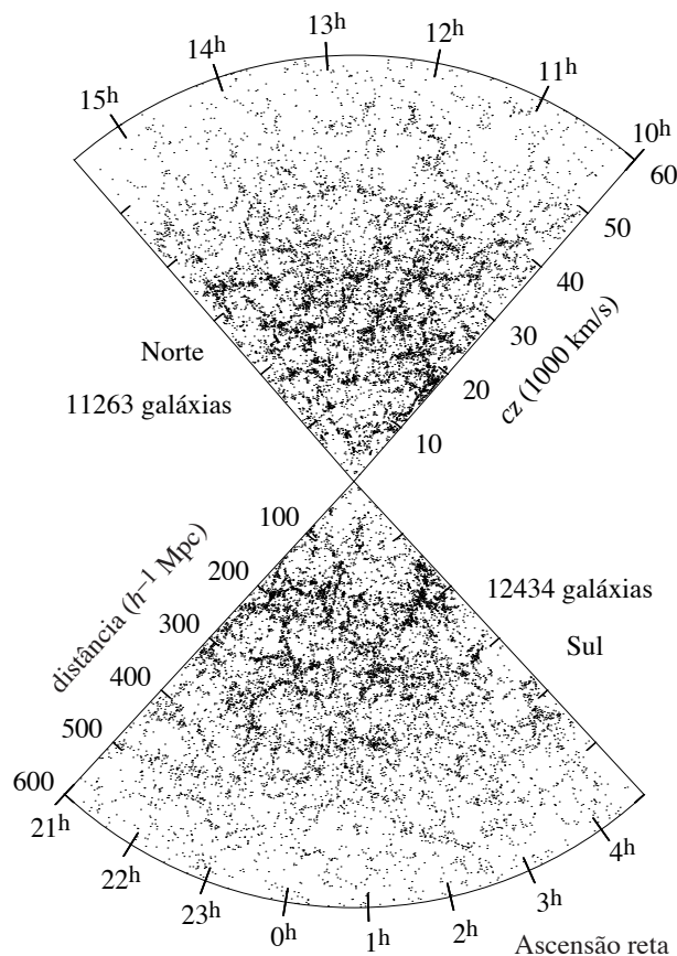
Figura 93: Survey de Las Campanas (Schechter et al., 1996). A parte Norte compreende as declinações -3^\circ \leq \delta \leq -12^\circ ; no Sul os limites são -39^\circ \leq \delta \leq -45^\circ . A aparente diminuição do número de galáxias para velocidades maiores do que \sim 45 \times 10^3 \text{ km s}^{-1} ( z \gtrsim 0,15 ) é devido à incompletude da amostra; apenas as galáxias mais brilhantes (e mais raras) são observadas a grandes distâncias (veja seção 4.6).
