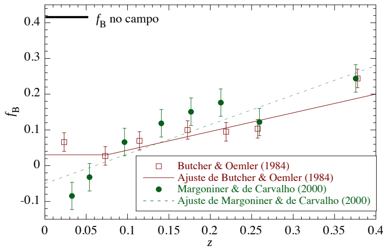
Figura 145: Fração de galáxias azuis em função do redshift . O traço contínuo se refere ao trabalho original de Butcher & Oemler (1984) , a linha tracejada é um trabalho mais recente de Margoniner & de Carvalho (2000) . O traço espesso no alto à esquerda dá a fração de galáxias azuis no campo.
