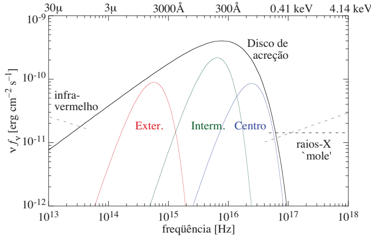
Figura 230: Espectro térmico de um disco de acreção. Este espectro pode ser interpretado pela soma de corpos negros de diferentes regiões do disco (Malkan, 1983).
