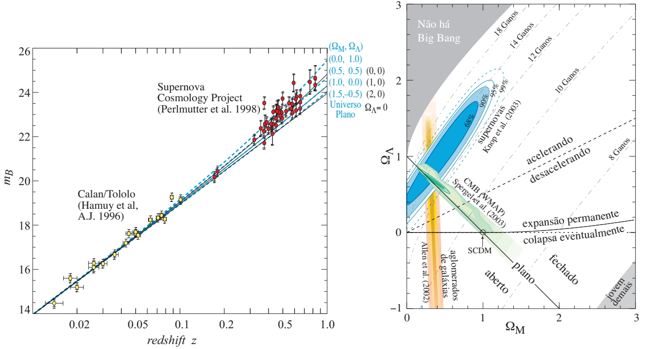
Figura 46: Diagrama de Hubble utilizando uma amostragem de Supernovas de tipo Ia e determinação dos parâmetros cosmológicos. Do diagrama a direita temos também a idade do Universo hoje (usando h = 0,7 ) em função dos parâmetros cosmológicos.
