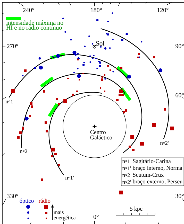
Figura 9: Mapa da Galáxia de Yvonne e Yvon Georgelin, baseado em medidas de distância de regiões HII observadas em rádio e no óptico. Aqui aparecem os quatro principais braços da Via Láctea. Baseado na figura original de Georgelin & Georgelin (1976) .
