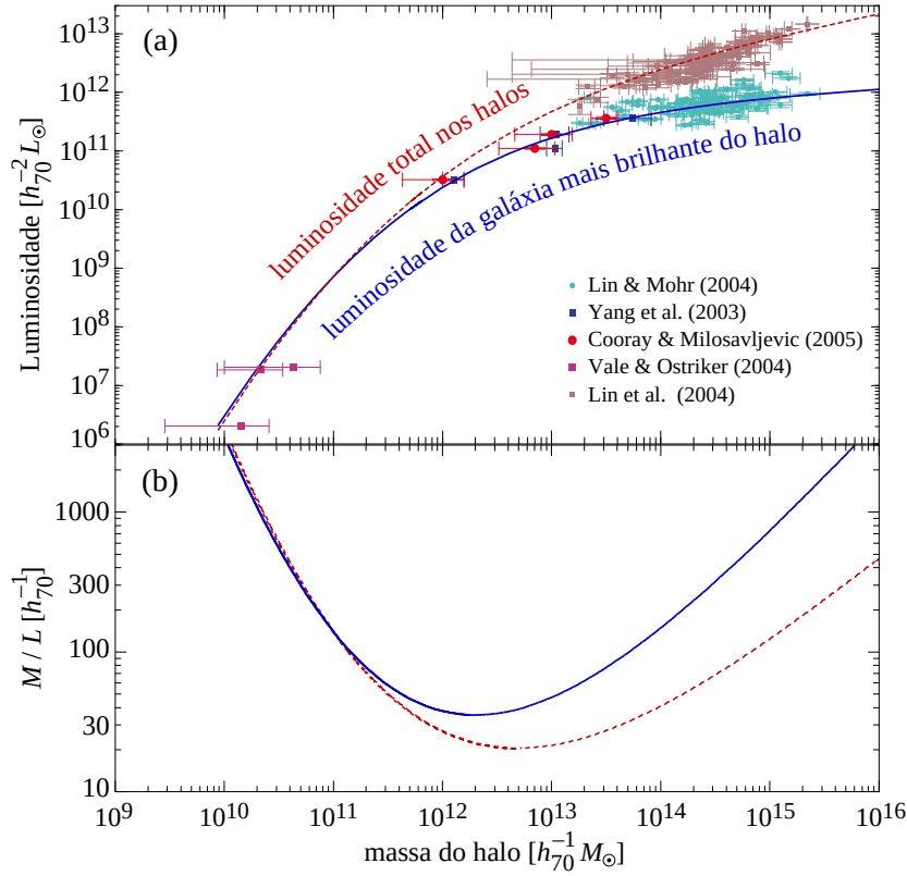
Figura 189: Acima: Luminosidade da galáxia mais brilhante (linha cheia azul) ou de todas as galáxias (linha tracejada vermelha) em função da massa total do halo que contem estes objetos. Abaixo: as razões massa-luminosidade correspondentes às funções do painel acima. As luminosidades aqui correspondem à banda no infravermelho próximo, K . Figura baseada em Cooray & Milosavljevič (2005).
