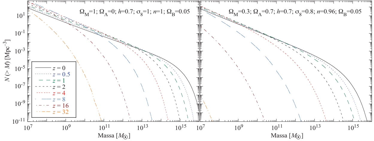
Figura 178: Distribuição integrada de massas de halos colapsados para diferentes redshifts . Esquerda: SCDM. Direita: LambdaCDM.
