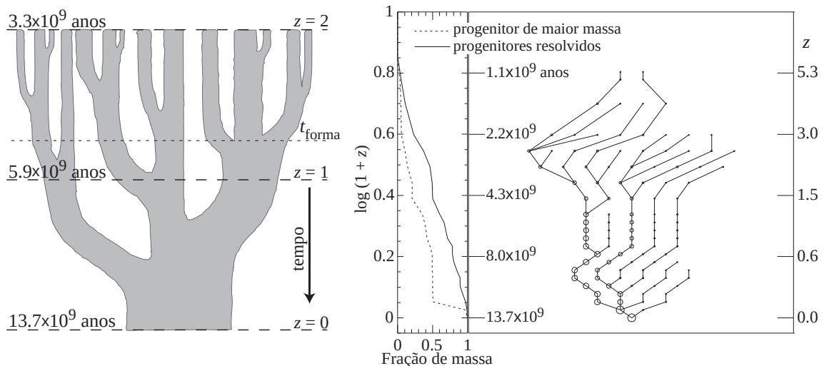
Figura 80: Esquerda: representação gráfica de uma “árvore de fusões” onde a largura dos “galhos” é proporcional à massa do objeto. Cortes horizontais mostram os progenitores que darão origem ao objeto final (uma galáxia, grupo ou aglomerado). A linha t_{\text{forma}} indica o momento de formação do objeto final, definido pelo momento em que sua massa é superior à metade da massa final. Direita: Outra representação de uma árvore de fusões tiradas de uma simulação numérica da formação de uma halo de matéria escura de \sim 10^{13} M_{\odot} . Figura tirada de Lacey & Cole (1993) e Helly et al. (2003).
