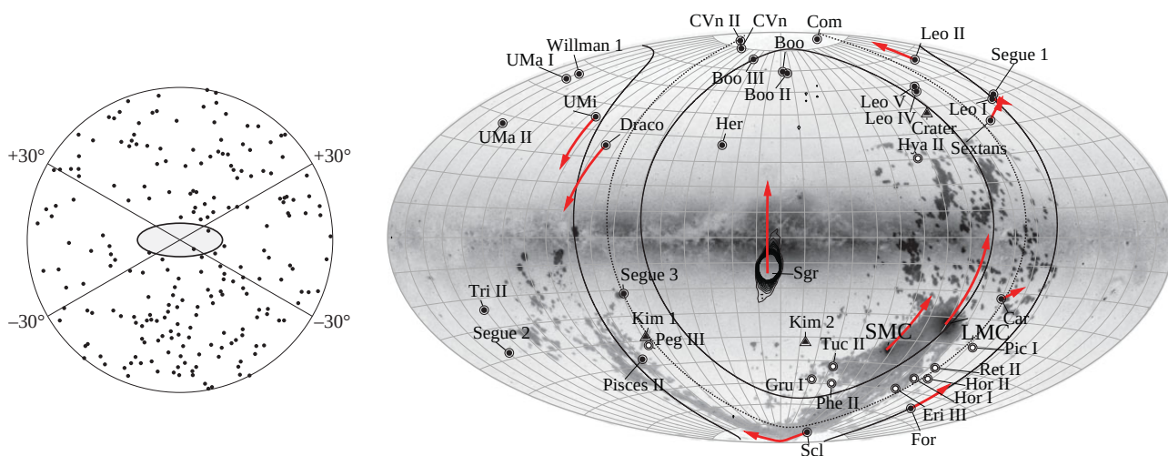
Figura 167: Esquerda: Distribuição de 218 galáxias vizinhas de espirais gigantes vistas de perfil segundo Holmberg (1969) . As galáxias satélites tendem a se concentrarem ao longo do eixo menor. Direita: Distribuição das galáxias satélites da Via Láctea na esfera celeste em coordenadas galácticas. As curvas espessas indicam o grande círculo onde as galáxias satélites se concentram. Os vetores (em vermelho) indicam o movimento projetado no plano do céu de algumas galáxias. Figura tirada de Pawlowski et al. (2015) .
