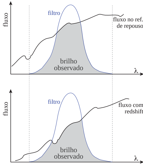
Figura 32: Correção K. O brilho observado é a convolução entre o fluxo emitido pela fonte (mais precisamente a distribuição espectral de energia, SED) e o perfil do filtro utilizado (além da óptica e eficiência do detector, absorção pelo meio interestelar, etc. . . ). A diferença em magnitude dos brilhos da mesma fonte em movimento e em repouso é a correção K.
