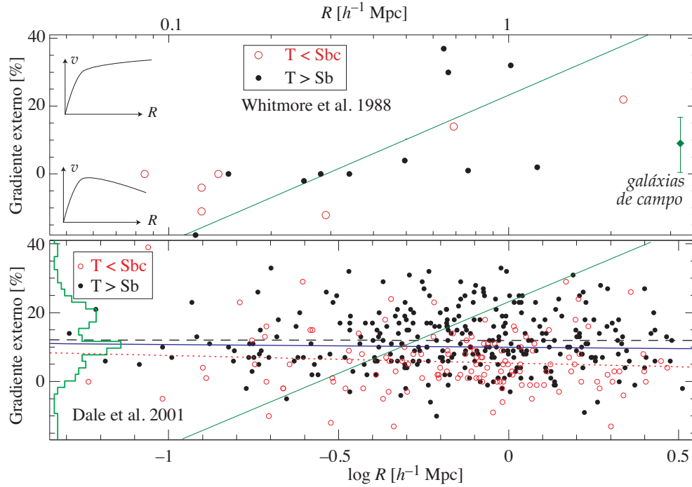
Figura 150: Gradiente externo da curva de rotação de espirais em função da distância ao centro do aglomerado. Acima: amostra de Whitmore et al. (1988) com 19 galáxias em 5 aglomerados. A reta diagonal indica a correlação encontrada por estes autores e o ponto mais a direita dá o valor para galáxias de campo. Abaixo: amostra de Dale et al. (2001) com 438 galáxias em 53 aglomerados de Abell. Os traços pontilhados, tracejados e contínuo são as correlações para espirais de tipo precoce, tipo tardio e todas as galáxias, respectivamente (o traço diagonal é a correlação de Whitmore et al.
