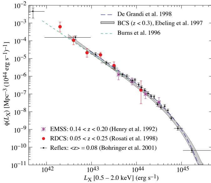
Figura 187: Função de luminosidade de aglomerados selecionados em raios-X (diversos surveys ROSAT e Einstein ) no Universo próximo (supondo Einstein-de Sitter e H_0 = 50 \text{ km s}^{-1} \text{ Mpc}^{-1} ). Figura tirada de Rosati et al. (2002).
