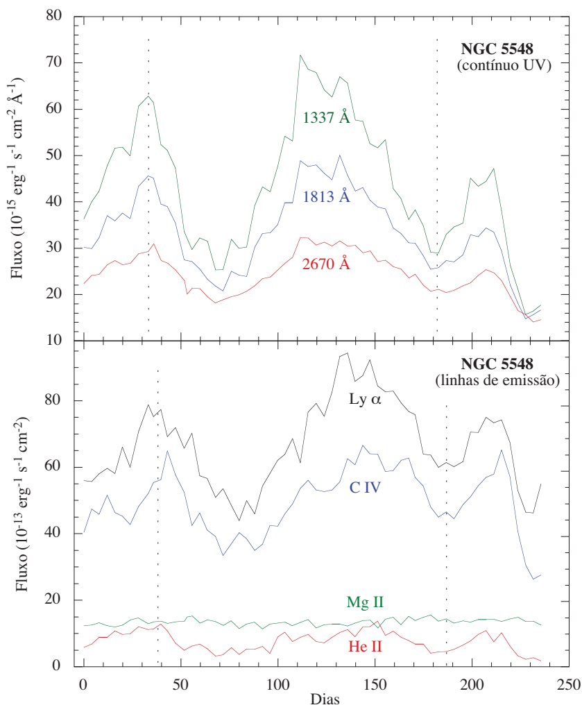
Figura 226: Variação do contínuo UV e de linhas de emissão de NGC 5548 (Seyfert tipo 1). Note que as variações não são simultâneas: isto permite estimarmos as distâncias entre as regiões que produzem as diferentes linhas/contínuos.
