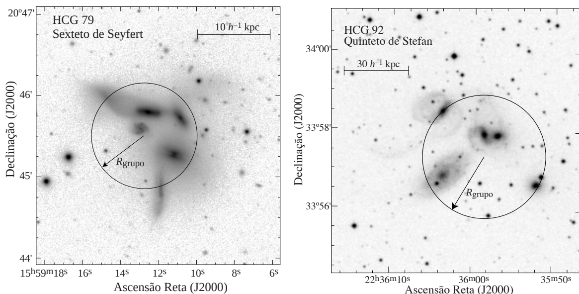
Figura 155: Dois aglomerados do catálogo de Hickson. R_{\text{grupo}} satisfaz o critério de seleção e define o raio do grupo. As imagens são do SDSS (filtro r ) e do DSS (filtro vermelho) para HCG 79 e HCG 92, respectivamente.
