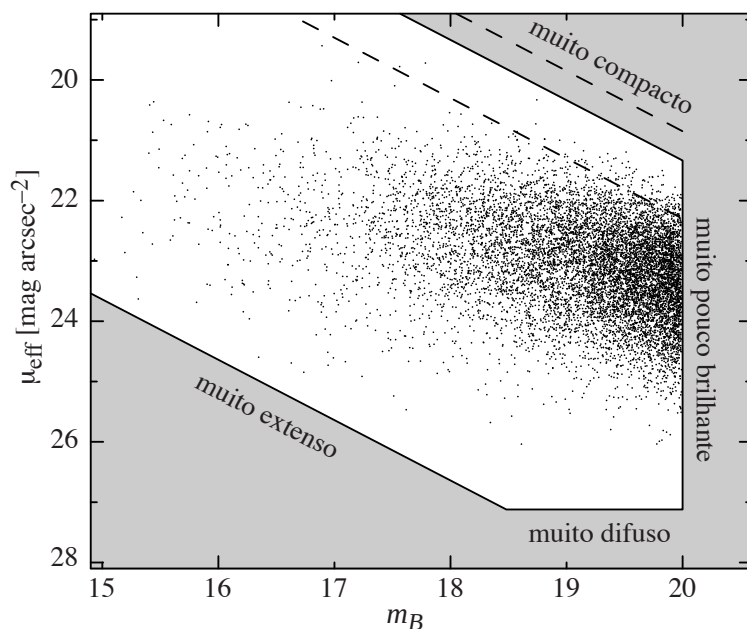
Figura 111: Efeitos de seleção na contagem de galáxias. As linhas tracejadas diagonais superiores indicam o efeito do “seeing” na detecção de objetos compactos. Figura tirada de Liske et al. (2002) .
