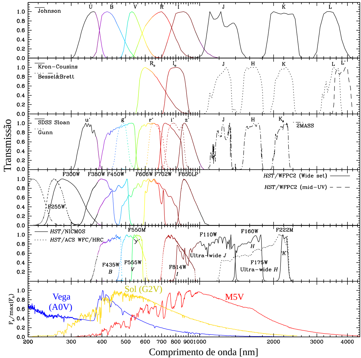
Figura 263: Perfis de transmissão de algumas das bandas fotométricas mais utilizadas
