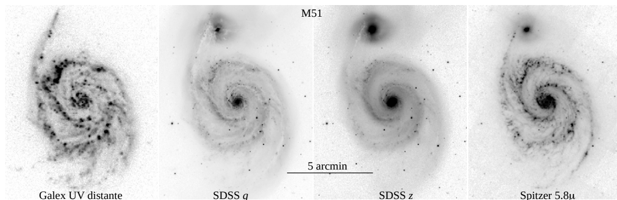
Figura 253: “Correção K morfológica”. Galáxia M51 observada em diferentes comprimentos de onda, do ultravioleta (0,135–0,175 \mu ) ao infravermelho 5,8 \mu .
