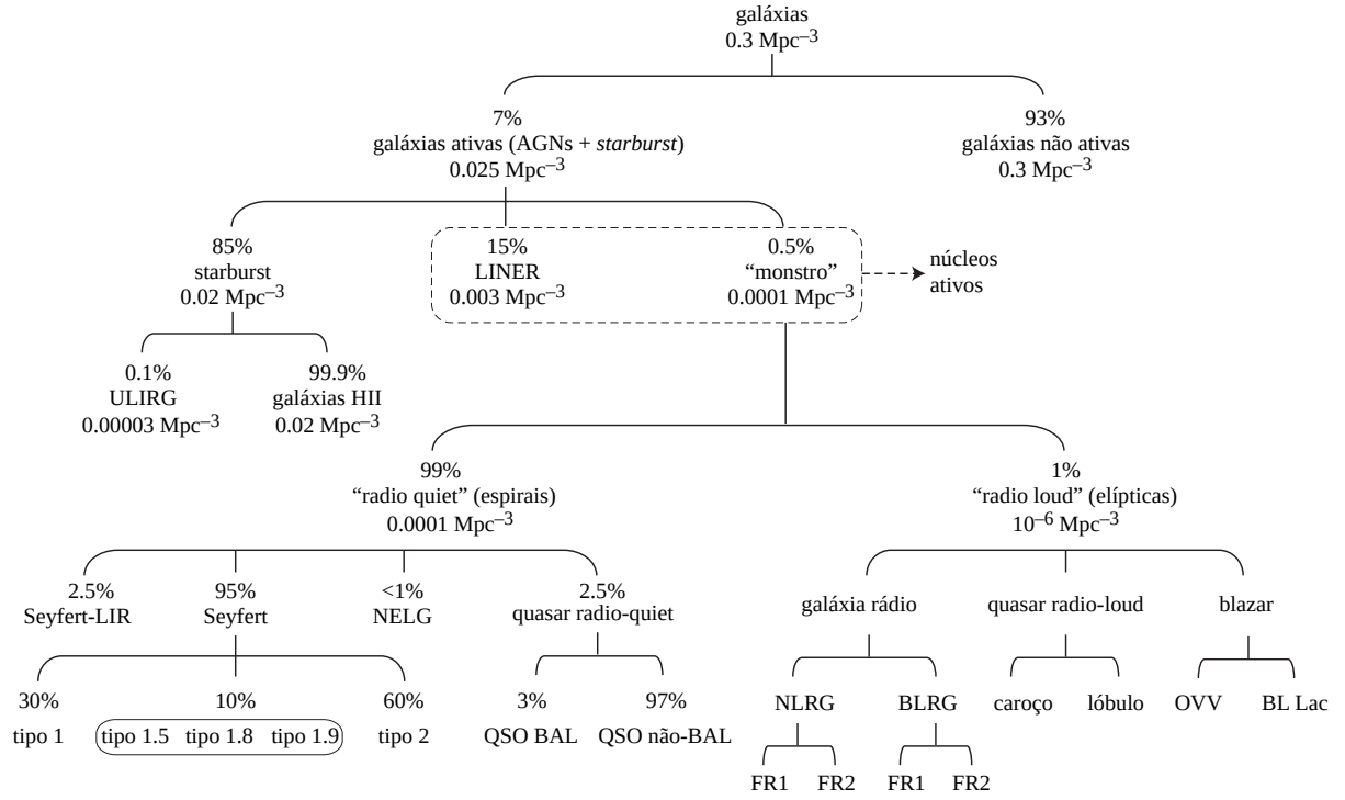
Figura 210: Demografia de galáxias com atividade (AGNs e formação estelar intensa). As porcentagens e densidades são aproximadas. “LIR” significa luminoso no infravermelho; “BAL” linha de absorção larga; “FR” Fanaroff-Riley (veja seção 11.5.2); “NELG” galáxia com linha de emissão estreita. Tirado de Roy (1994).
