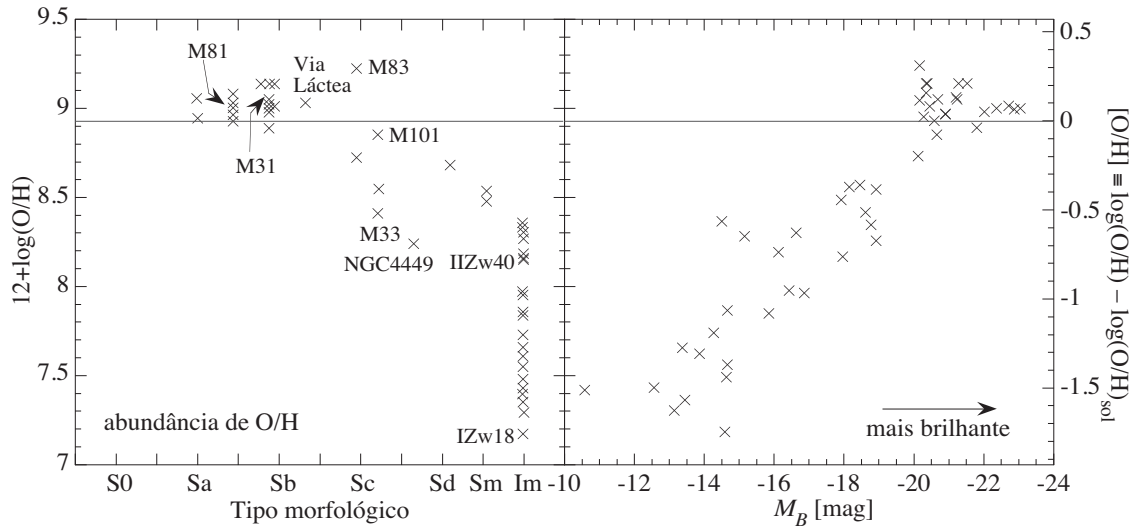
Figura 246: Abundância de oxigênio em função do tipo morfológico (espirais e irregulares) e da massa das galáxias. A abundância solar de oxigênio é 12 + \log(\text{O}/\text{H}) = 8,91 e a metalicidade pode ser calculada como Z/Z_{\odot} = 10^{\log(\text{O}/\text{H}) - 3,09} . Figura baseada em Roberts & Haynes (1994) .
