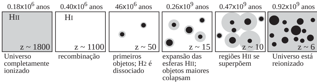
Figura 236: Reionização do Universo após a recombinação. Cinza escuro representa o hidrogênio ionizado. Círculos pretos são objetos colapsados. A escala de tempo é baseada no cenário \Lambda CDM com h = 0,7 . Figura baseada em Barkana & Loeb (2001) .
