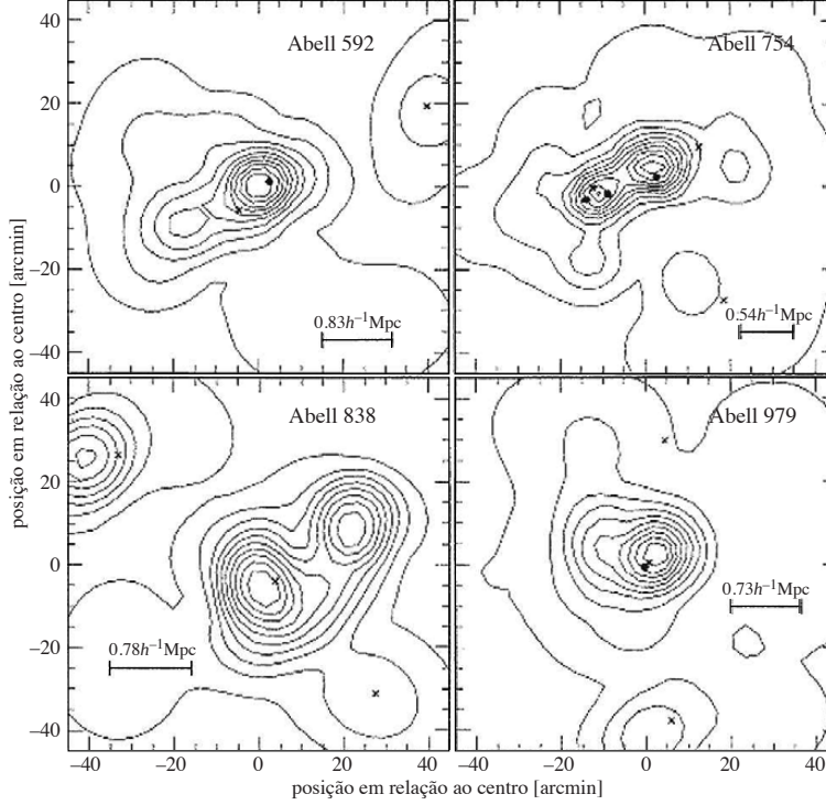
Figura 117: Isocontornos da densidade numérica projetada de galáxias em alguns aglomerados (isopletas), utilizando a técnica “kernel adaptativo”. Círculos cheios correspondem a galáxias D ou cD. Figura tirada de Kriessler & Beers (1997) .
