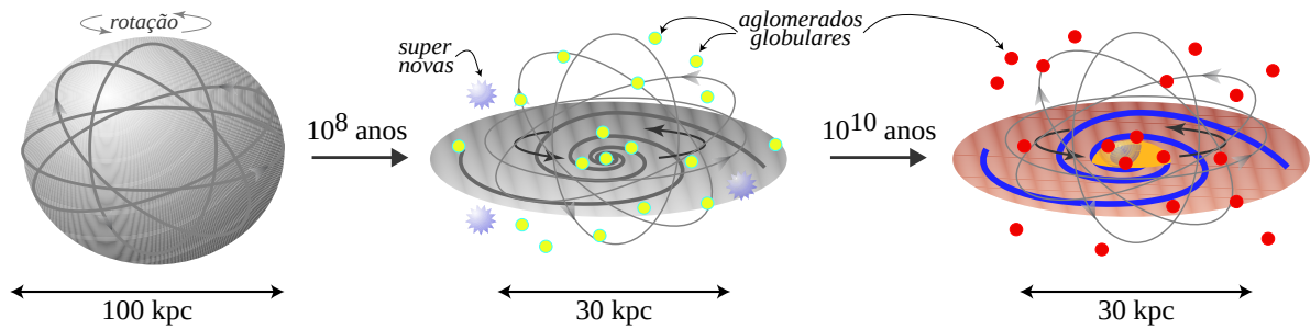
Figura 180: Cenário monolítico para formação de galáxias. Uma nuvem de gás (e matéria escura) em rotação colapsa em queda livre. Durante a queda, há fragmentação e formação de aglomerados globulares e algumas estrelas. O meio é pouco enriquecido devido à rápida escala de tempo de colapso. O gás que não forma estrelas dissipa energia ao colapsar e se assenta em um disco em rotação; neste disco há formação gradual de estrelas, mantendo a cor “azulada” e enriquecendo o meio.
