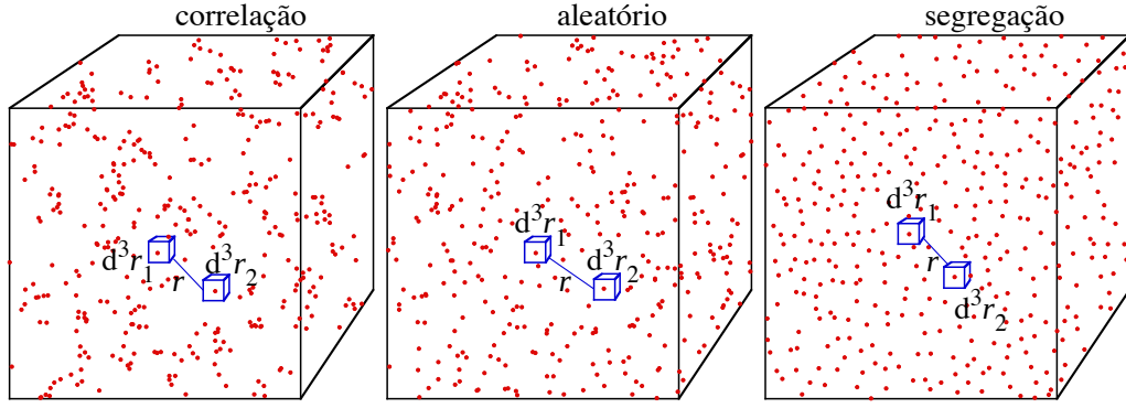
Figura 96: Esquerda: Distribuição onde as partículas se encontram preferencialmente agrupadas (função de correlação positiva); Centro: Distribuição aleatória (Poisson); Direita: Distribuição anti-correlacionado, onde as partículas estão preferencialmente distantes uma das outras, como na superfície de bolhas ou em uma rede cristalina.
