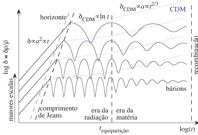
Figura 68: Evolução do contraste de densidade ao entrar no horizonte e se tornar menor que o comprimento de Jeans. A partir deste momento, a perturbação passa a oscilar até o momento da equipartição entre matéria e energia (ver seção 2.5.2). A partir daí, as perturbações de matéria não bariônica fria crescem enquanto que a oscilação das perturbações dos bárions é amortecida ( Silk damping , veja seção 2.5.3). Note que as pequenas escalas entram primeiro no horizonte e oscilam com maior frequência. As curvas estão deslocadas verticalmente para maior clareza.
