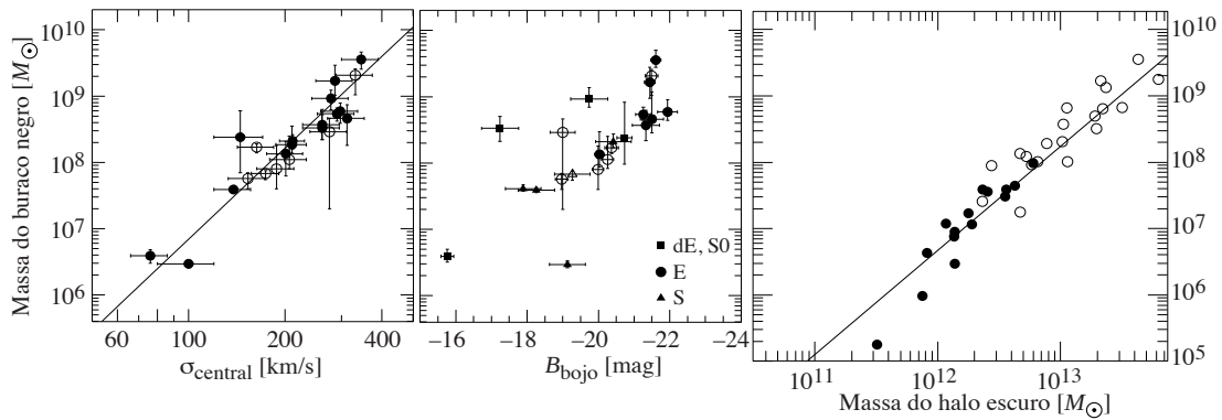
Figura 235: Correlações da massa do BN com a dispersão central de velocidades, luminosidade na banda B e massa do halo escuro da galáxia hospedeira. Os símbolos cheios e vazios são dados publicados e não publicados, respectivamente. A massa do halo escuro é estimada pela velocidade circular e/ou \sigma da galáxia hospedeira. Figura adaptada de Ferrarese (2002) .
