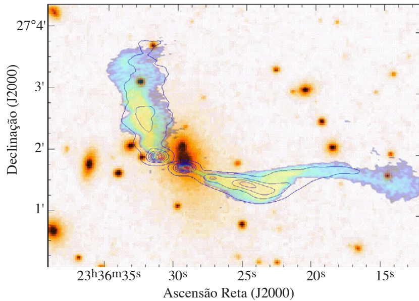
Figura 119: Emissão rádio de tipo “head-tail” 3C465 associada à galáxia elíptica NGC 7720 no aglomerado Abell 2634. A emissão rádio (em tons azuis e com curvas de nível) adquire esta forma devido ao movimento da galáxia em relação ao meio intra-aglomerado. NGC 7720 tem uma velocidade de \sim 200 \text{ km/s} em relação à velocidade média do aglomerado.
