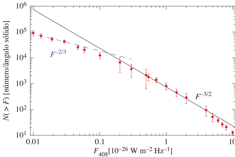
Figura 34: Número de fontes rádio por unidade de ângulo sólido com densidade de fluxo superior a F (Pooley & Ryle, 1968).
