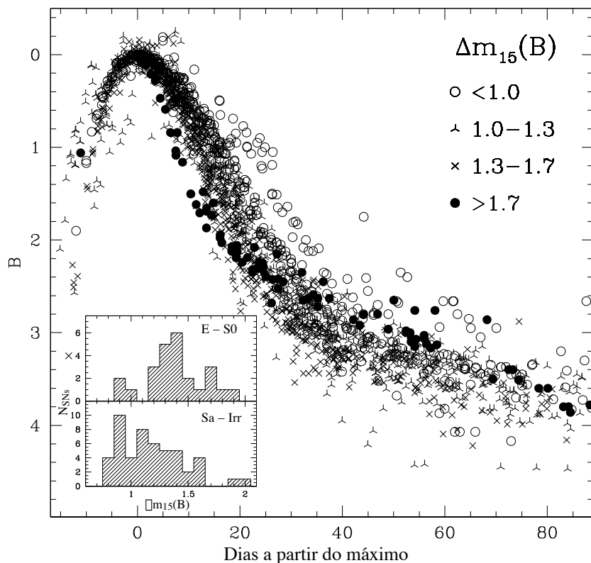
Figura 259: Curva de luminosidade de SNs tipo Ia em relação à fase e à magnitude máxima. Os diferentes símbolos correspondem à diferentes \Delta_{15} , o declínio da luminosidade nos primeiros 15 dias (Cappellaro & Turatto, 2000). No detalhe, os histogramas de \Delta m_{15} separados em early e late-type : a diferença das distribuições é estatisticamente significativa.
