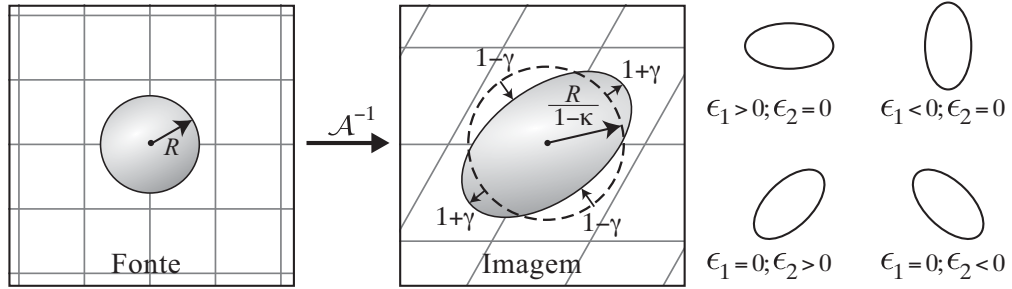
Figura 135: Efeito de lente gravitacional fraca: uma fonte esférica (esquerda) de raio R tem sua imagem deformada (centro), tornando-se uma elipse. O círculo tracejado representa o efeito de convergência. Direita: Representação gráfica da elipticidade complexa, \epsilon_i . Figura baseada em Kneib & Natarajan (2011).
