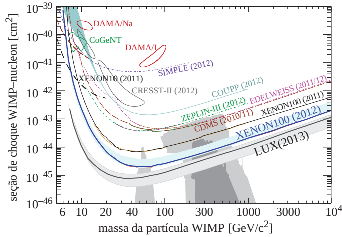
Figura 71: Limite superior (90% de confiança) de detecção da seção de choque de partículas de matéria escura de tipo WIMP para diversos experimentos. As áreas cinzas representam previsões teóricas para a seção de choque em modelos de supersimetria ( constrained minimal supersymmetric Standard Model , cMSSM). Figura adaptada de Aprile et al. XENON100 Collaboration (2013) ; Akerib et al. LUX Collaboration (2013) .
