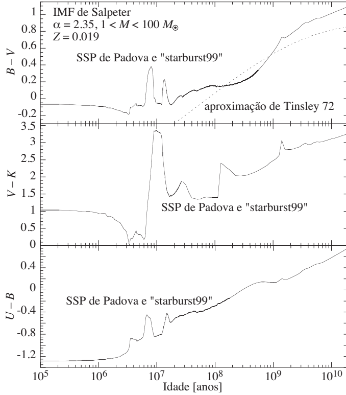
Figura 201: Evolução do índice de cor para um surto de formação estelar em t = 0 . Dados de Leiteher et al. 1999 (código “starburst”) e do grupo de Padova (Salasnich et al., 2000).
