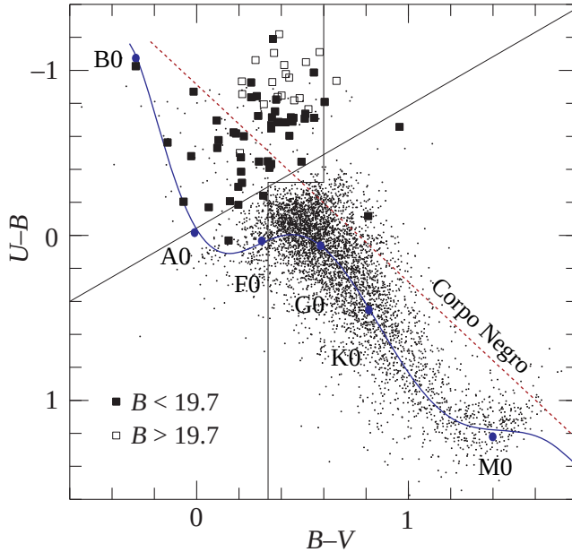
Figura 219: Diagrama cor-cor U-B vs. B-V , ilustrando como os Quasares podem ser identificados. A reta diagonal representa a relação (U-B) = -0,75(B-V) - 0,05 . Os símbolos quadrados (vazios e cheios) representam os Quasares, o pontos são estrelas. Para comparação, superpomos a posição neste diagrama das estrelas da sequência principal e a reta correspondente a um corpo negro. Figura baseada em Scholz et al. (1997).
