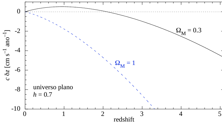
Figura 29: Variação do redshift de uma fonte comóvel (em termos de velocidade) em função do redshift cosmológico correspondente ao intervalo de um ano.
