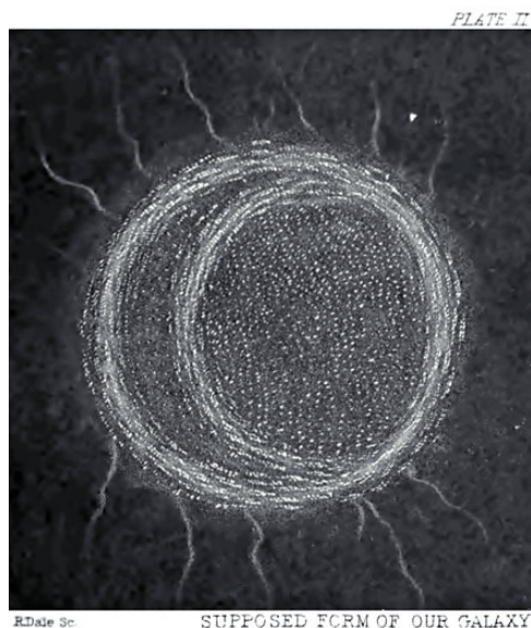
Figura 6: Modelo da Via Láctea de Nichol (1848) (de onde foi tirada esta figura) na forma de um anel (um modelo semelhante já havia sido proposto por Nichol em 1839). Nichols acrescenta uma subestrutura a um simples anel devido a não homogeneidade observada ao longo da Via Láctea (o que poderia ser considerada a primeira evidência da presença de braços espirais na Galáxia). O Sol se encontra próximo mas não exatamente no centro do sistema. Este modelo foi influenciado pela observação de M51 por John Herschel [veja Fig. 3, painel (a)].
