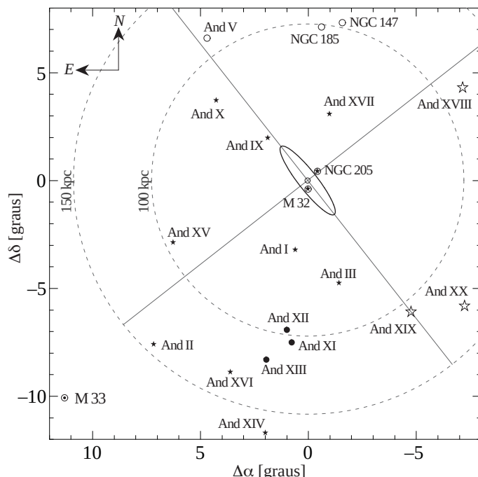
Figura 160: Distribuição das galáxias do sub-grupo de M31. A elipse central representa o disco de M31, inclinada na linha de visada de 77^\circ e com raio de 2^\circ (27 kpc). Figura adaptada de McConnachie et al. (2008) .
