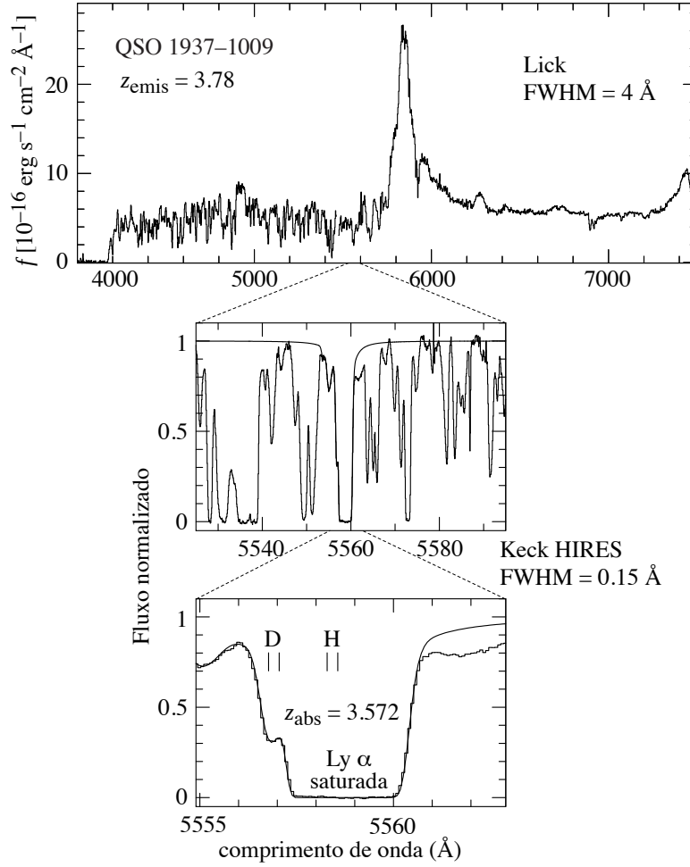
Figura 56: Detecção do deutério em um QSO de alto redshift . Figura tirada de Burles & Tytler (1998) .
