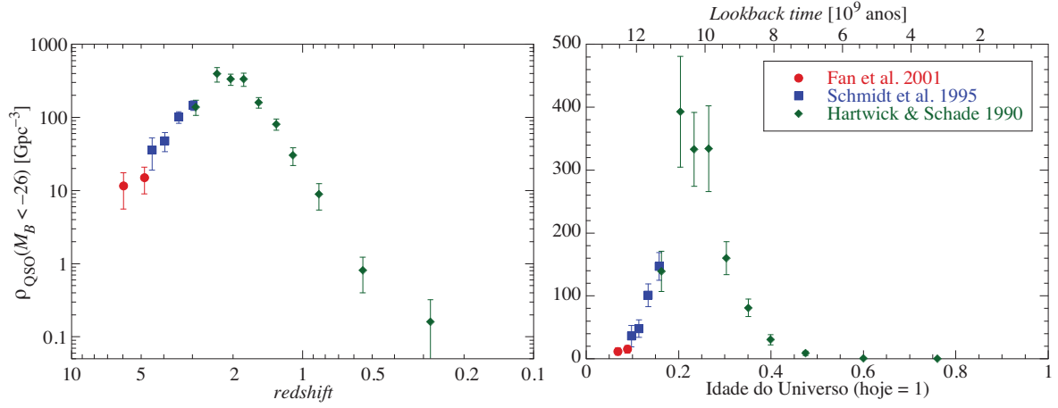
Figura 220: Abundância (densidade em coordenadas comóveis) de QSOs em função da idade do Universo e do redshift para QSOs com M_B < -26 . Para z \gtrsim 6 não sabemos ainda como evolui esta abundância. A maior abundância de QSOs ocorre cerca de 3 bilhões de anos após o Big Bang, quando a densidade comóvel é de \sim 350 \text{ Gpc}^{-3} . Dados tirados de Fan et al. (2001); Schmidt et al. (1995); Hartwick & Schade (1990).
