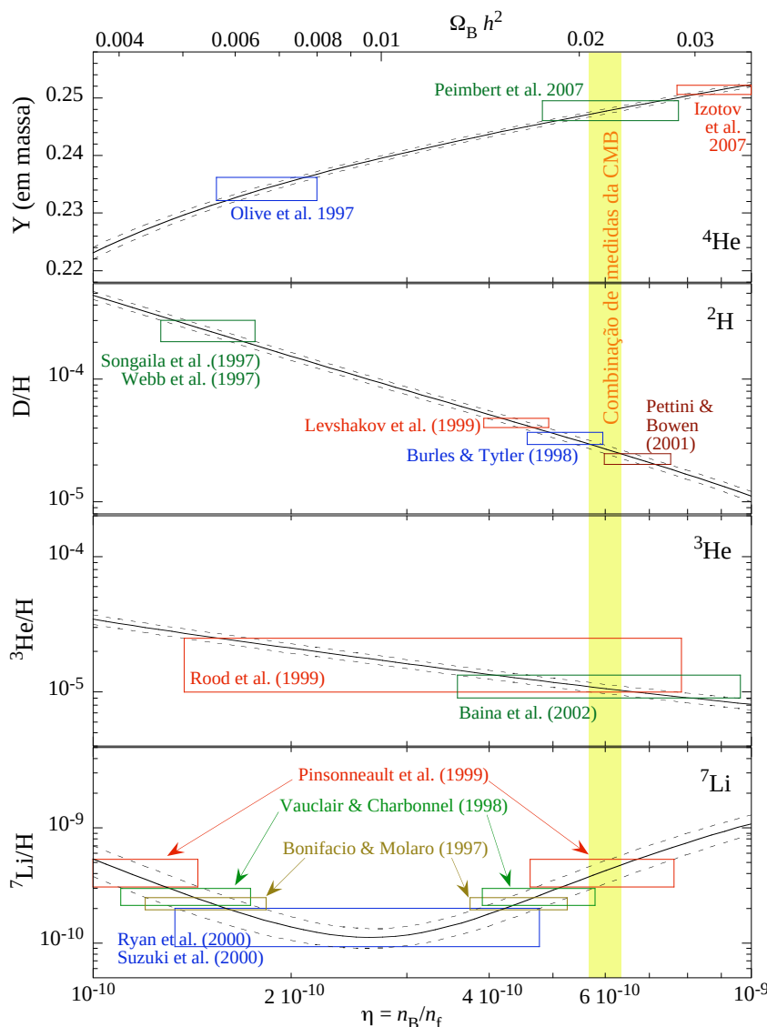
Figura 55: Abundância dos elementos devido à nucleossíntese primordial em função da densidade de bárions no Universo (expresso pelo fator \eta ou \Omega_B h^2 ). O deutério é o elemento cuja abundância depende mais sensivelmente de \eta . Para \Omega_B h^2 \rightarrow 1 , a abundância de D é virtualmente zero. As linhas tracejadas indicam a incerteza do modelo na abundância de cada elemento. As observações atuais se encontram nos retângulos para cada elemento. O retângulo vertical dá a estimativa combinada das medidas dos detectores WMAP, ACBAR e CBI utilizando a CMB, \Omega_B h^2 = 0,0224 \pm 0,0010 .
