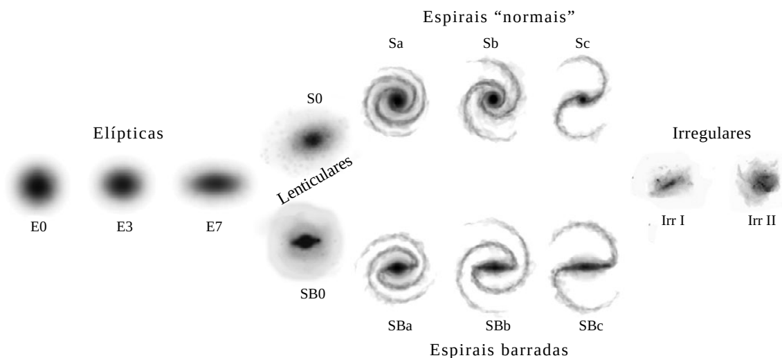
Figura 244: Classificação morfológica de Hubble ( ‘tunefork’ ou diapasão).
