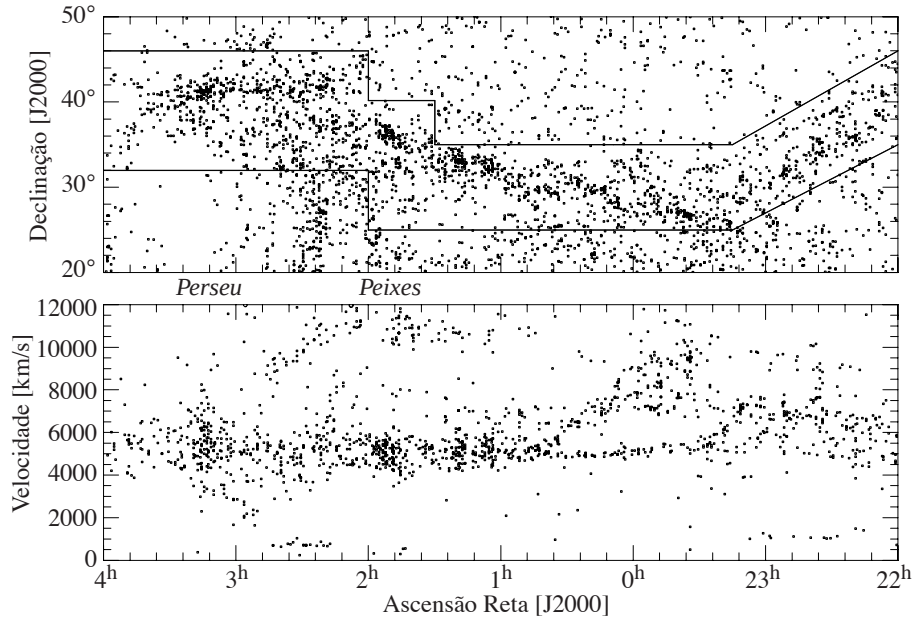
Figura 92: Filamento de galáxias na região Perseu–Peixes, projetado no plano do céu (acima) e no espaço de velocidades (abaixo). Survey realizado por Wegner et al. (1993).
