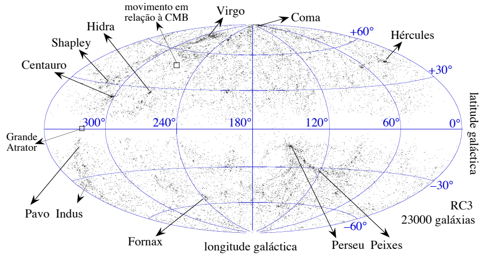
Figura 88: Distribuição em toda a esfera celeste (em coordenada galácticas) das galáxias mais brilhantes que m_B = 15,5 [catálogo RC3, de Vaucouleurs et al. (1991)]. Note a “zona de exclusão” (avoidance zone) relacionada ao obscurecimento devido à poeira da Via Láctea no plano equatorial deste gráfico.
