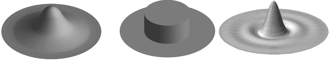
Figura 175: Exemplo de filtros em 2 dimensões. Esquerda: gaussiano; Meio: ‘top-hat’ (cartola); Direita: transformada de Fourier do filtro top-hat..
