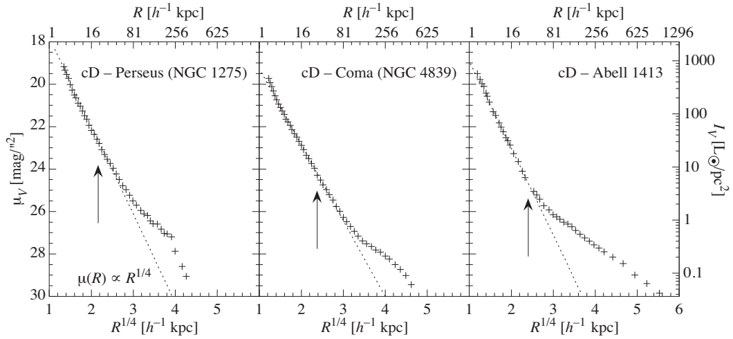
Figura 140: Perfil de brilho superficial da galáxia cD de Abell 1413, do aglomerado de Perseus e de Coma. A reta pontilhada corresponde ao perfil de de Vaucouleurs, típico de elípticas. A flecha vertical indica o raio efetivo. Perfis tirados de Schombert (1986)
