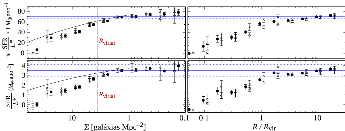
Figura 149: Acima: fração de galáxias com taxa de formação estelar (SFR) normalizada por unidade de L^* ( L^* \approx 10^{10} L_\odot , seção 9.2.2) acima de 1 M_\odot/\text{ano} . Abaixo: SFR mediana (normalizada por L^* ). À esquerda, grandezas em função da densidade local de galáxias; à direita em função do raio do virial (veja seção 8.1). Nos painéis da esquerda, a curva representa o decréscimo da SFR esperado baseando-se na segregação morfológica. Figura adaptada de Lewis et al. (2002).
