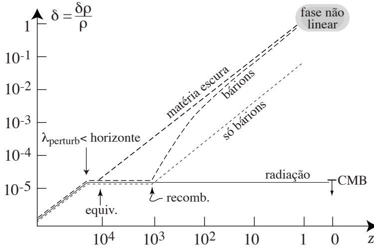
Figura 72: Evolução do contraste de densidade em um cenário CDM de uma região com 10^{14} M_{\odot} . Em um Universo puramente bariônico, não há tempo para que estruturas em colapso atinjam a fase não linear em z \leq 1 . Figura tirada de (Combes et al., 2006) . A evolução de \delta\rho/\bar{\rho} no momento em que a perturbação entra no horizonte pode ser vista na Fig. 68.
