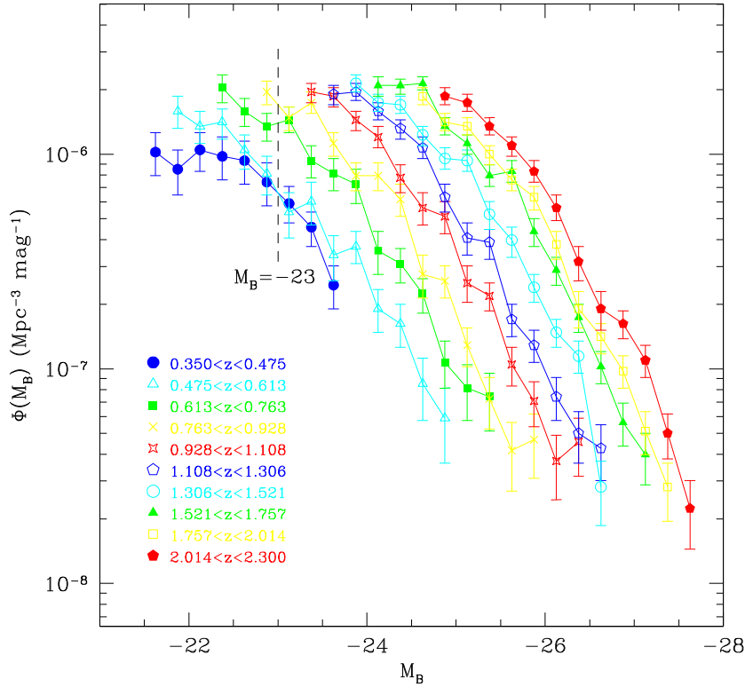
Figura 221: Função de luminosidade de QSOs por intervalo de redshift a partir dos catálogos 2QZ e LBQS (supondo um Universo plano, q_0 = 0.5 e h_{100} = 1/2 ). Figura tirada de Boyle et al. (2000).
