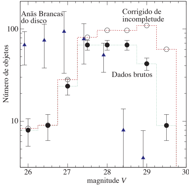
Figura 43: Função de luminosidade de anãs brancas no aglomerado M5 (círculos) e no disco da Via Láctea (triângulos). A queda da FL para objetos fracos é um indicador de idade. O corte em magnitudes menos elevadas do disco mostra que este é mais jovem que M5. Figura tirada de Hansen et al. (2002).
