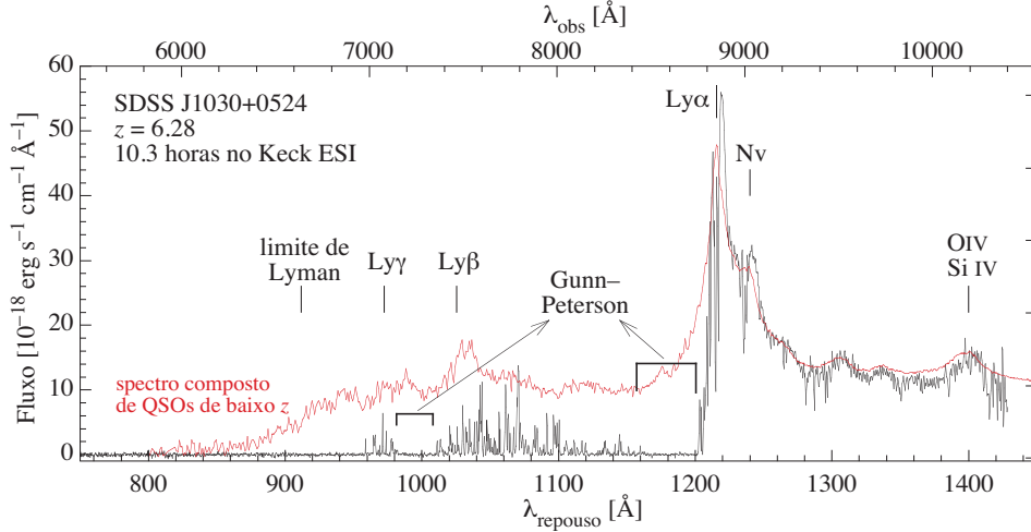
Figura 237: Efeito Gunn-Peterson observado em um QSO de alto redshift , do lado azul das linhas Ly- \alpha e Ly- \beta . Onde o efeito G-P não ocorre, observamos a “floresta de Lyman”. Para efeito de comparação, o espectro composto de QSOs de baixo redshift está superposto ao QSO de alto redshift . Figura baseada em White et al. (2003).
