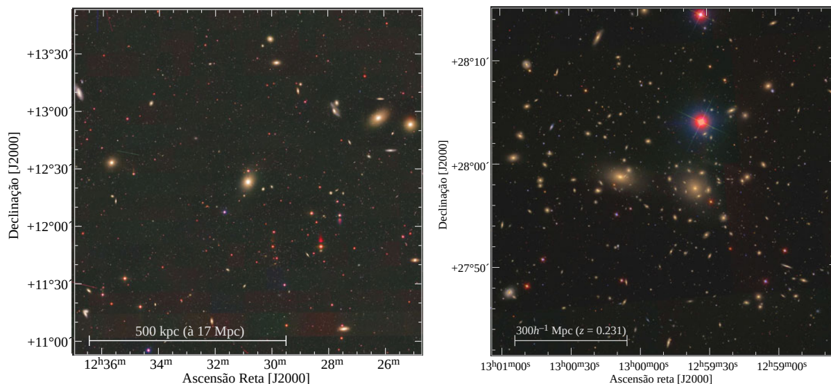
Figura 112: Esquerda: Região central do Aglomerado de Virgo. Direita: Aglomerado de Coma. Ambas as imagens são em cores verdadeiras do SDSS.
