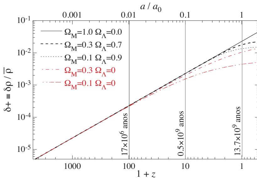
Figura 69: Crescimento de perturbações de densidade no regime linear. \delta_+ indica a solução da equação (146) que aumenta com o tempo (existe também uma solução de decréscimo). A idade do Universo (linhas verticais) é calculada para um modelo \Omega_\Lambda = 0,7 , \Omega_M = 0,3 e H_0 = 70 \text{ km s}^{-1} \text{ Mpc}^{-1} . O efeito de H_0 é equivalente à normalização.
