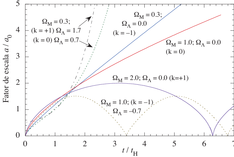
Figura 37: Evolução do fator de escala a/a_0 para universos de Friedmann ( \Omega_\Lambda = 0 , traços contínuos) e com \Omega_\Lambda \neq 0 . Para cada modelo, damos a curvatura: aberto ( k = -1 ), crítico ( k = 0 ) e fechado ( k = 1 ). Neste exemplo, H_0 é a mesma para todos os universos, a/a_0 = 1 corresponde a época atual.
