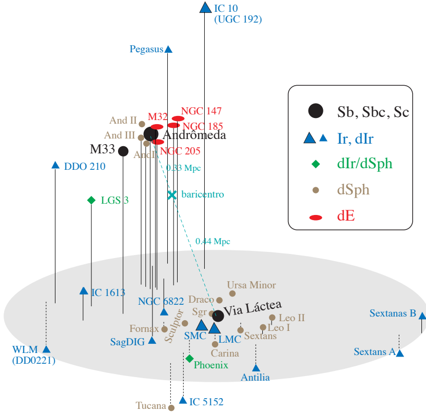
Figura 158: Representação esquemática do Grupo Local (fora de escala). Figura tirada de Grebel (2000) .
