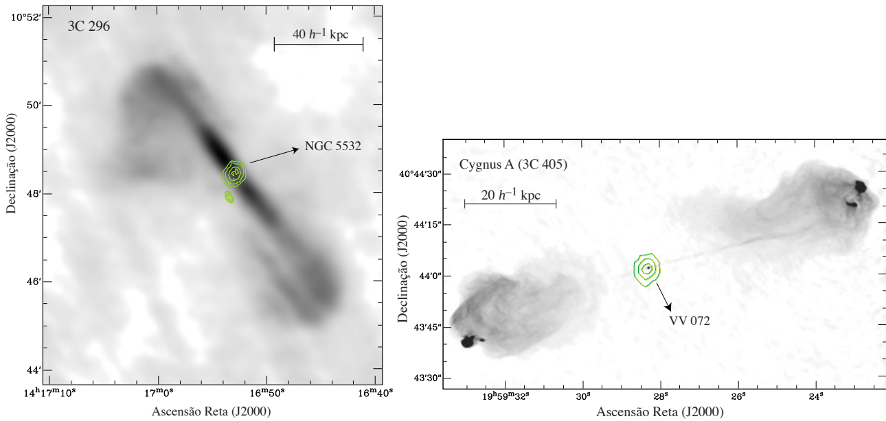
Figura 214: Esquerda: Rádio galáxia tipo FR I. Os contornos centrais correspondem à imagem óptica da galáxia responsável pela emissão rádio. Direita: Rádio galáxia tipo FR II. As imagens são do banco de dados do VLA.
