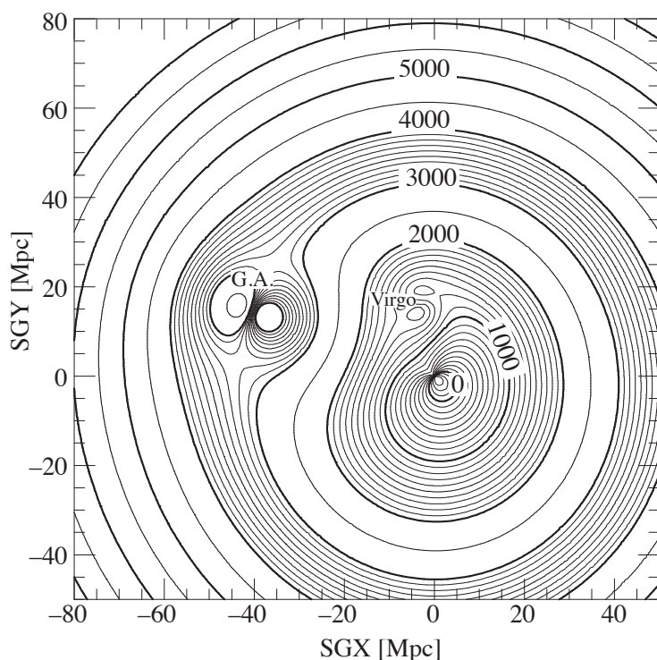
Figura 109: Campo de velocidade no universo local no plano supergaláctico. Podemos ver claramente os efeitos do Grande Atrator e do aglomerado de Virgo. Mais sutil, mas visível, é o efeito do próprio Grupo Local [com coordenadas (0, 0)]. As velocidades são dadas em km/s. Esta determinação foi feita de maneira independente do método POTENT descrito acima. Figura tirada de Tonry et al. (2000).
