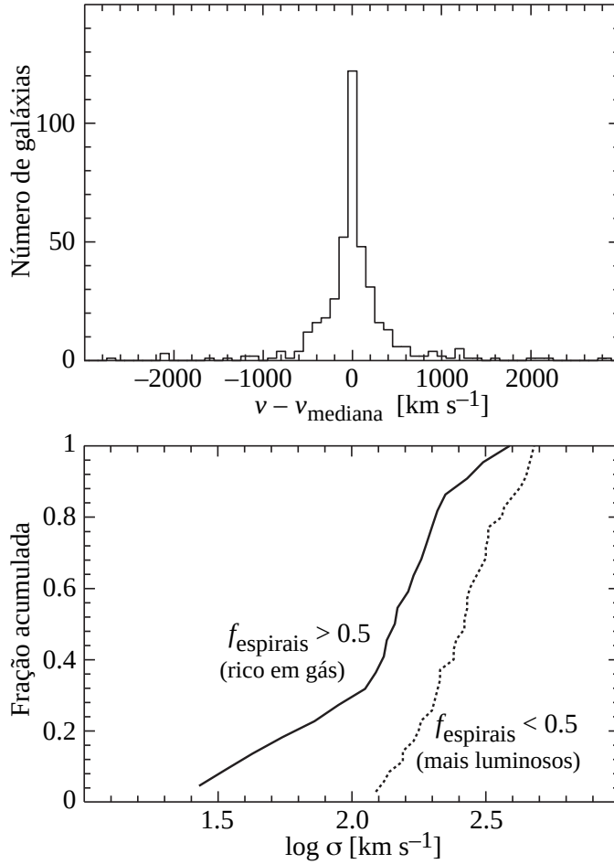
Figura 156: Acima: distribuição de velocidades de 410 galáxias do catálogo de Hickson em relação à mediana dos respectivos grupos. A distribuição pode ser aproximada por uma gaussiana com \sigma \approx 250 \text{ km s}^{-1} (77% das galáxias têm uma diferença de velocidade inferior a 500 \text{ km s}^{-1} ). Abaixo: Relação entre a morfologia e a dispersão de velocidades. A dispersão em grupos pobres em espirais é tipicamente o dobro da dispersão em grupos com f_{\text{espirais}} > 0.5 . Figuras tiradas de Hickson (1997)
