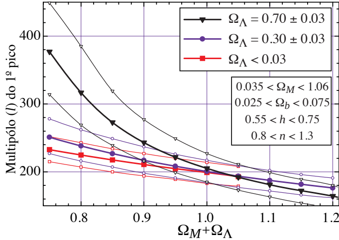
Figura 62: Posição do primeiro pico do espectro de potência angular da CMB em função da curvatura do Universo, para diversos cenários cosmológicos. Os traços espessos correspondem aos valores médios dos modelos e os traços finos dão os limites levando-se em conta todas as incertezas dos parâmetros cosmológicos ( n é a inclinação do espectro de potência inicial, cf. seção 3.4). Figura tirada de Masi et al. (2002).
